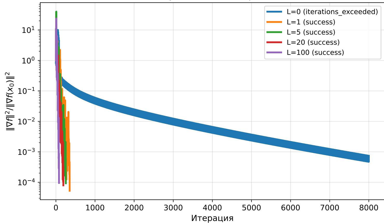
П. 2.3 (в): плохо обусловленная квадратура, n=40 , \kappa=10^4
