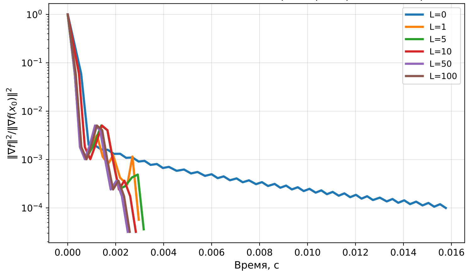
П. 2.3 (б): triazines, относительный квадрат нормы градиента vs время
