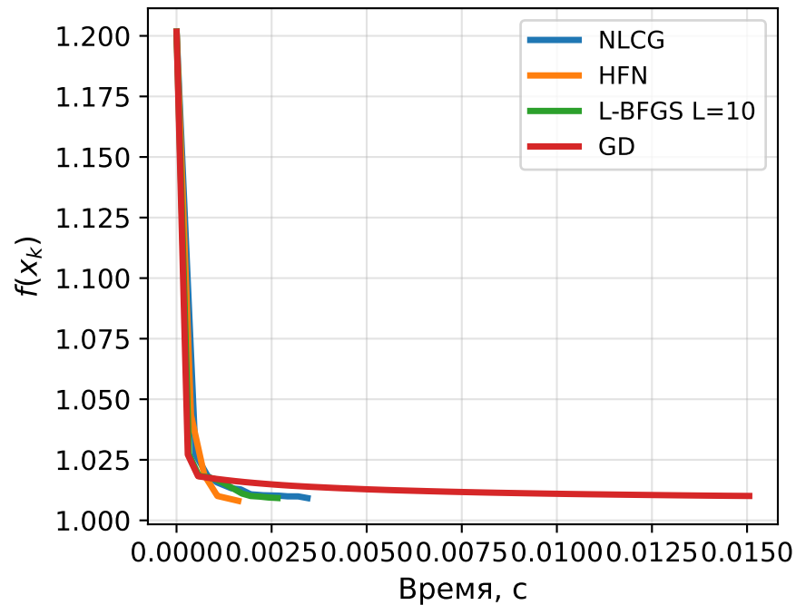
(б) f vs время
