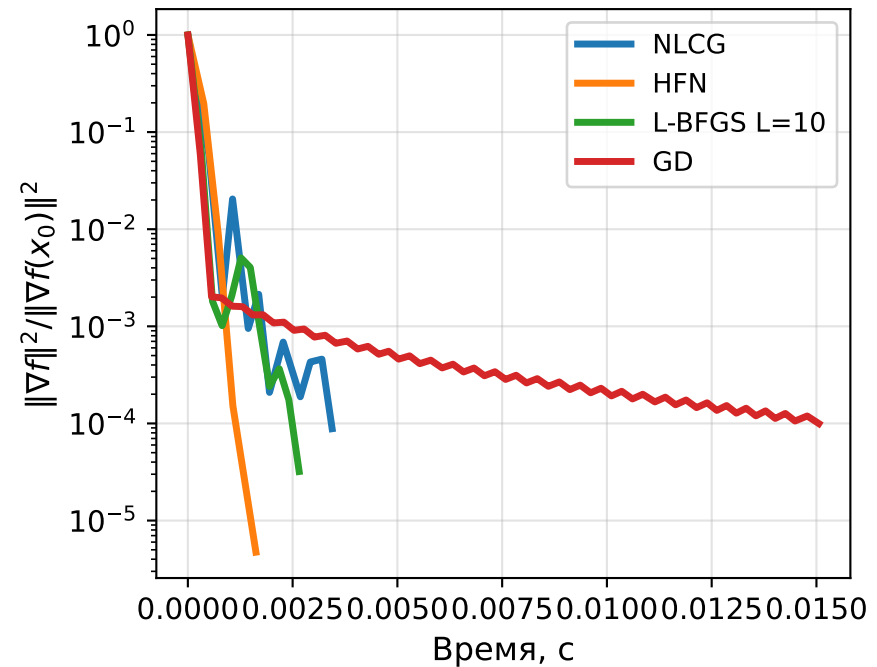
(в) отн. квадрат нормы градиента
