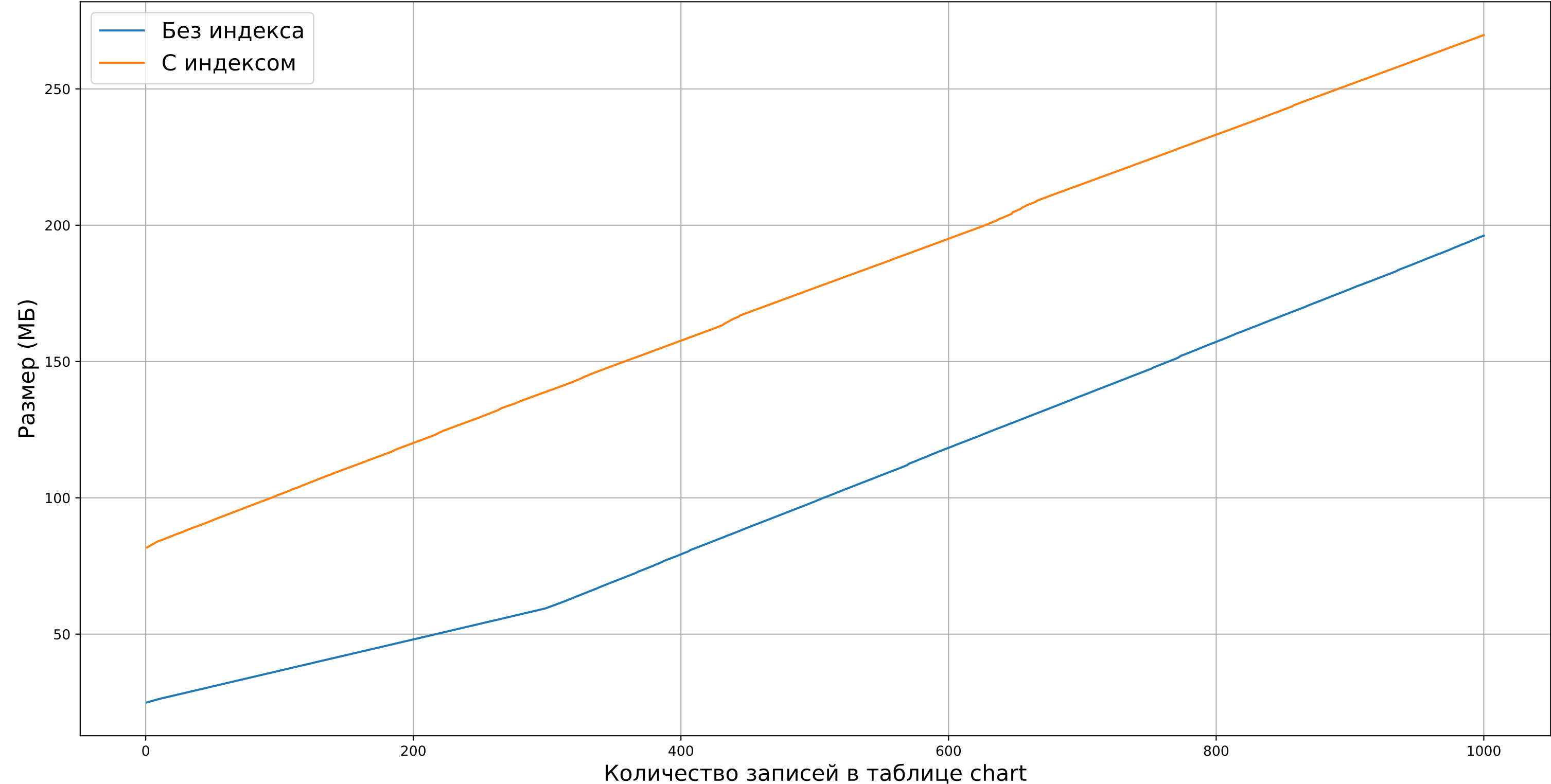
График зависимости объема дискового пространства от количества записей
