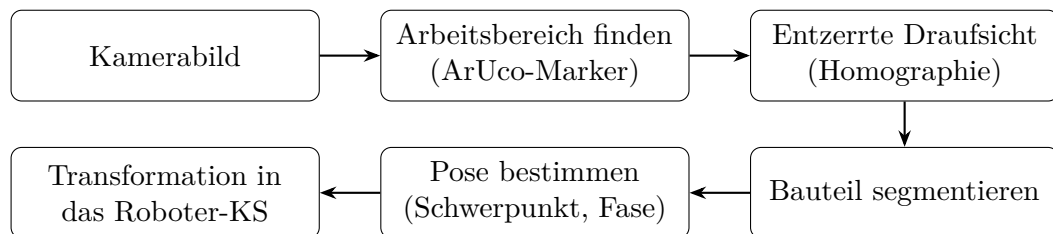
Abbildung 4.1: Verarbeitungskette der Objekterkennung
