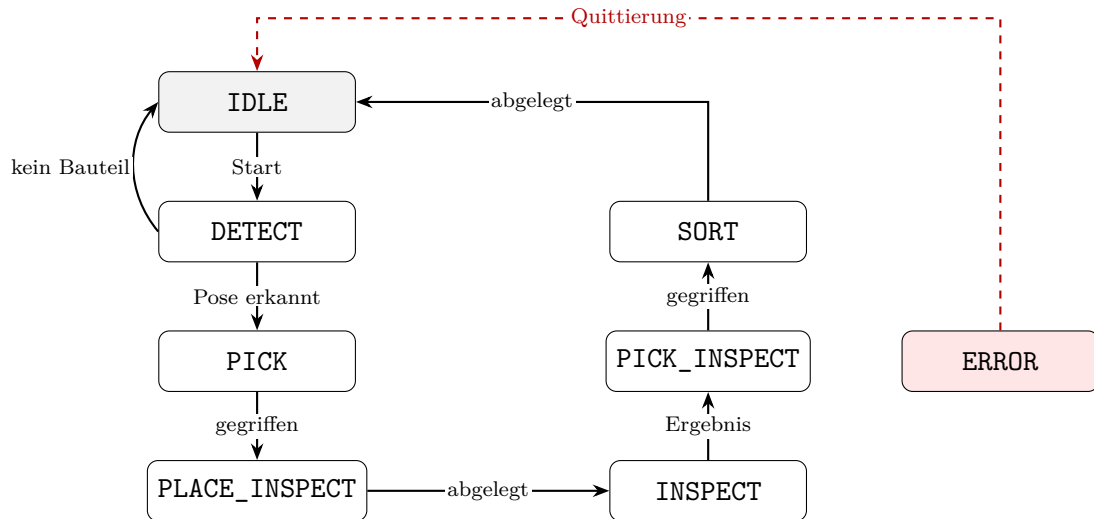
Abbildung 3.3: Zustandsautomat eines Arbeitszyklus. Aus jedem Zustand außer IDLE führt ein Fehler in den Zustand ERROR (nicht eingezeichnet).
