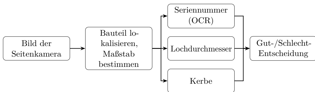
Abbildung 6.1: Ablauf der Sichtprüfung. Die drei Merkmale werden unabhängig voneinander bestimmt und gemeinsam bewertet.
