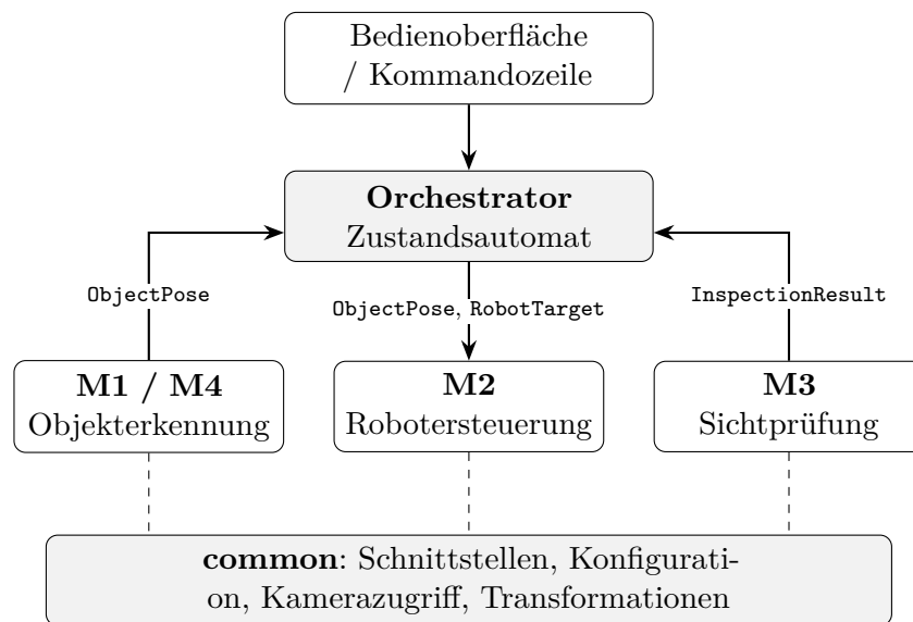
Abbildung 3.2: Modulstruktur der Software
