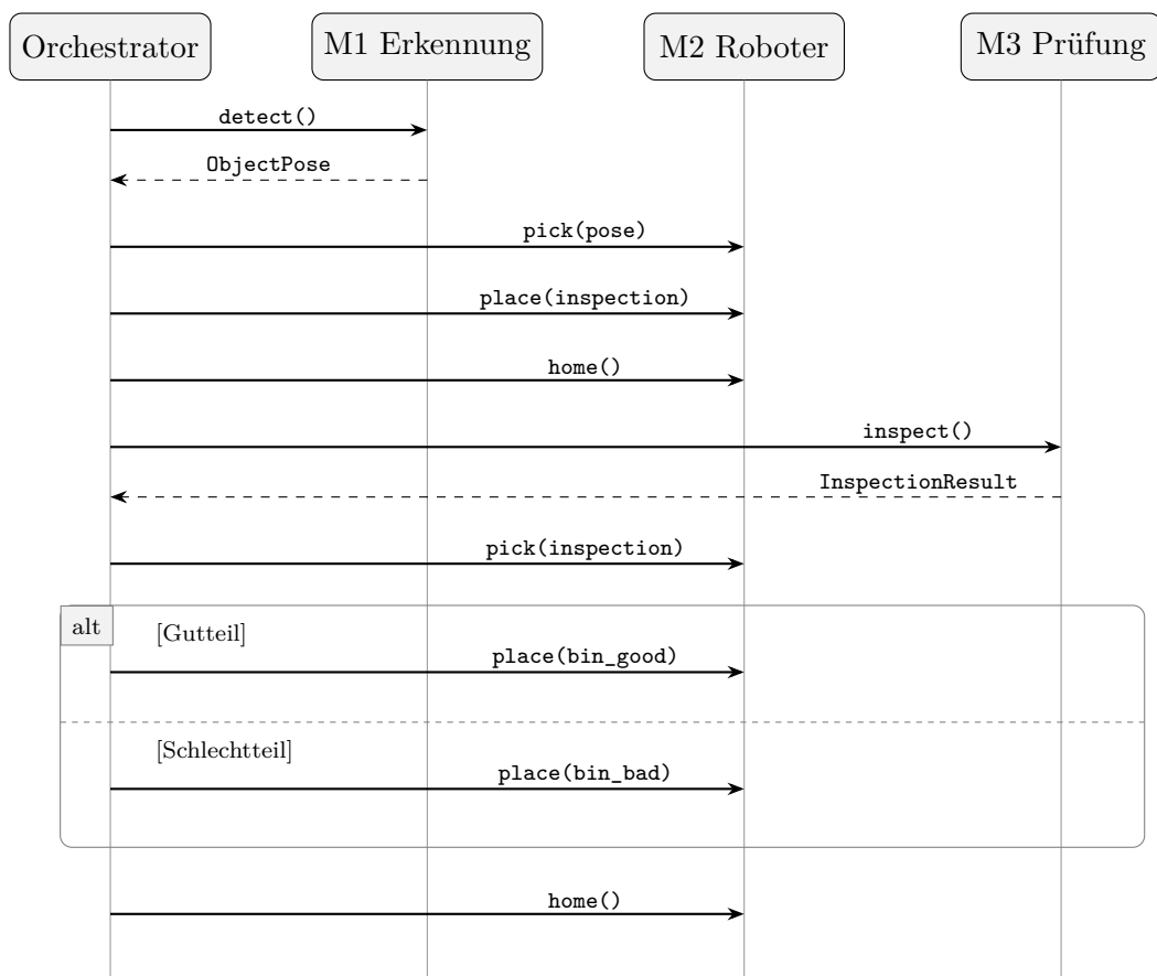
Abbildung 8.1: Aufrufe des Orchestrators an die Module während eines Arbeitszyklus
