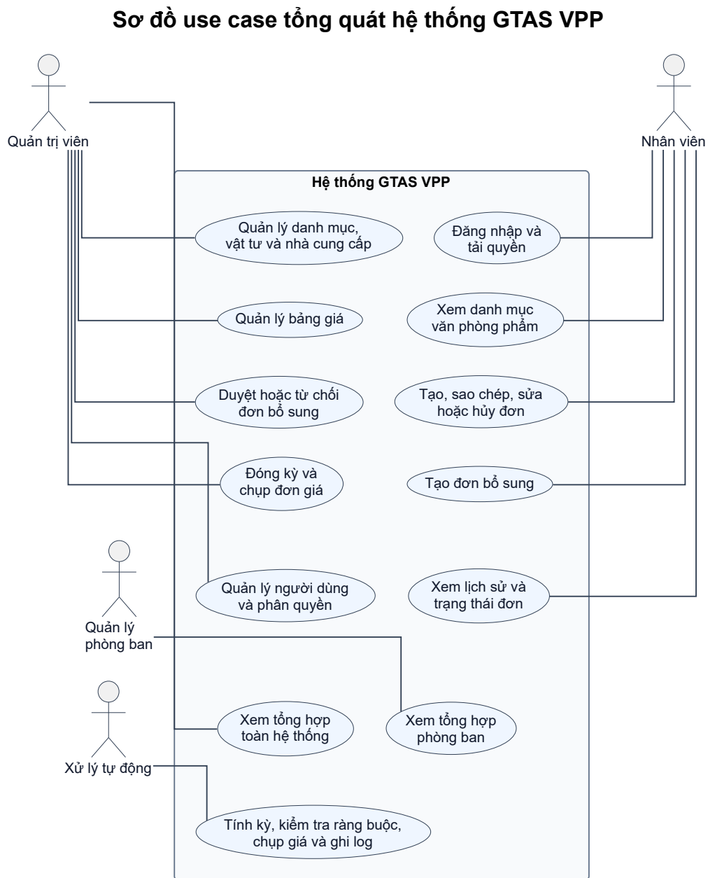
Hình 2-3: Sơ đồ use case tổng quát hệ thống
