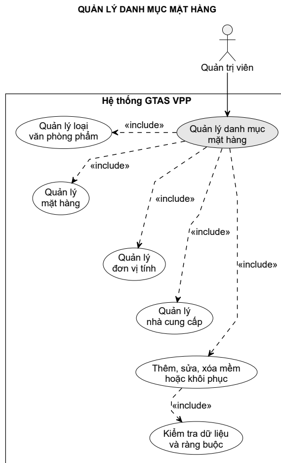
Hình 3-10: Sơ đồ use case chức năng quản lý danh mục mặt hàng
