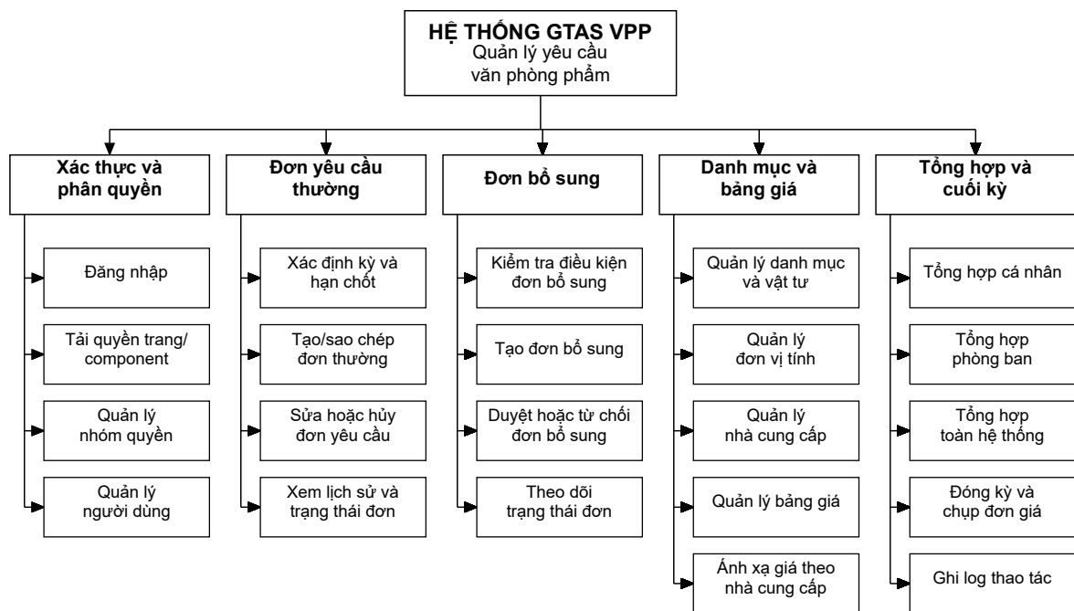
Hình 2-2: Sơ đồ phân rã chức năng hệ thống
