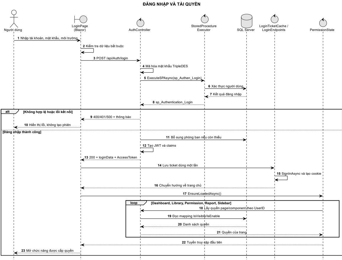
Hình 3-15: Sơ đồ tuần tự chức năng đăng nhập và tải quyền
