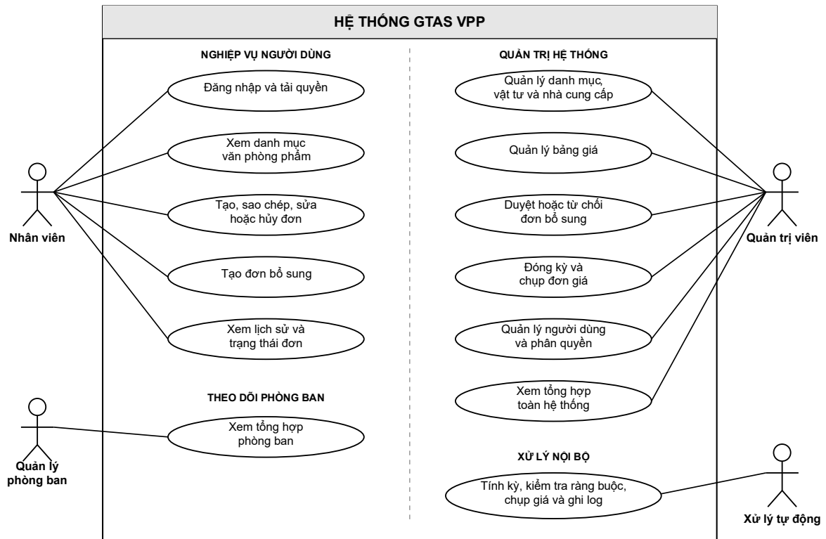
Hình 2-3: Sơ đồ use case tổng quát hệ thống
