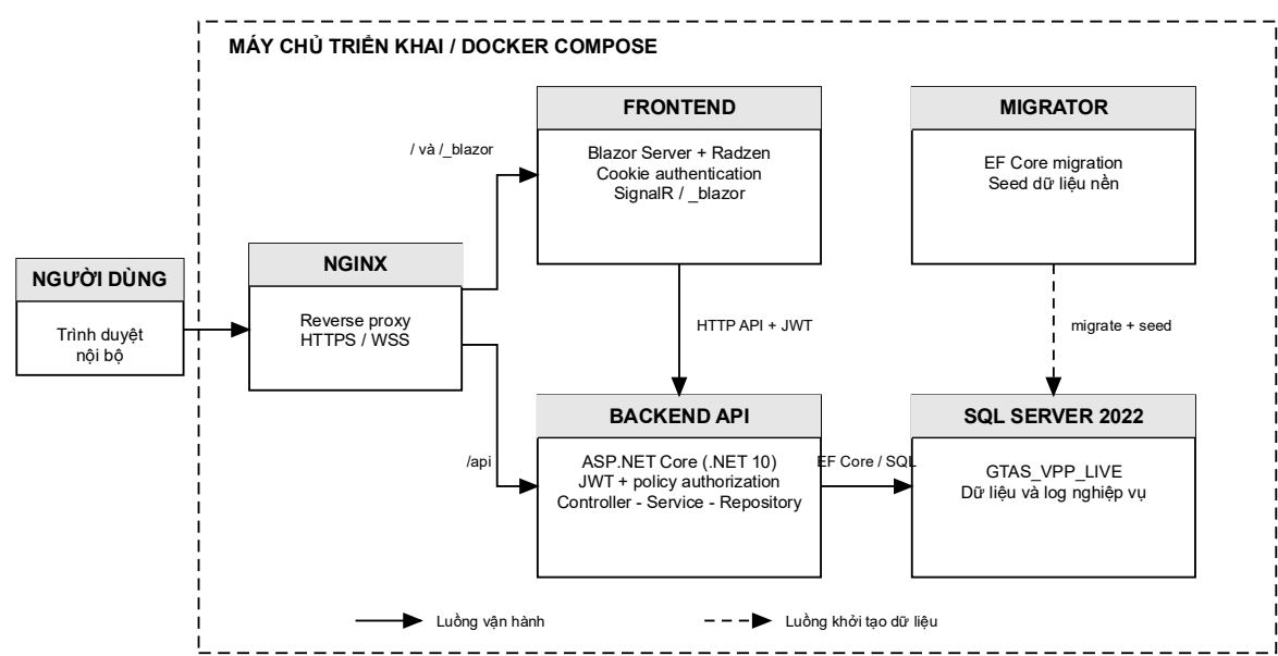
Hình 2-1: Kiến trúc triển khai tổng thể hệ thống GTAS VPP
