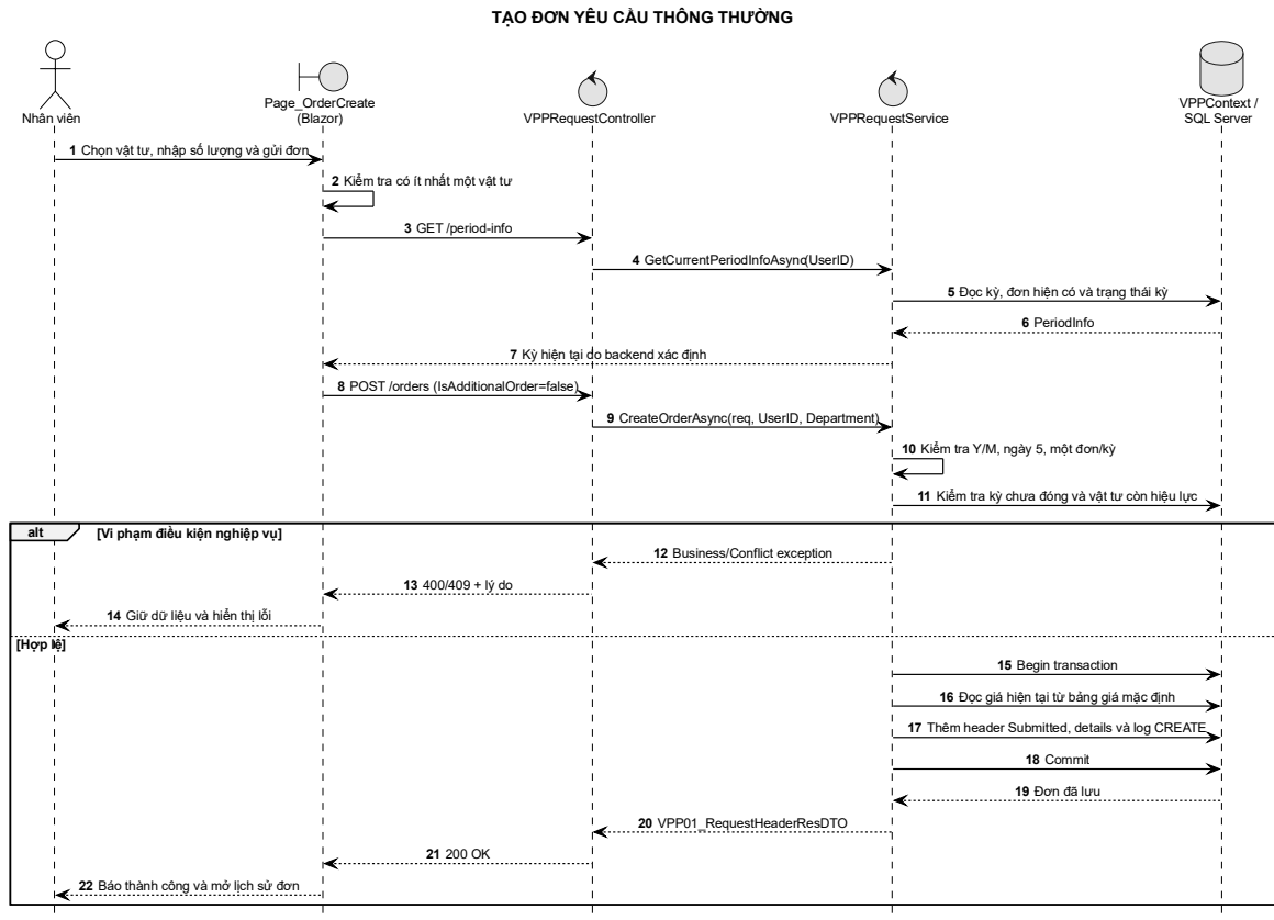
Hình 3-16: Sơ đồ tuần tự chức năng tạo đơn yêu cầu thông thường
