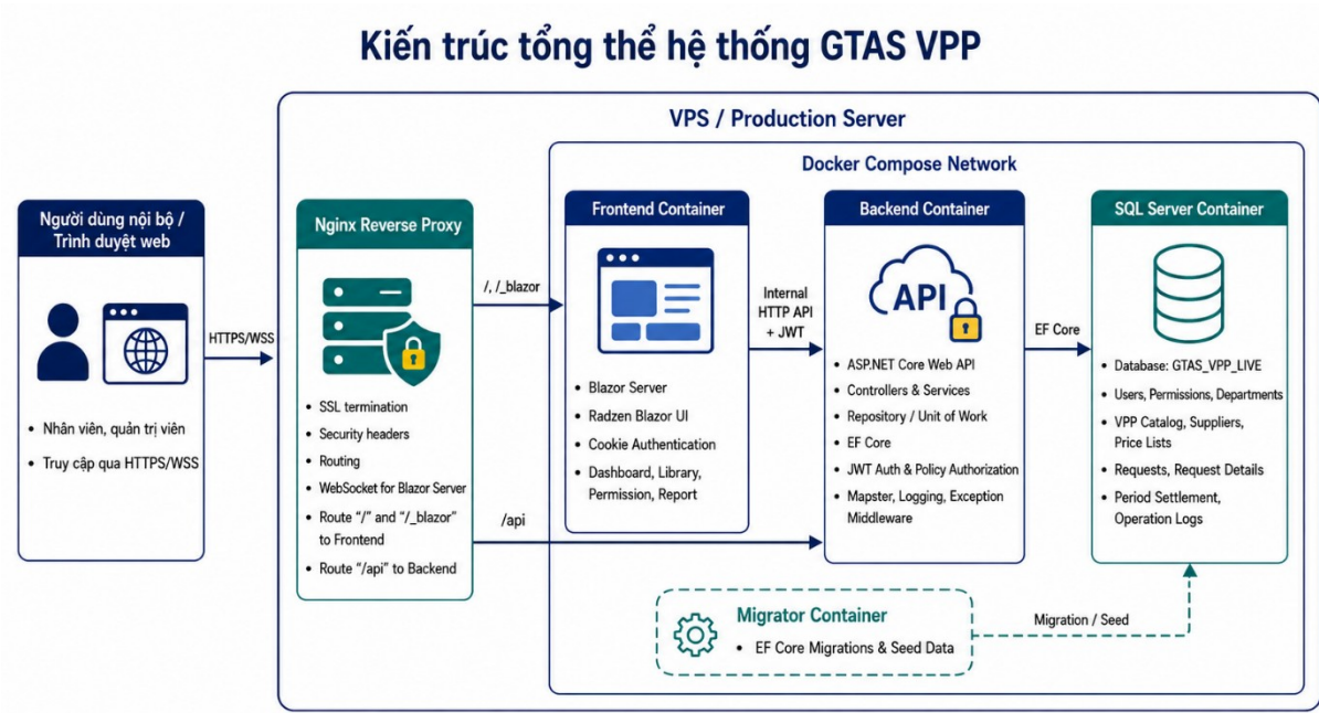
Hình 2-1: Kiến trúc tổng thể hệ thống GTAS VPP
