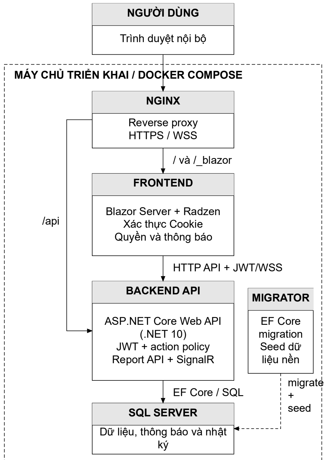
Hình 2-1: Kiến trúc triển khai tổng thể hệ thống GTAS VPP
