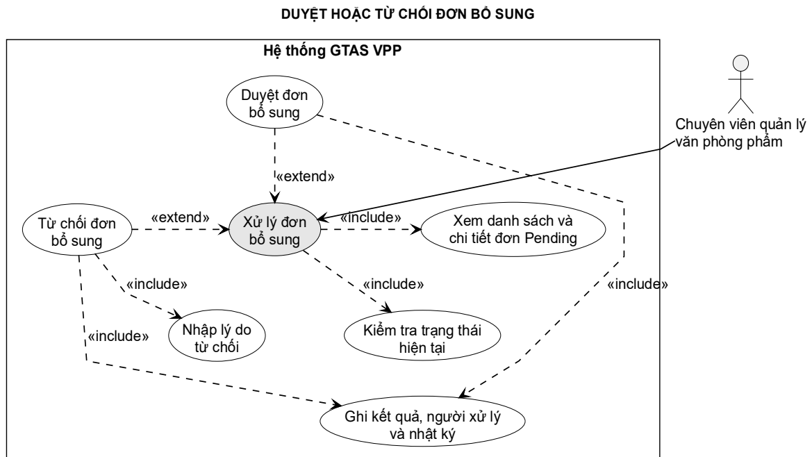
Hình 3-9: Sơ đồ use case chức năng duyệt đơn bổ sung
