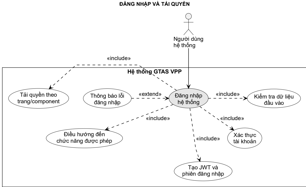
Hình 3-5: Sơ đồ use case chức năng đăng nhập và tải quyền
