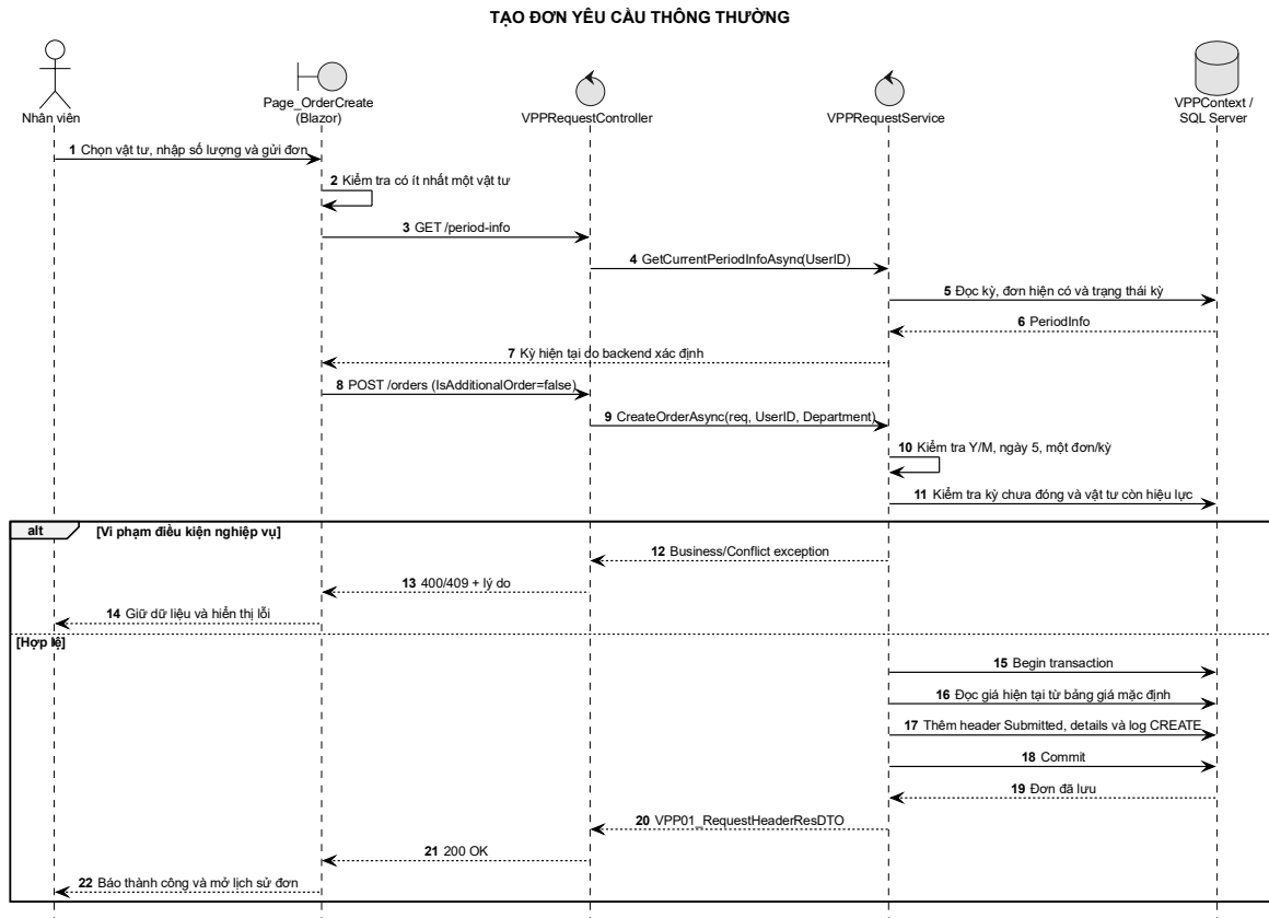
Hình 3-16: Sơ đồ tuần tự chức năng tạo đơn yêu cầu thông thường
