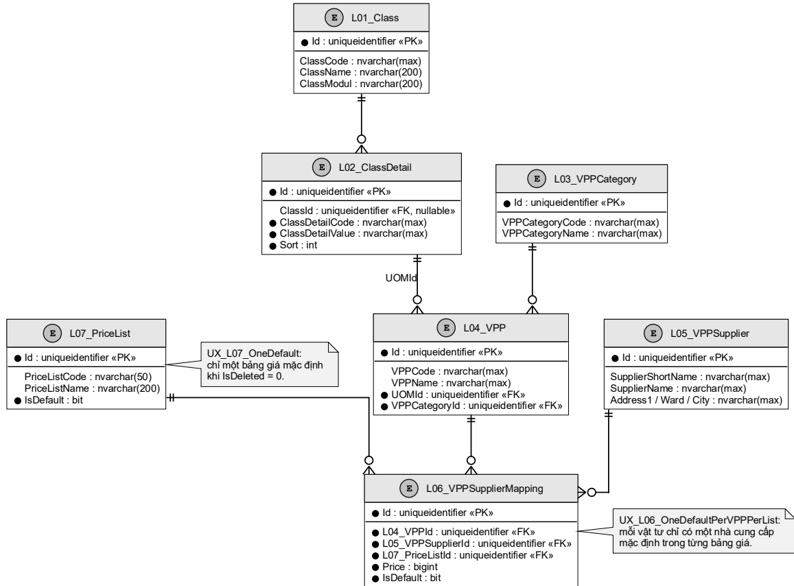
Hình 3-3: ERD luận lý nhóm danh mục và bảng giá
