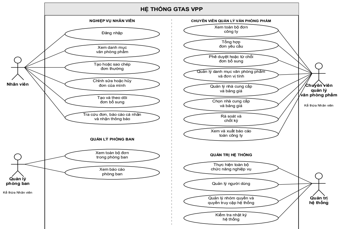
Hình 2-3: Sơ đồ use case tổng quát hệ thống
