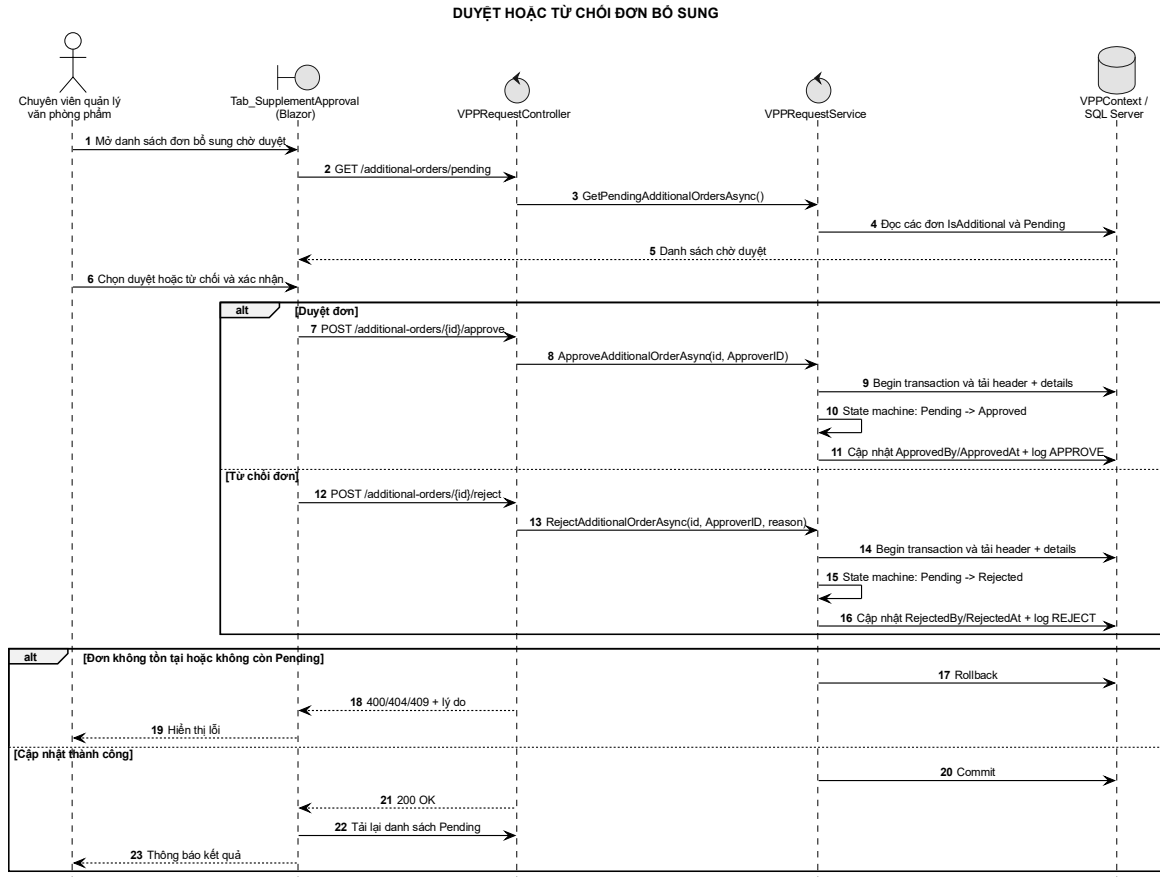
Hình 3-18: Sơ đồ tuần tự chức năng duyệt đơn bổ sung
