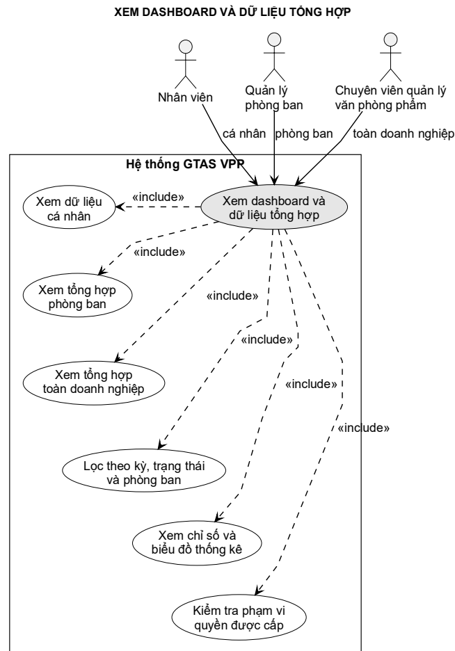
Hình 3-14: Sơ đồ use case chức năng xem dashboard và dữ liệu tổng hợp
