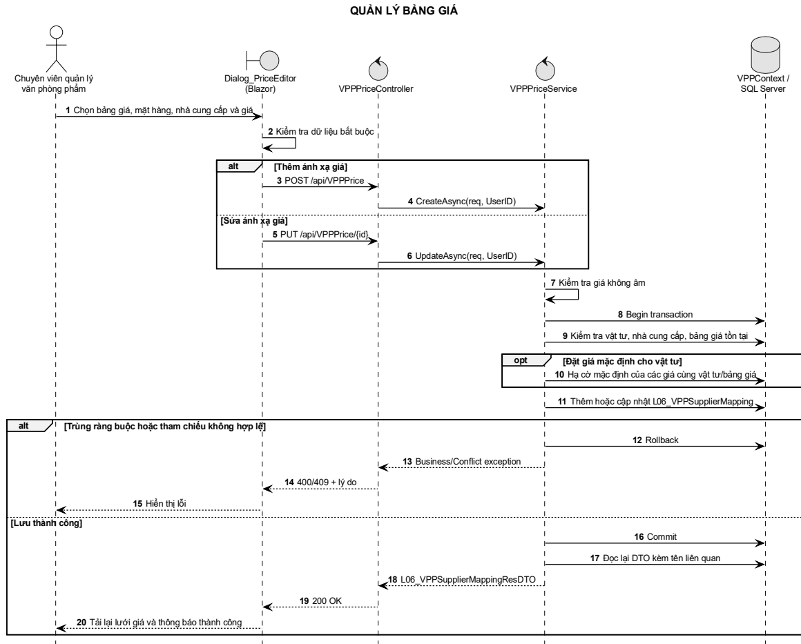
Hình 3-20: Sơ đồ tuần tự chức năng quản lý bảng giá
