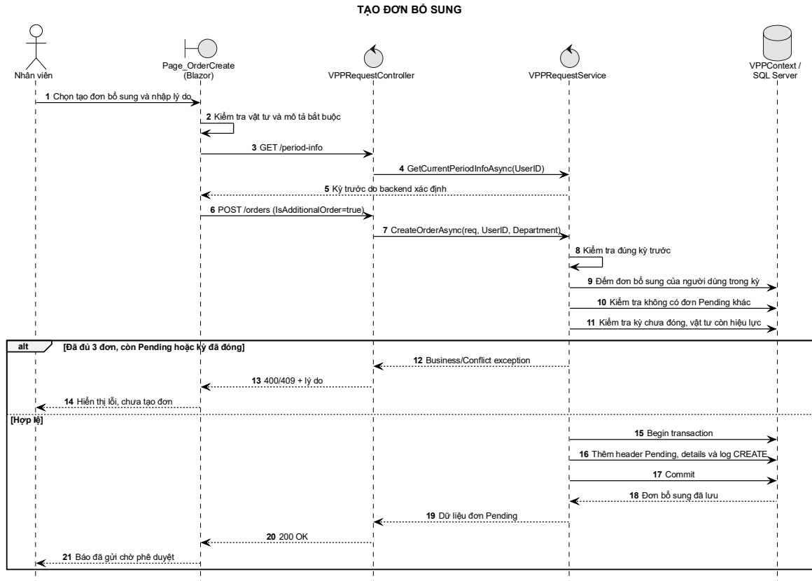
Hình 3-17: Sơ đồ tuần tự chức năng tạo đơn bổ sung
