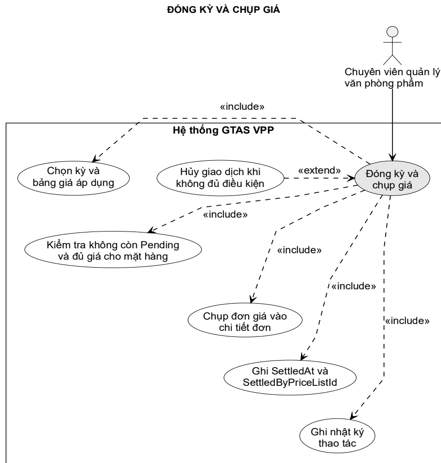
Hình 3-12: Sơ đồ use case chức năng đóng kỳ và chụp giá
