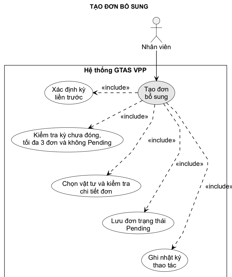
Hình 3-8: Sơ đồ use case chức năng tạo đơn bổ sung
