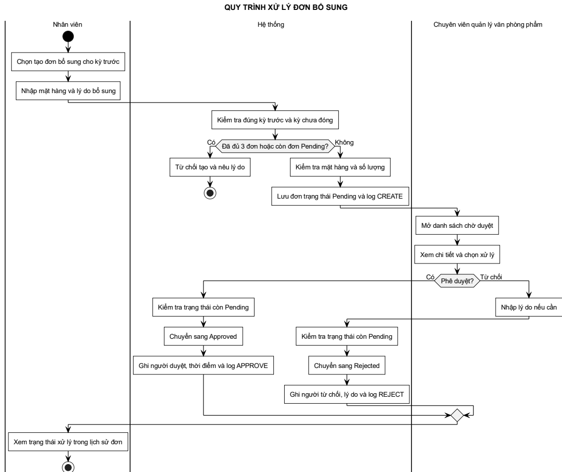
Hình 3-22: Sơ đồ hoạt động quy trình xử lý đơn bổ sung
