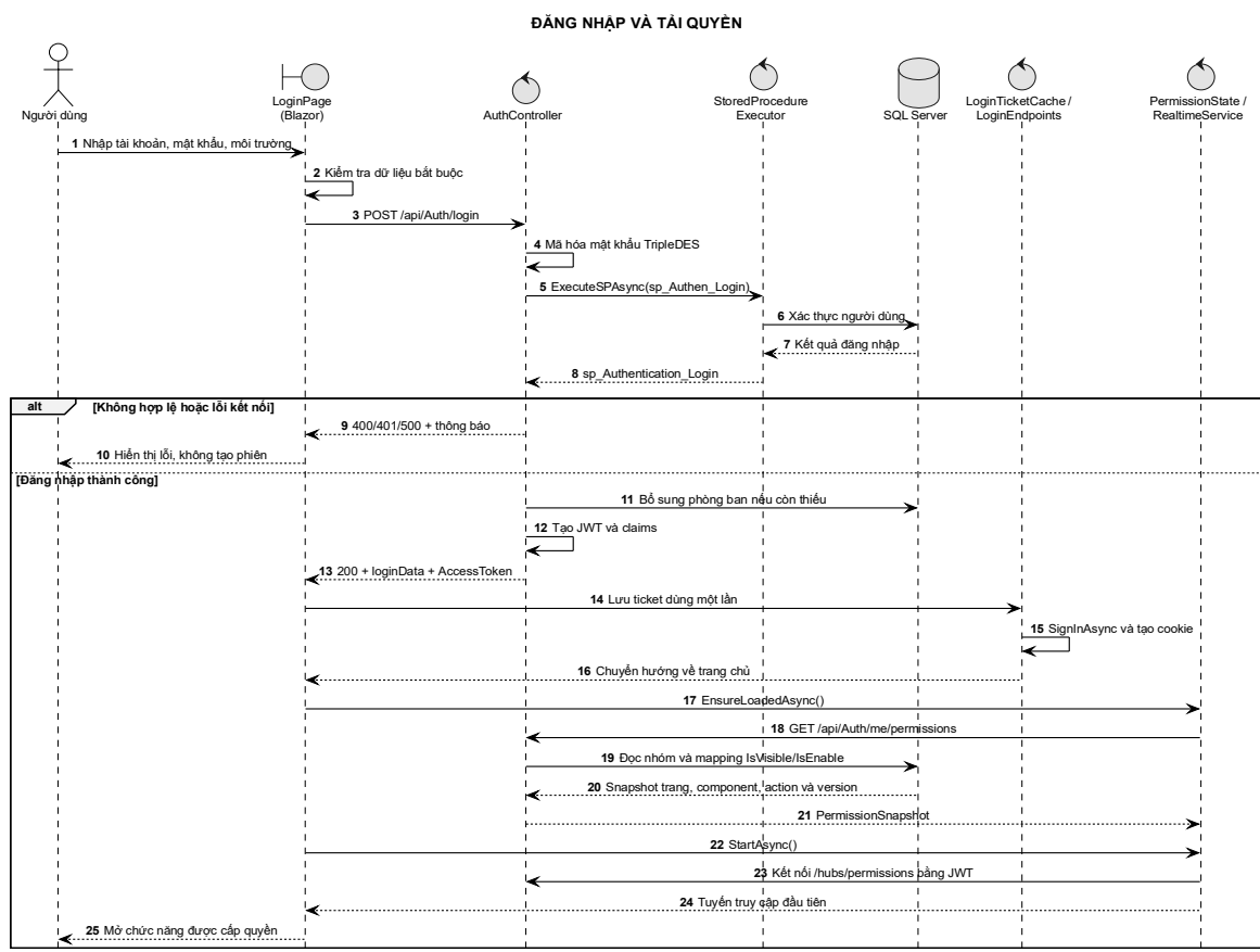
Hình 3-15: Sơ đồ tuần tự chức năng đăng nhập và tải quyền
