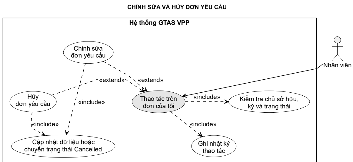
Hình 3-7: Sơ đồ use case chức năng chỉnh sửa và hủy đơn
