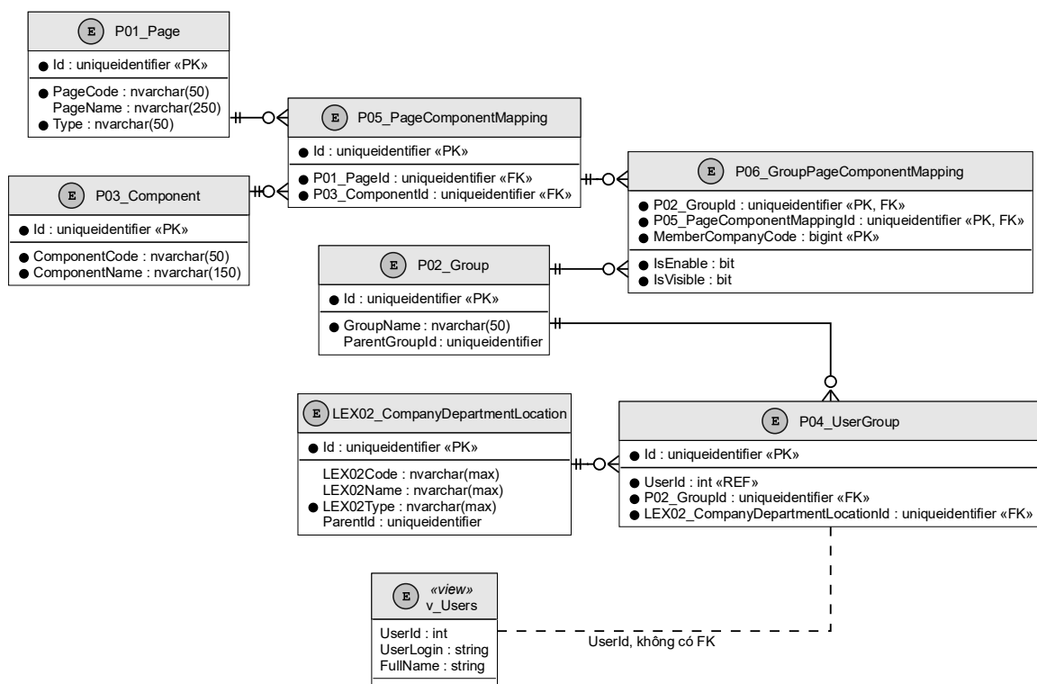
Hình 3-2: ERD luận lý nhóm tổ chức và phân quyền
