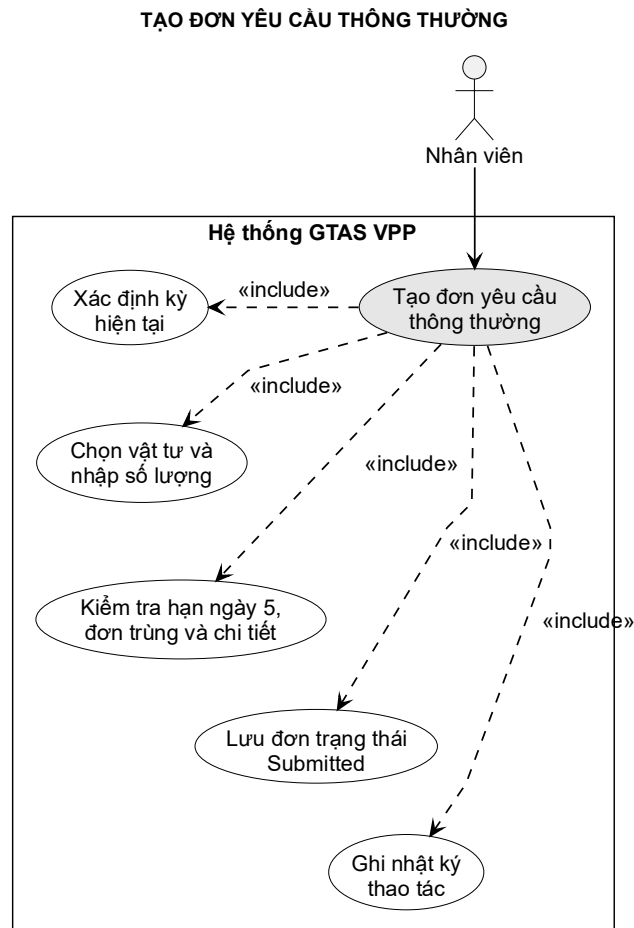
Hình 3-6: Sơ đồ use case chức năng tạo đơn yêu cầu thông thường
