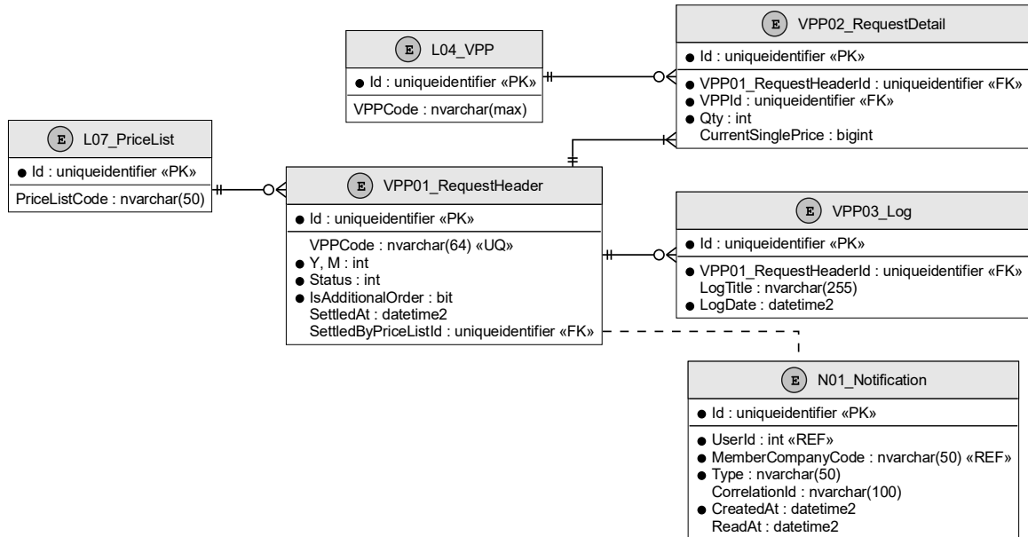
Hình 3-4: ERD luận lý nhóm đơn yêu cầu và nhật ký
