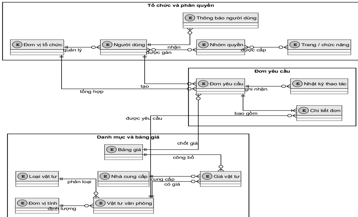
Hình 3-1: Mô hình dữ liệu ý niệm của hệ thống GTAS VPP
