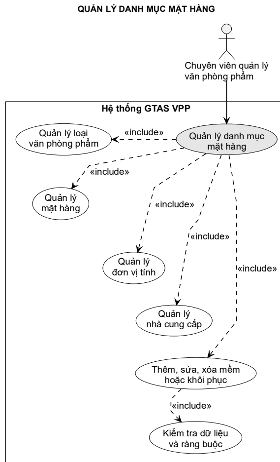
Hình 3-10: Sơ đồ use case chức năng quản lý danh mục văn phòng phẩm
