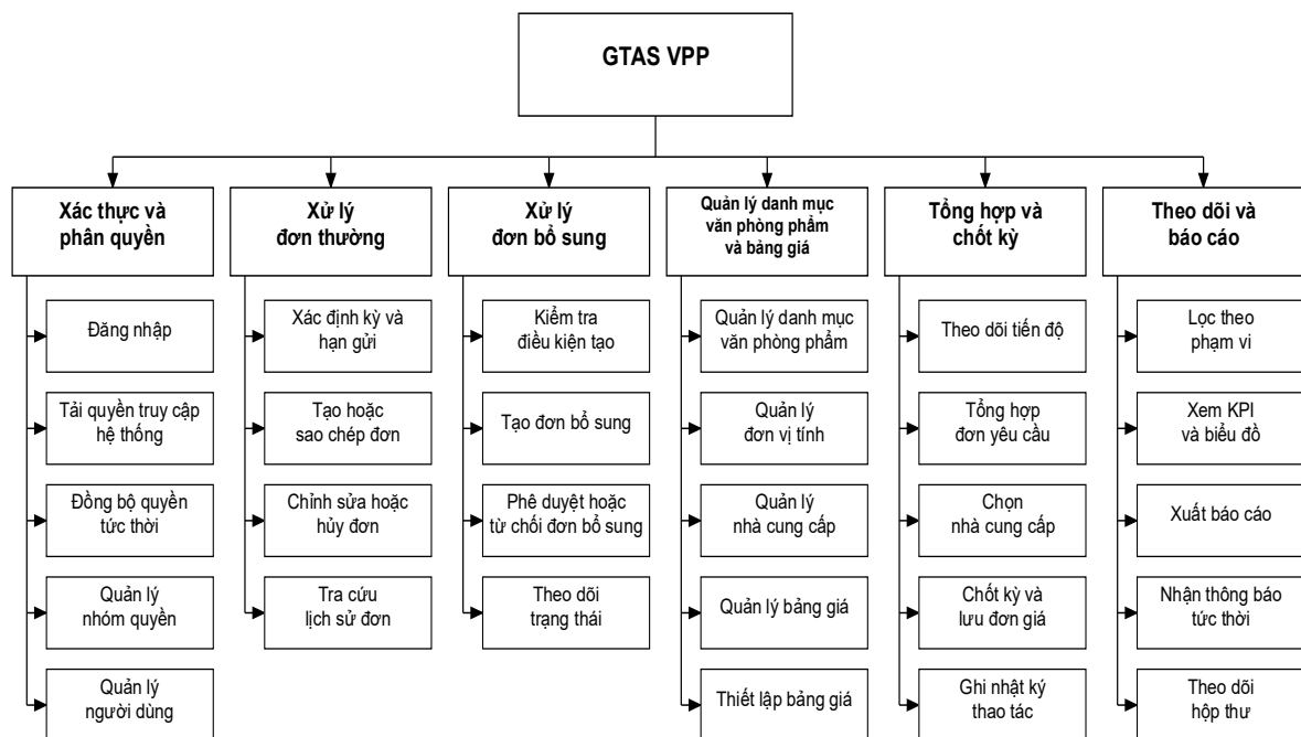
Hình 2-2: Sơ đồ chức năng
