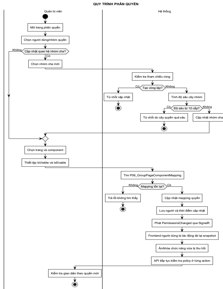
Hình 3-25: Sơ đồ hoạt động quy trình phân quyền
