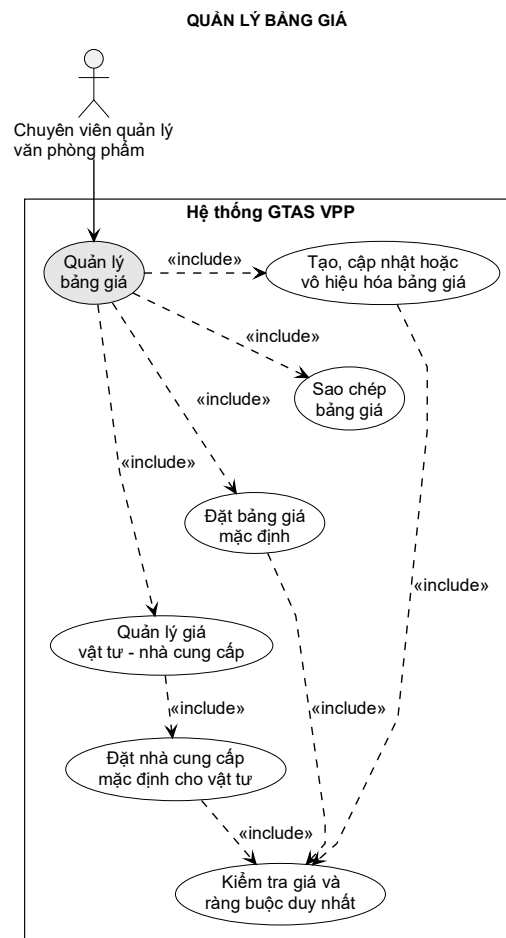
Hình 3-11: Sơ đồ use case chức năng quản lý bảng giá
