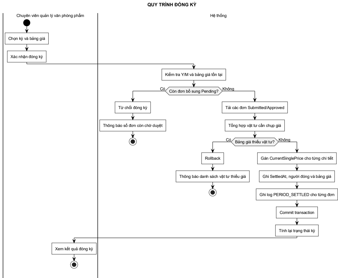
Hình 3-23: Sơ đồ hoạt động quy trình đóng kỳ
