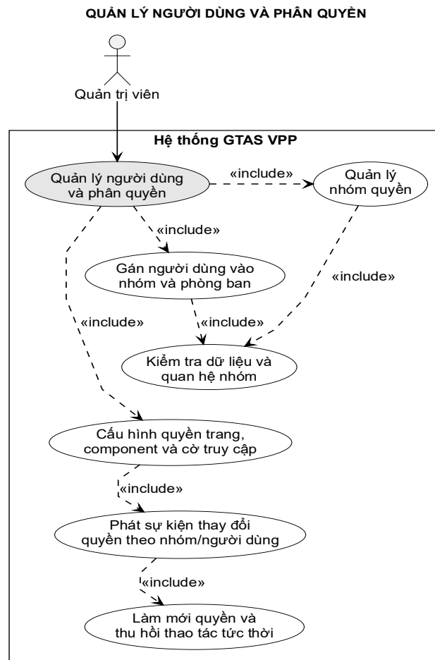
Hình 3-13: Sơ đồ use case chức năng quản lý người dùng và phân quyền
