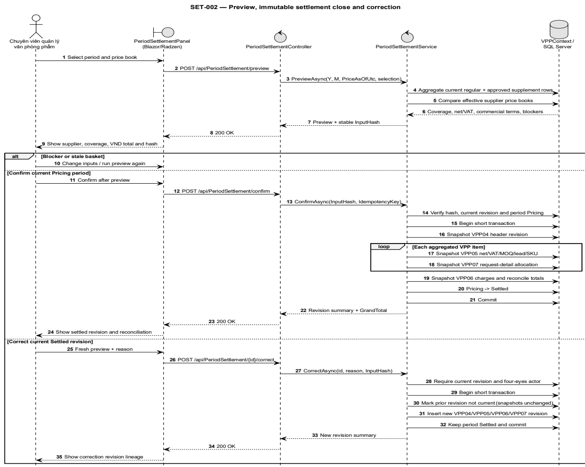
Hình 3-19: Sơ đồ tuần tự chức năng đóng kỳ và chụp giá
