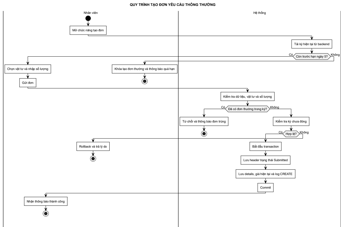
Hình 3-21: Sơ đồ hoạt động quy trình tạo đơn yêu cầu thông thường
