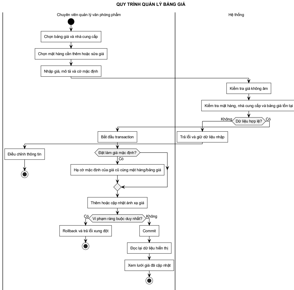
Hình 3-24: Sơ đồ hoạt động quy trình quản lý bảng giá
