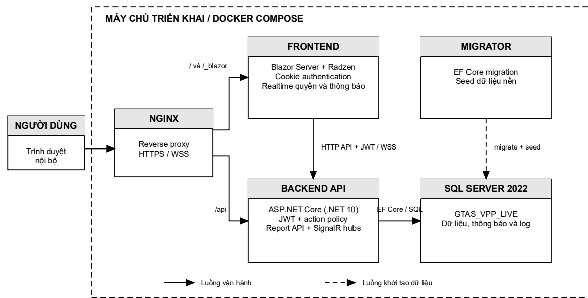
Hình 2-1: Kiến trúc triển khai tổng thể hệ thống GTAS VPP
