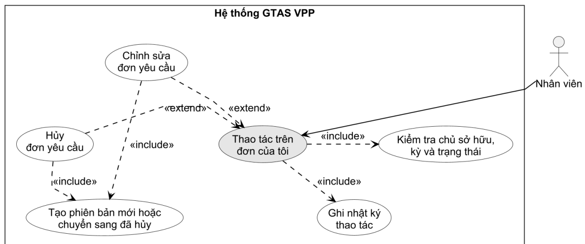
Hình 3-9: Use case chỉnh sửa và hủy đơn
