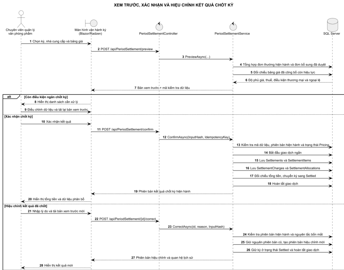
Hình 3-21: Sơ đồ tuần tự xem trước và xác nhận chốt kỳ
