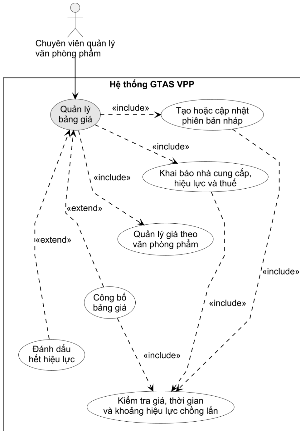
Hình 3-13: Use case quản lý bảng giá
