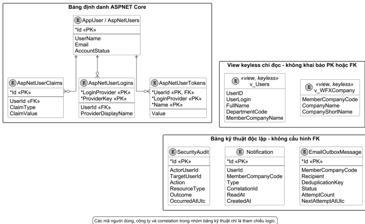
Hình 3-6: Mô hình dữ liệu luận lý về Identity, view keyless và bảng kỹ thuật
