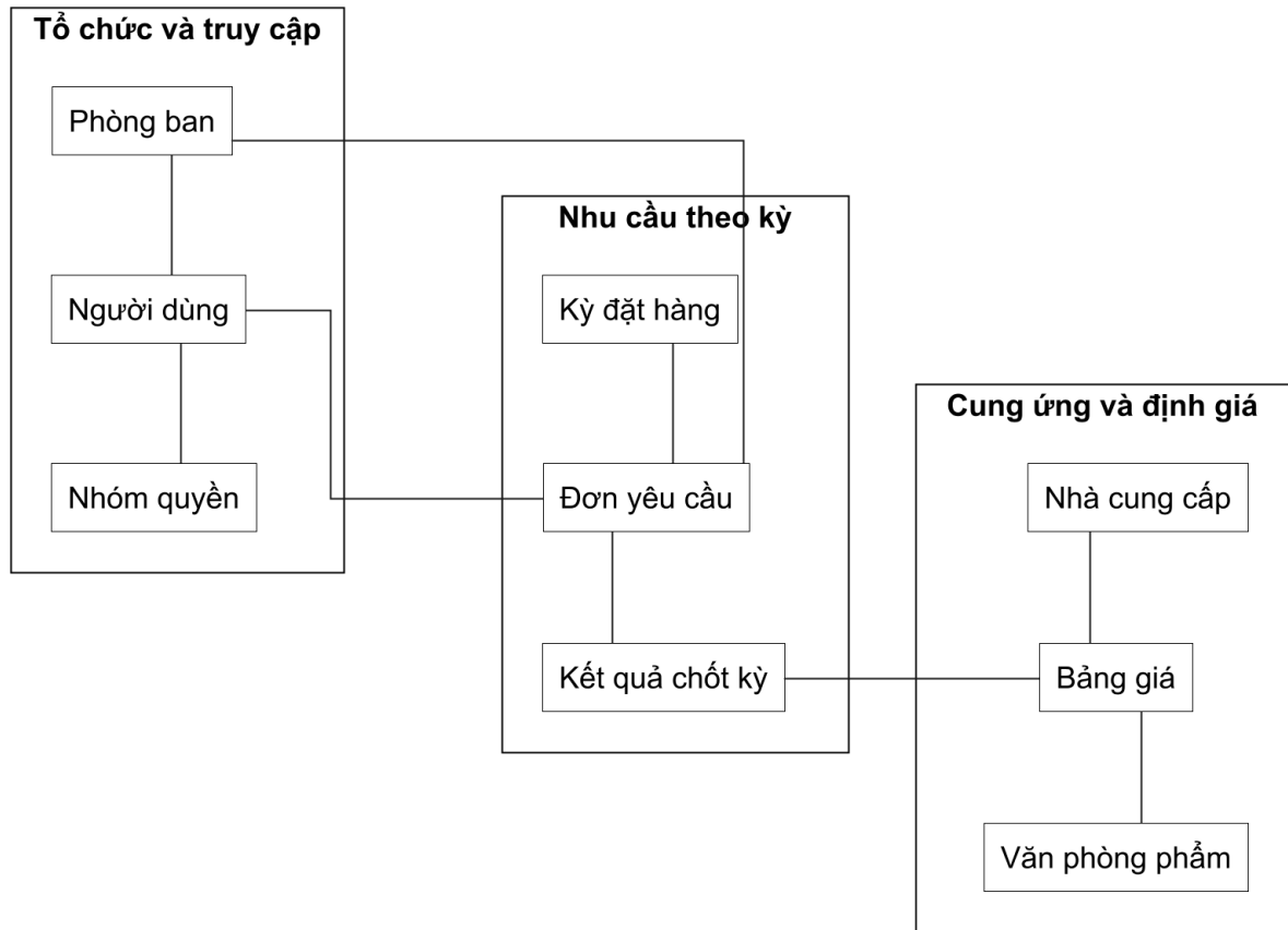
Hình 3-1: Mô hình dữ liệu ý niệm của GTAS VPP
