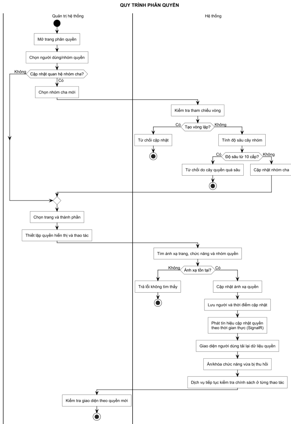
Hình 3-27: Sơ đồ hoạt động quản lý phân quyền
