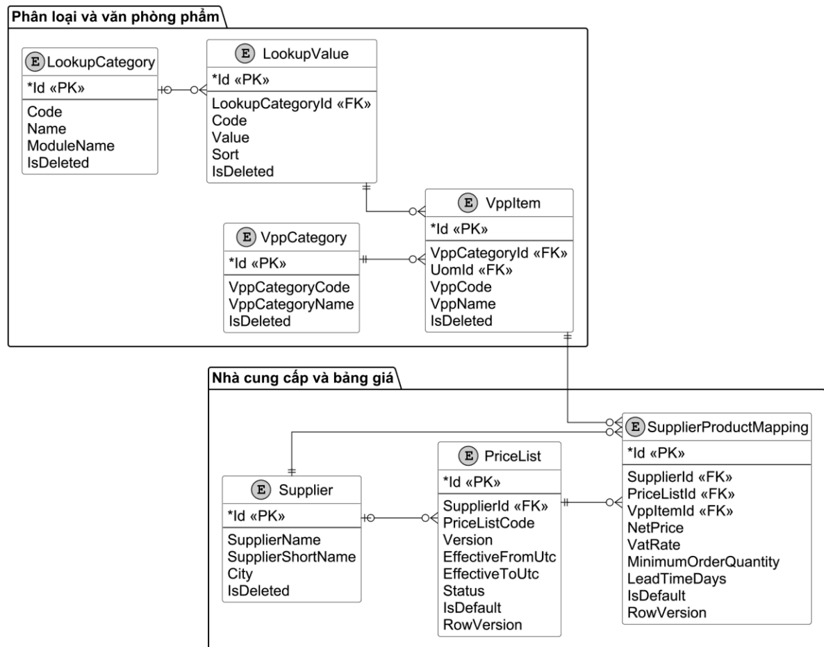
Hình 3-3: Mô hình dữ liệu luận lý về danh mục, nhà cung cấp và bảng giá
