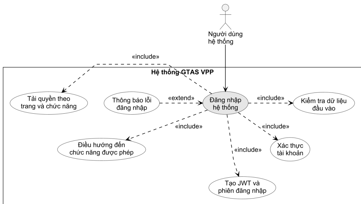
Hình 3-7: Use case đăng nhập và tải quyền
