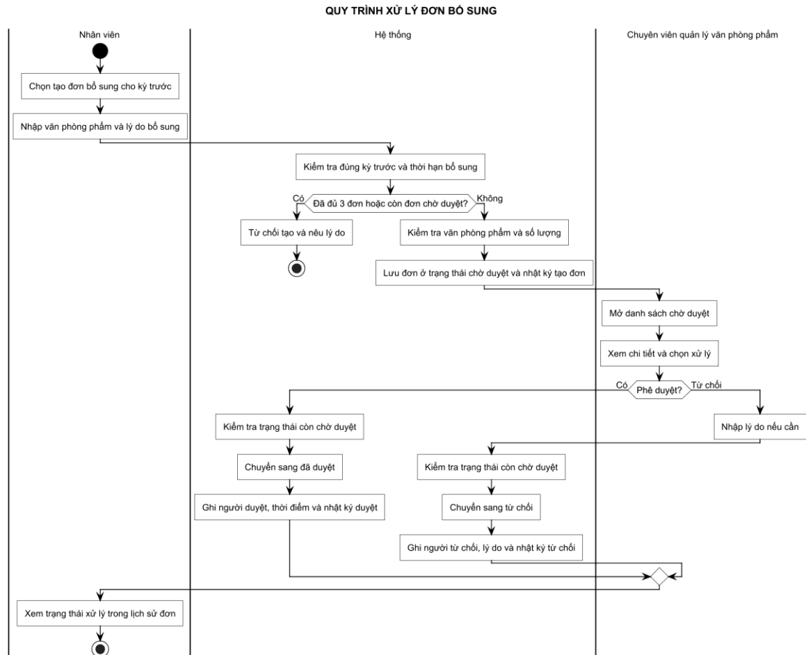
Hình 3-24: Sơ đồ hoạt động xử lý đơn bổ sung
