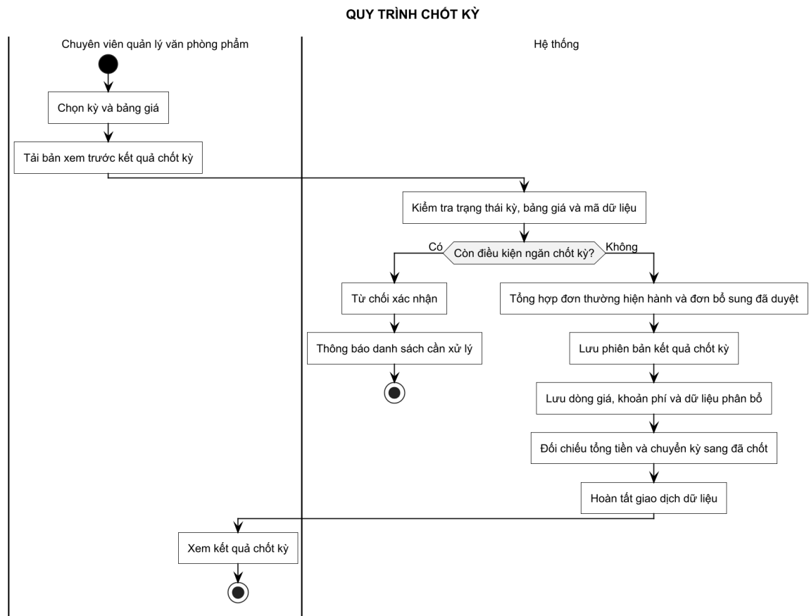
Hình 3-25: Sơ đồ hoạt động xem trước và chốt kỳ
