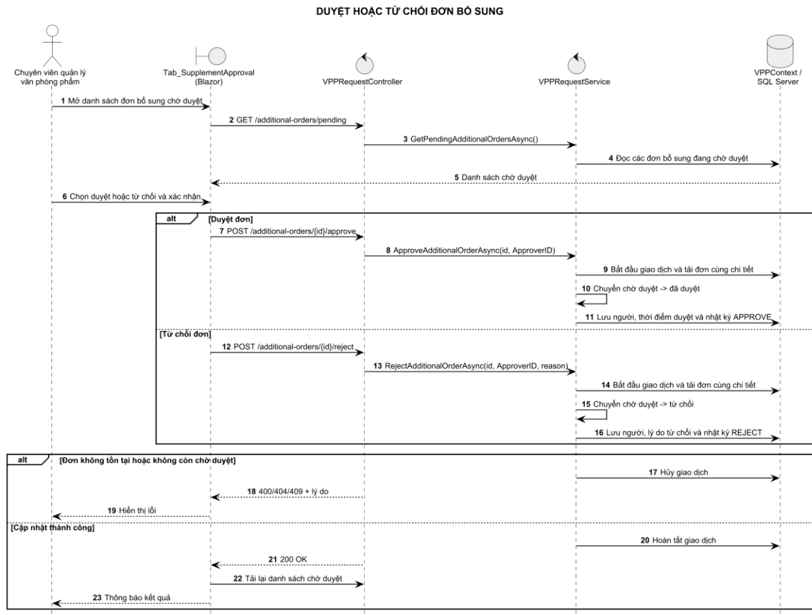
Hình 3-20: Sơ đồ tuần tự duyệt đơn bổ sung
