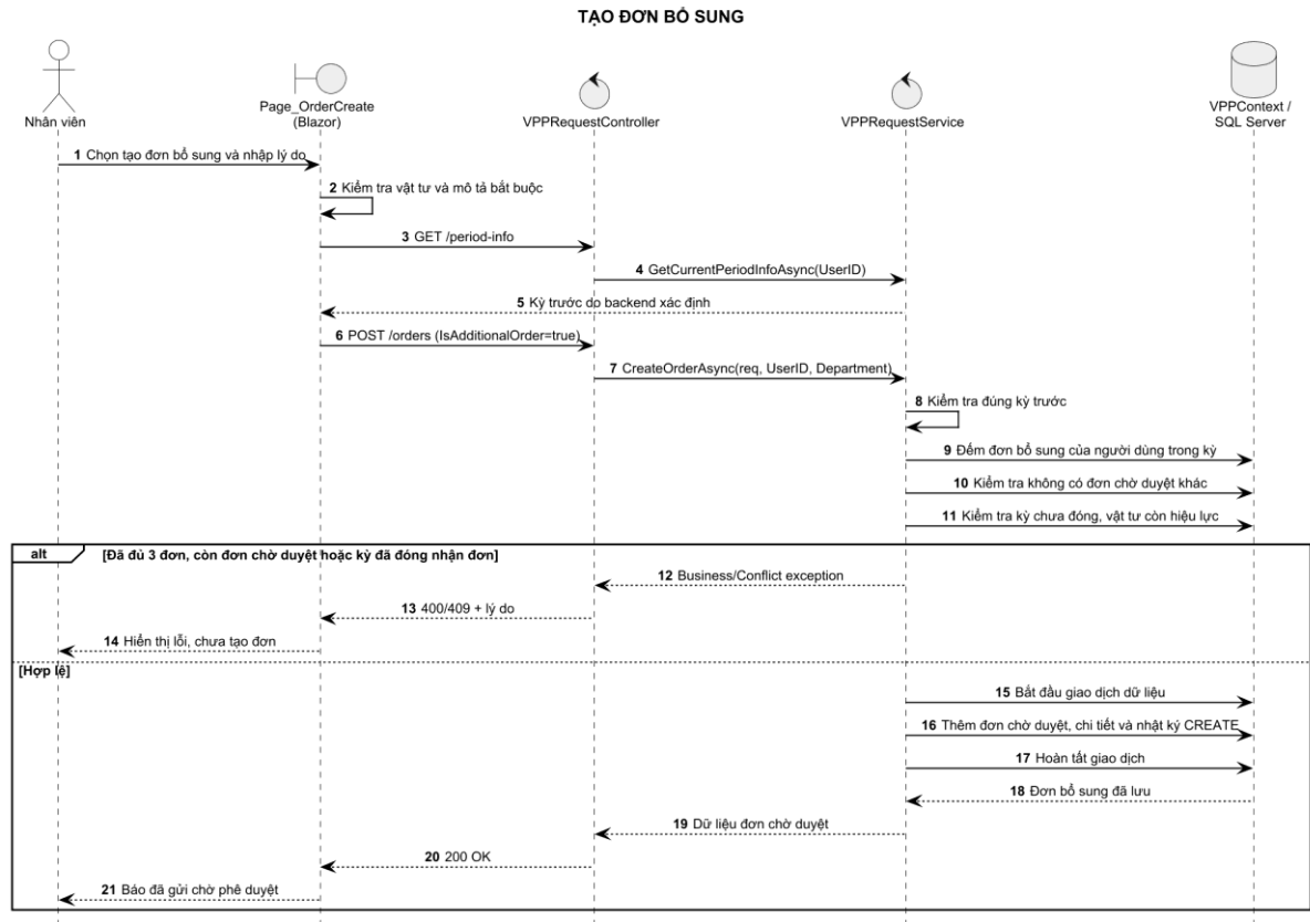
Hình 3-19: Sơ đồ tuần tự tạo đơn bổ sung
