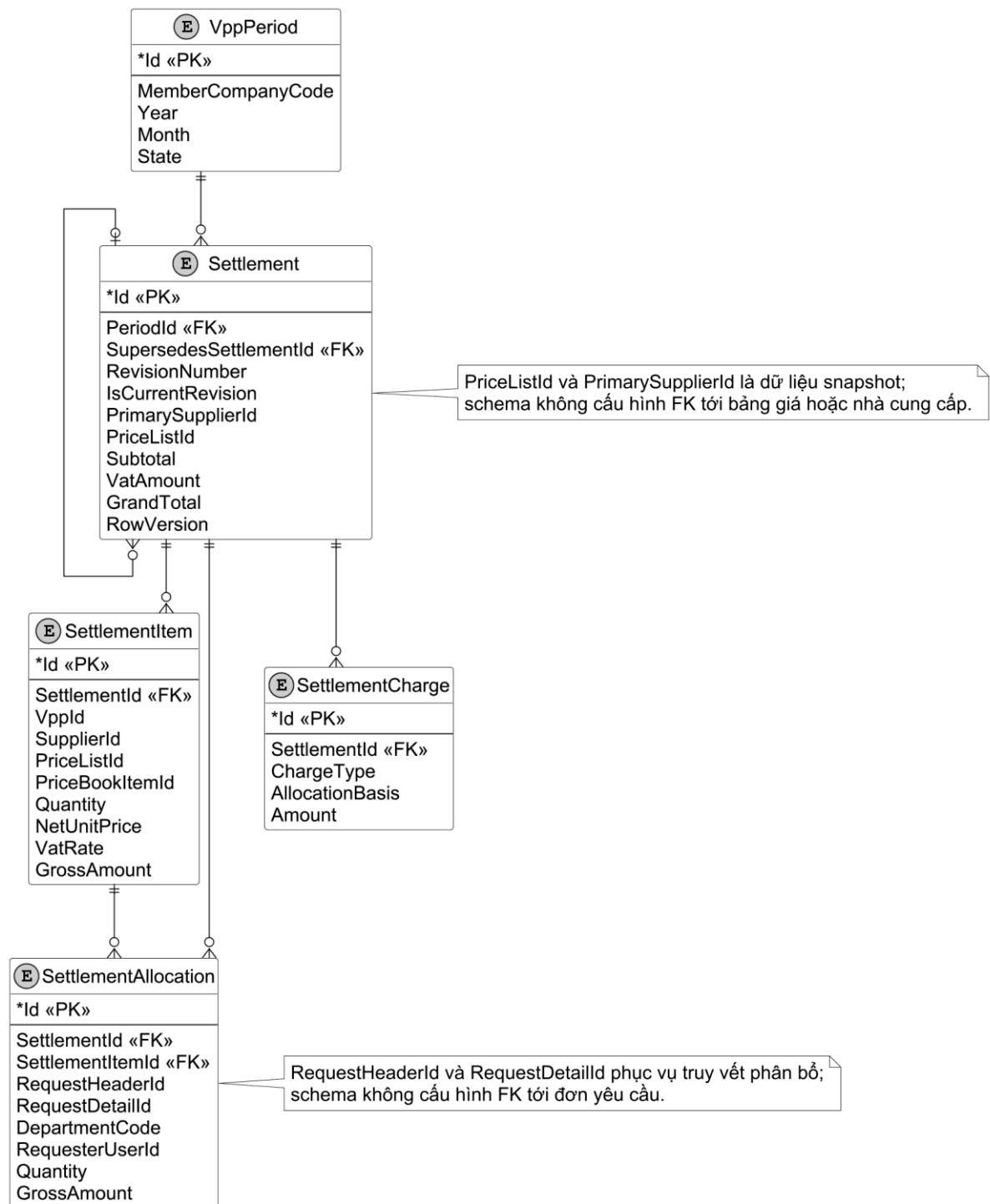
Hình 3-5: Mô hình dữ liệu luận lý về kết quả chốt kỳ, chi phí và phân bổ
