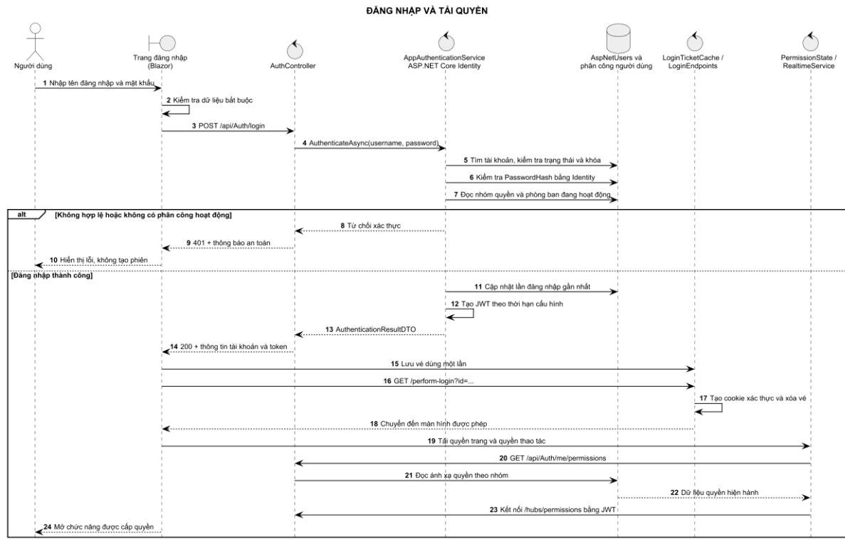
Hình 3-17: Sơ đồ tuần tự đăng nhập và tài quyền
