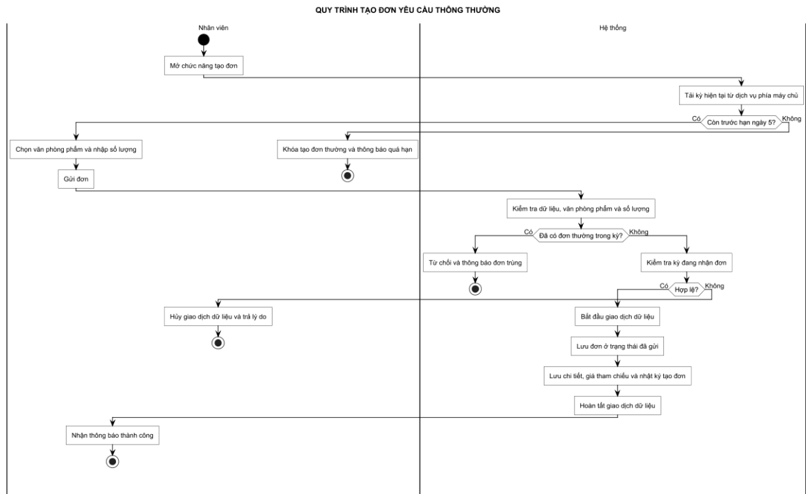
Hình 3-23: Sơ đồ hoạt động tạo đơn yêu cầu thông thường
