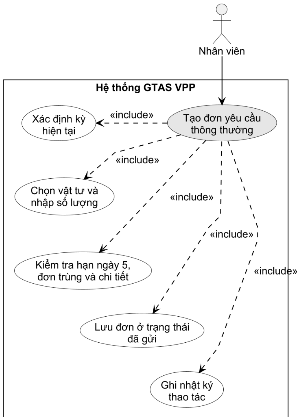
Hình 3-8: Use case tạo đơn yêu cầu thông thường
