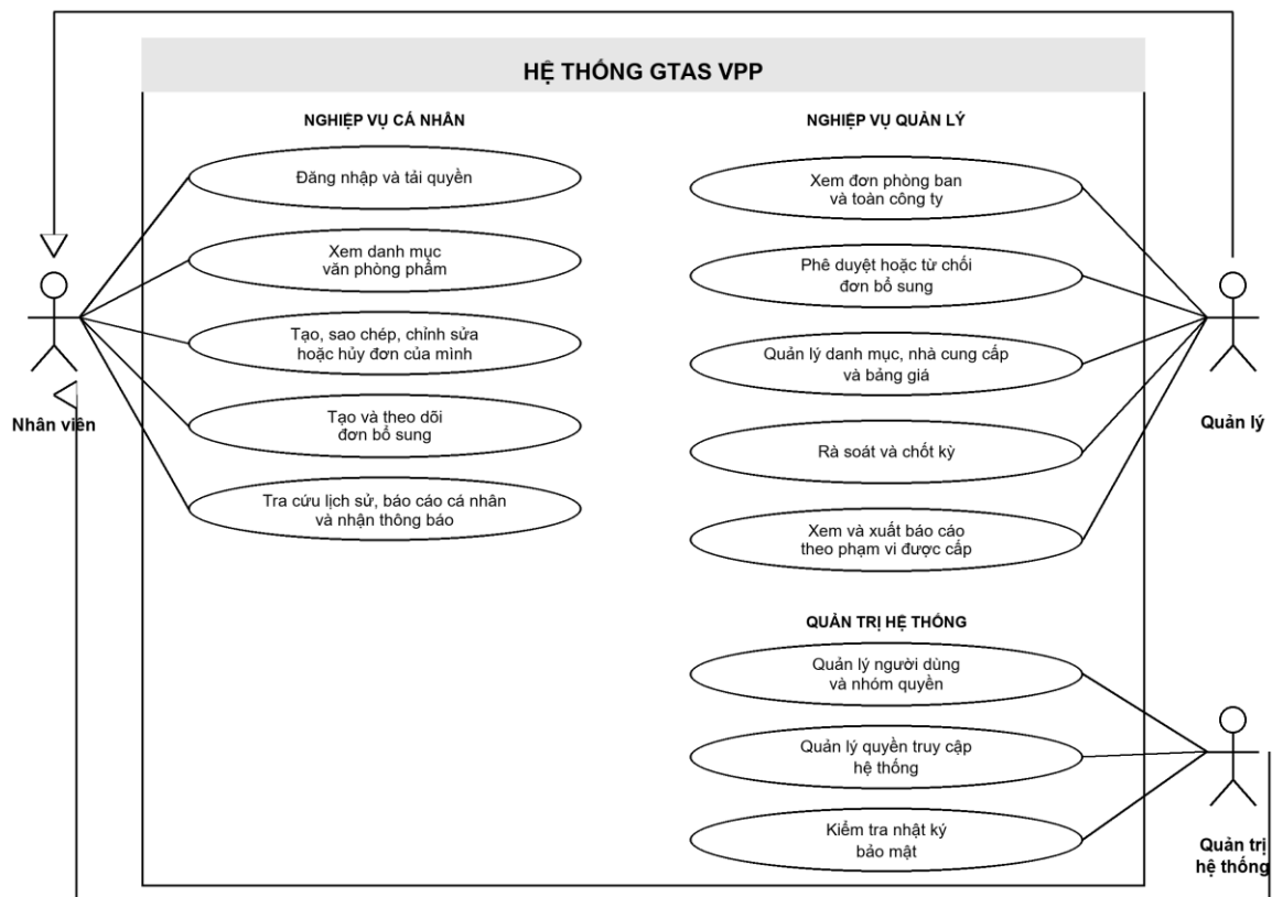
Hình 2-3: Sơ đồ use case tổng quát hệ thống
