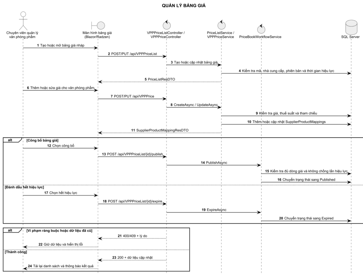
Hình 3-22: Sơ đồ tuần tự quản lý bảng giá
