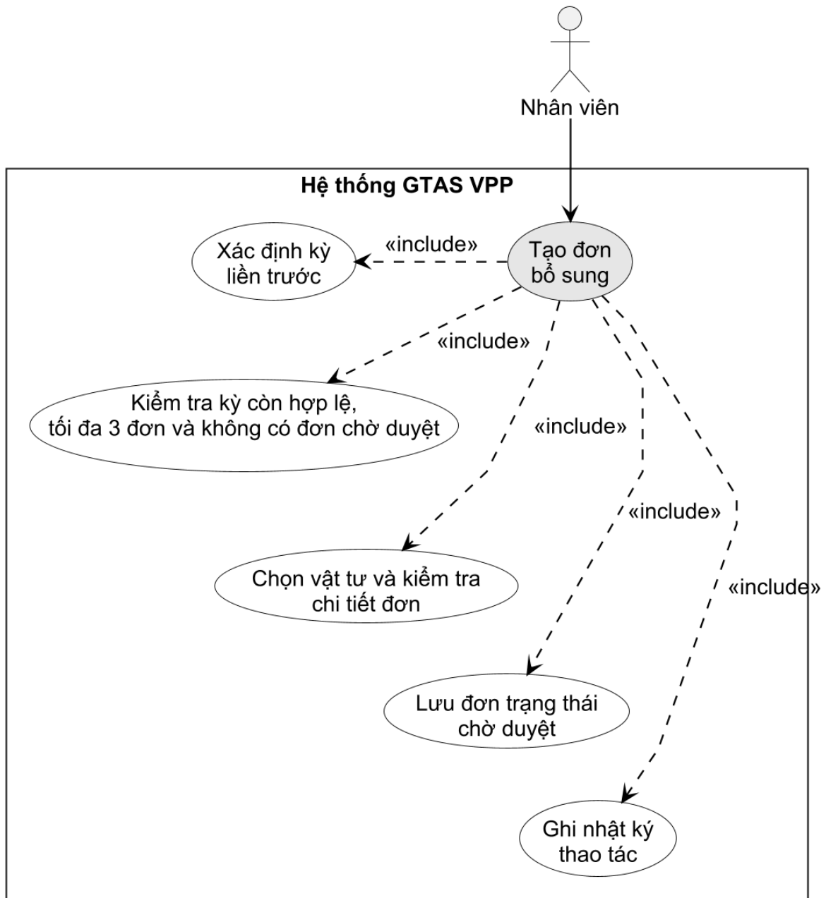
Hình 3-10: Use case tạo đơn bổ sung
