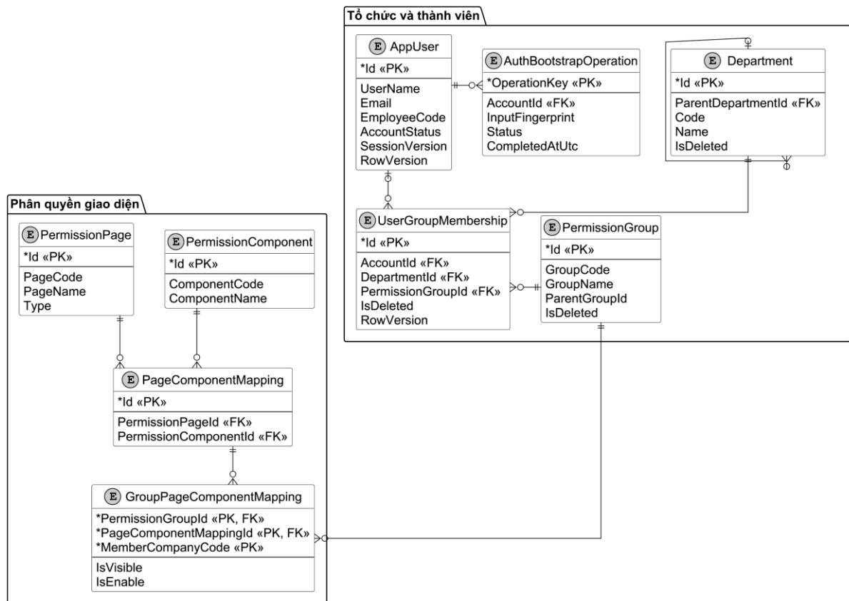
Hình 3-2: Mô hình dữ liệu luận lý về tổ chức và phân quyền
