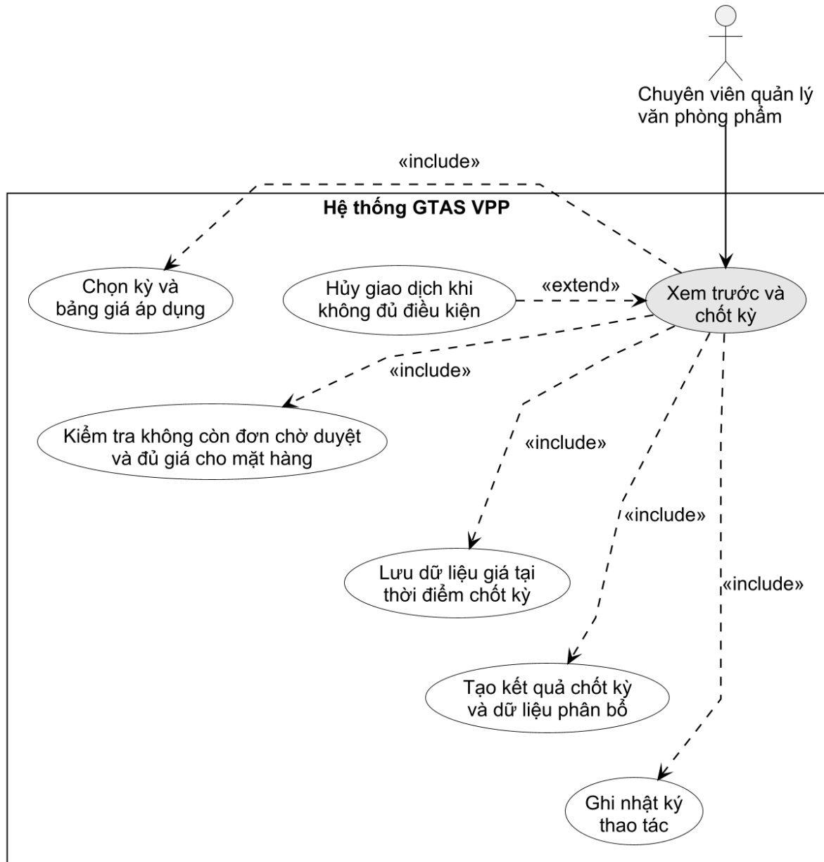
Hình 3-14: Use case xem trước và chốt kỳ
