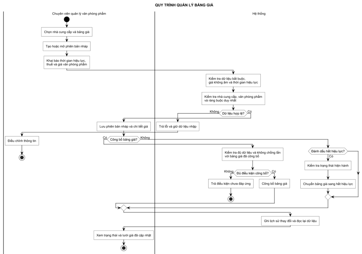
Hình 3-26: Sơ đồ hoạt động quản lý bảng giá
