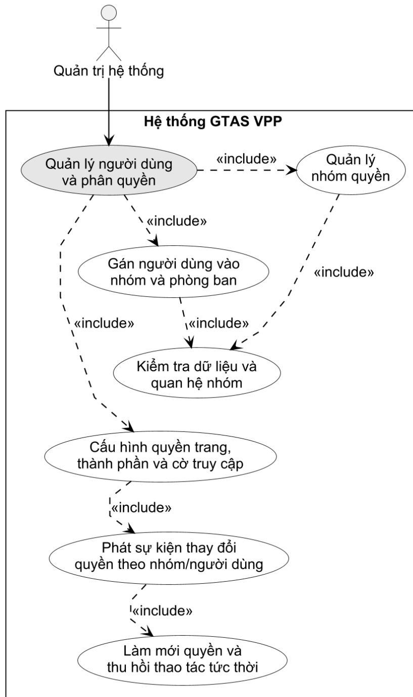
Hình 3-15: Use case quản lý người dùng và phân quyền
