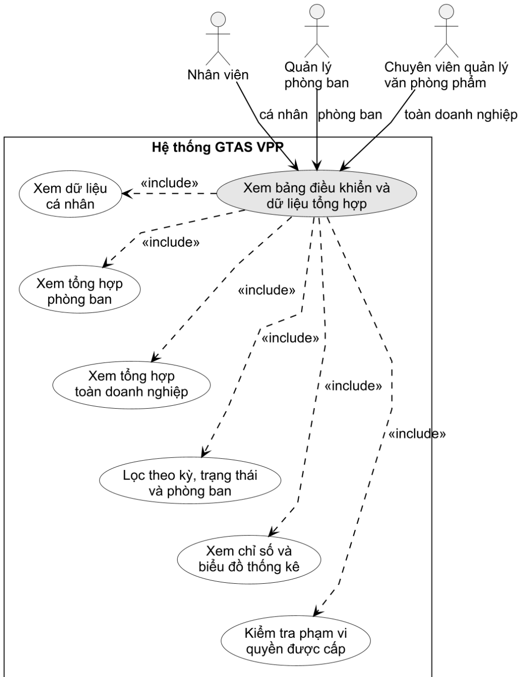
Hình 3-16: Use case xem dashboard và dữ liệu tổng hợp
