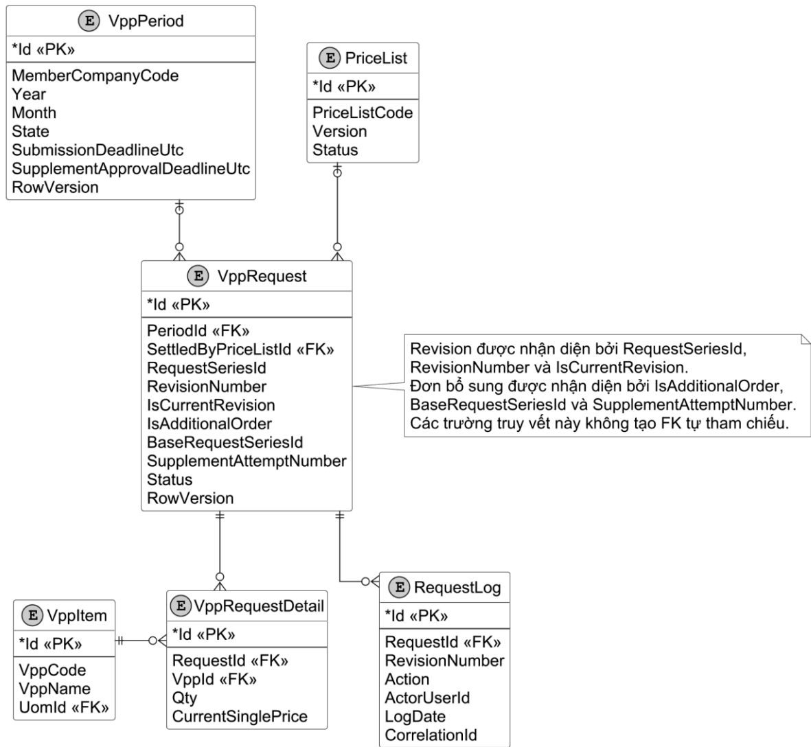
Hình 3-4: Mô hình dữ liệu luận lý về kỳ, đơn yêu cầu, phiên bản và nhật ký
