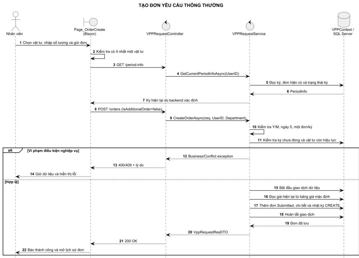
Hình 3-18: Sơ đồ tuần tự tạo đơn yêu cầu thông thường
