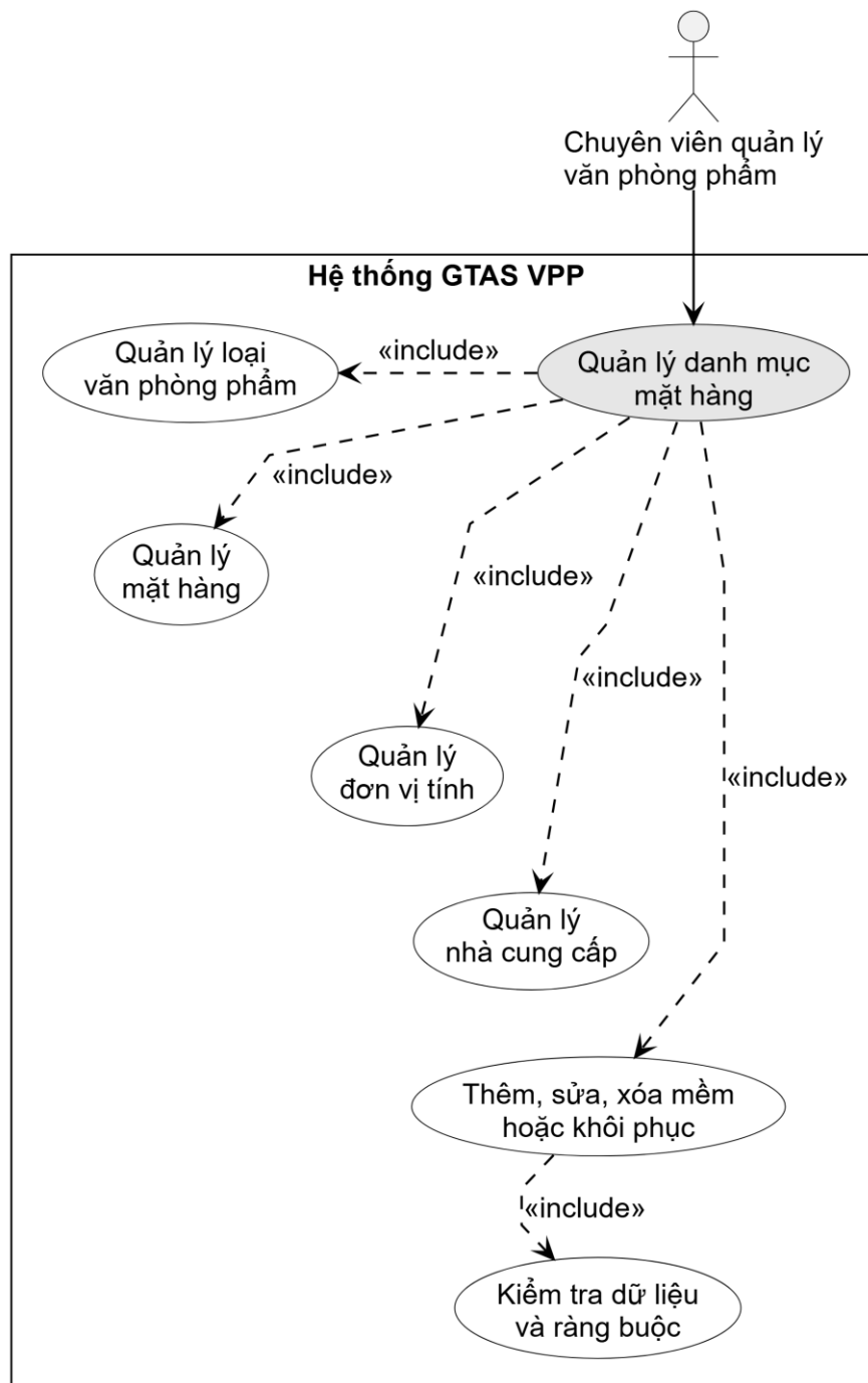
Hình 3-12: Use case quản lý danh mục văn phòng phẩm
