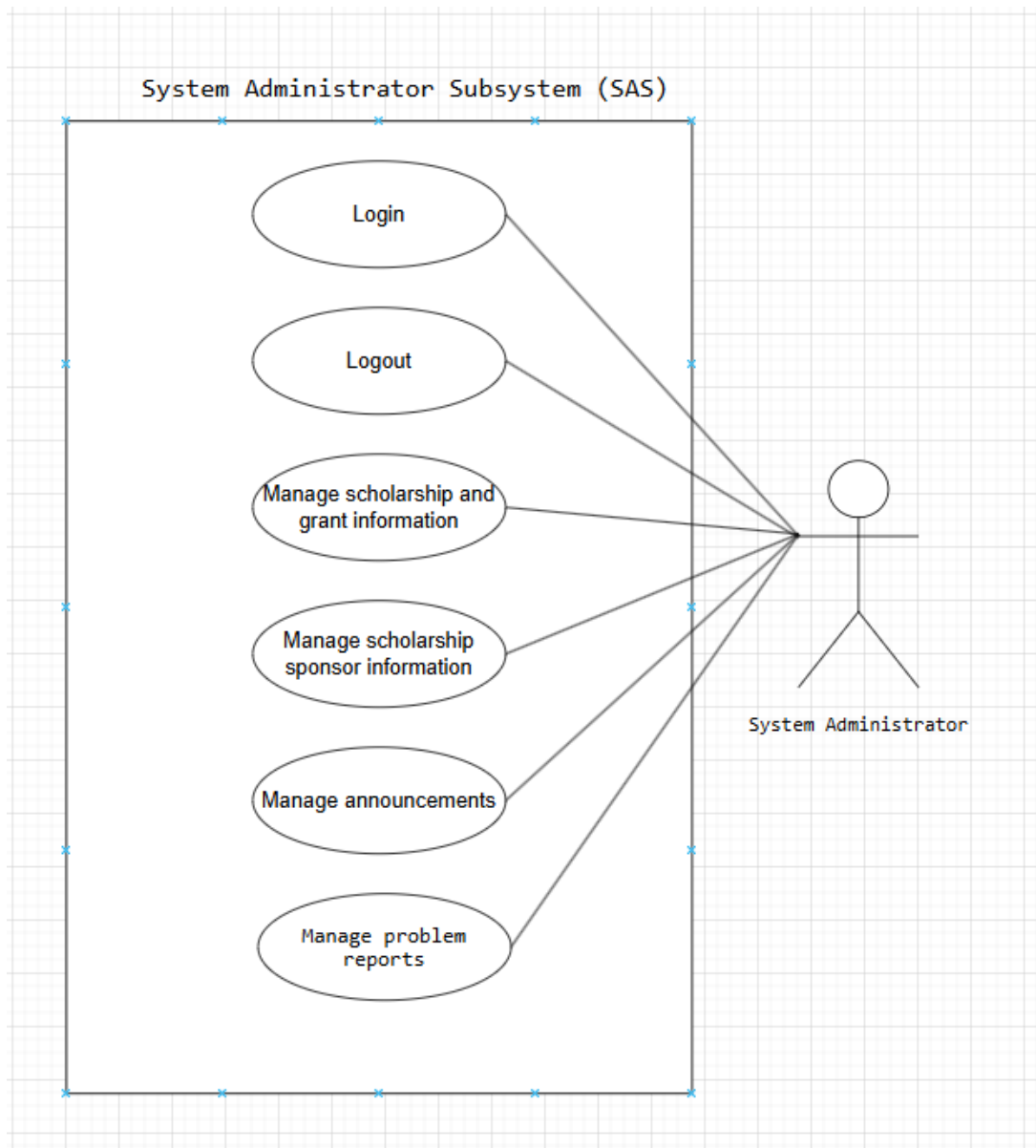
圖二 系統管理員 use case 概念圖
