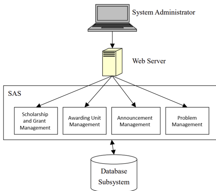
圖六 SAS 子系統架構圖
