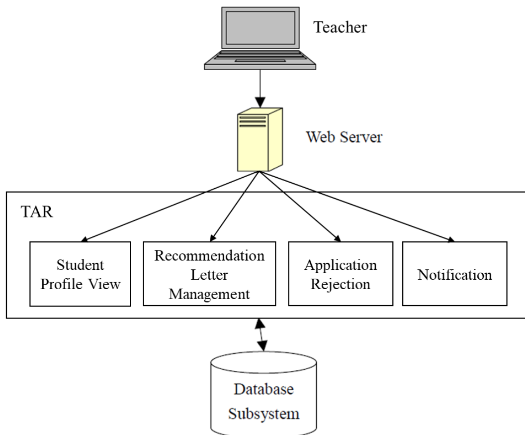
圖七 TAR 子系統架構圖
