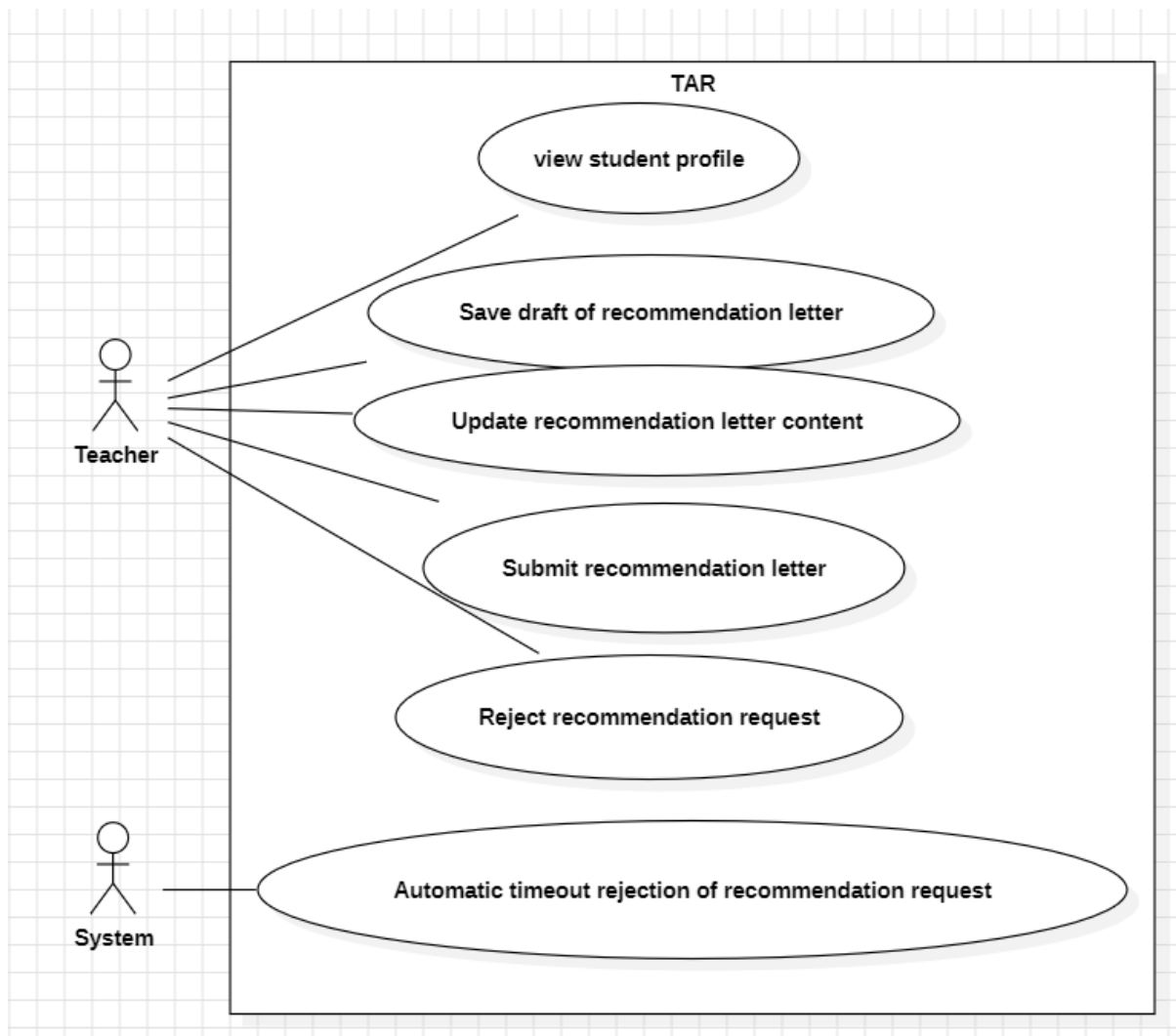
圖八 TAR Use Case Diagram
