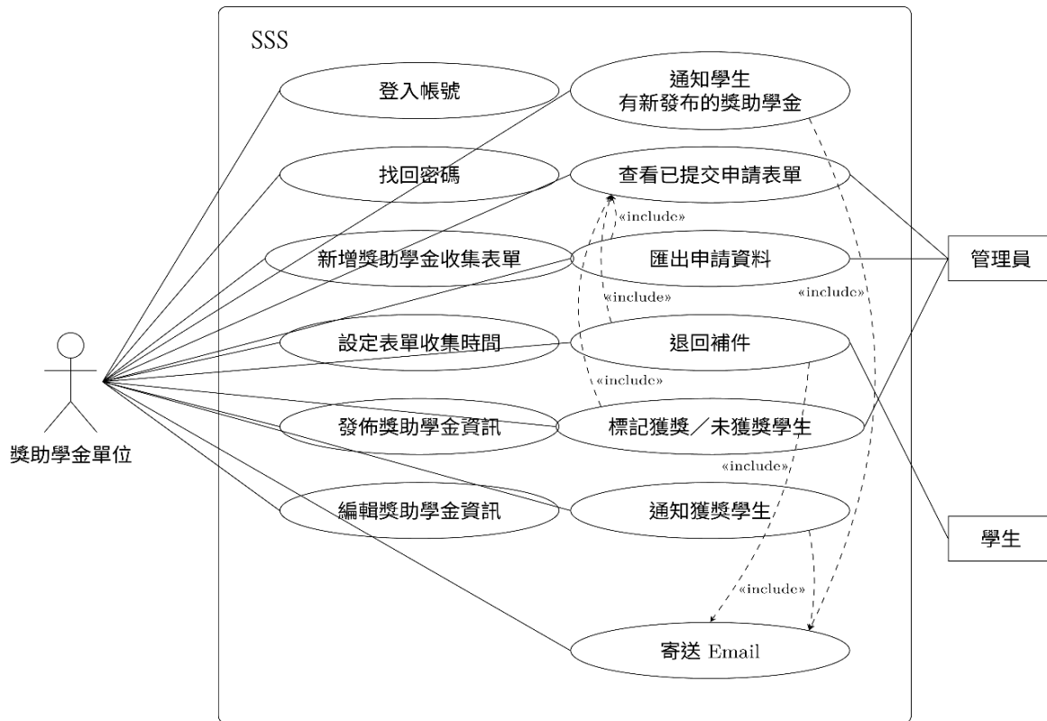
圖四 獎助單位 use case 概念圖
