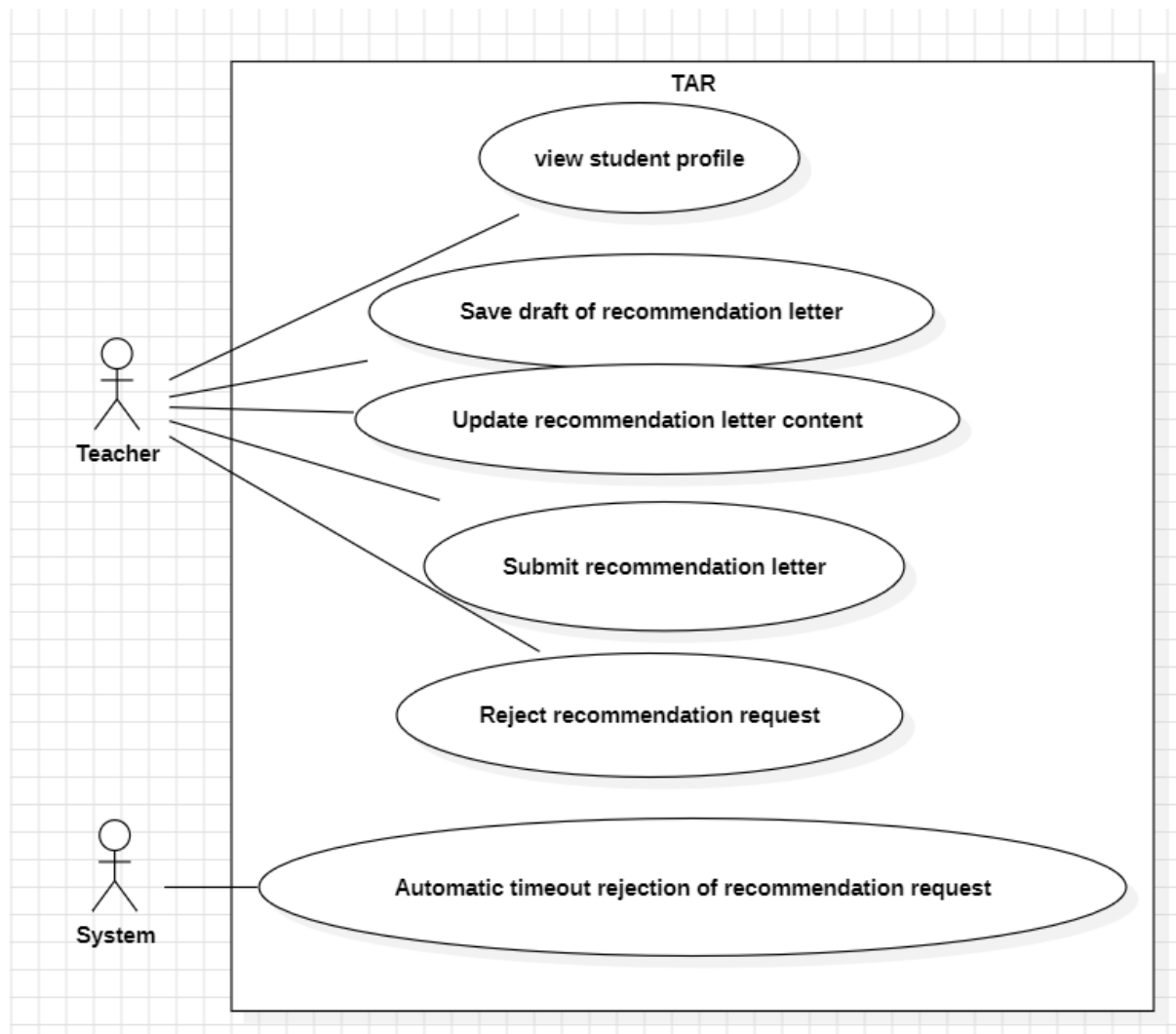
圖三 導師 use case 概念圖
