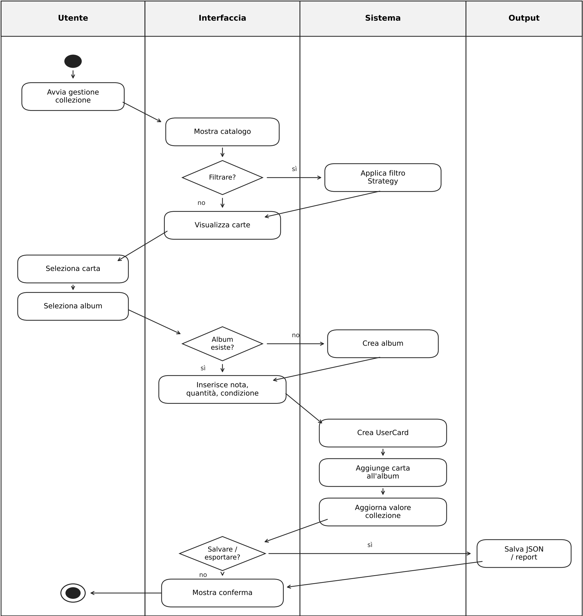
Activity Diagram - Aggiunta carta alla collezione
