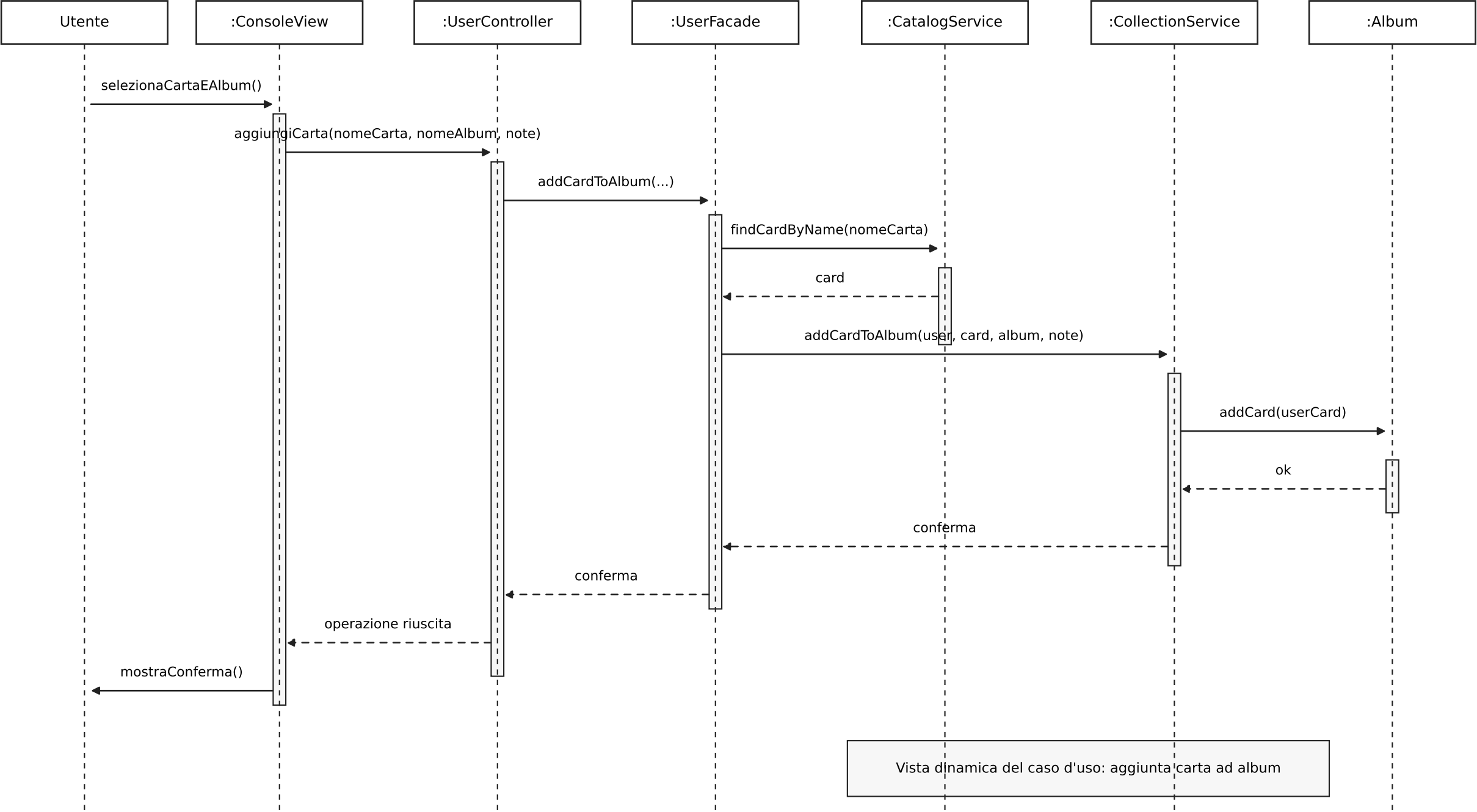
Sequence Diagram - Aggiunta carta ad album
