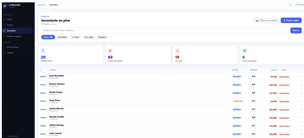
Figura 13. Inventario en piso, con filtros y acceso a escaneo de código de barras (RF06, RF03). Captura del prototipo.
