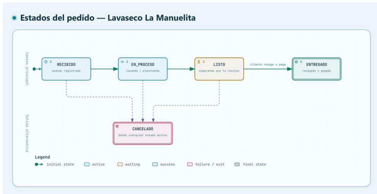
Figura 7. Diagrama de estados del pedido — Lavaseco La Manuelita. Elaboración propia.
