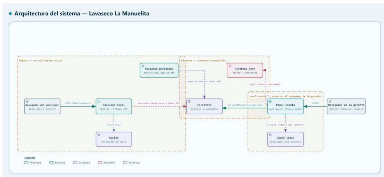
Figura 5. Arquitectura de despliegue local-first — Lavaseco La Manuelita. Elaboración propia.
