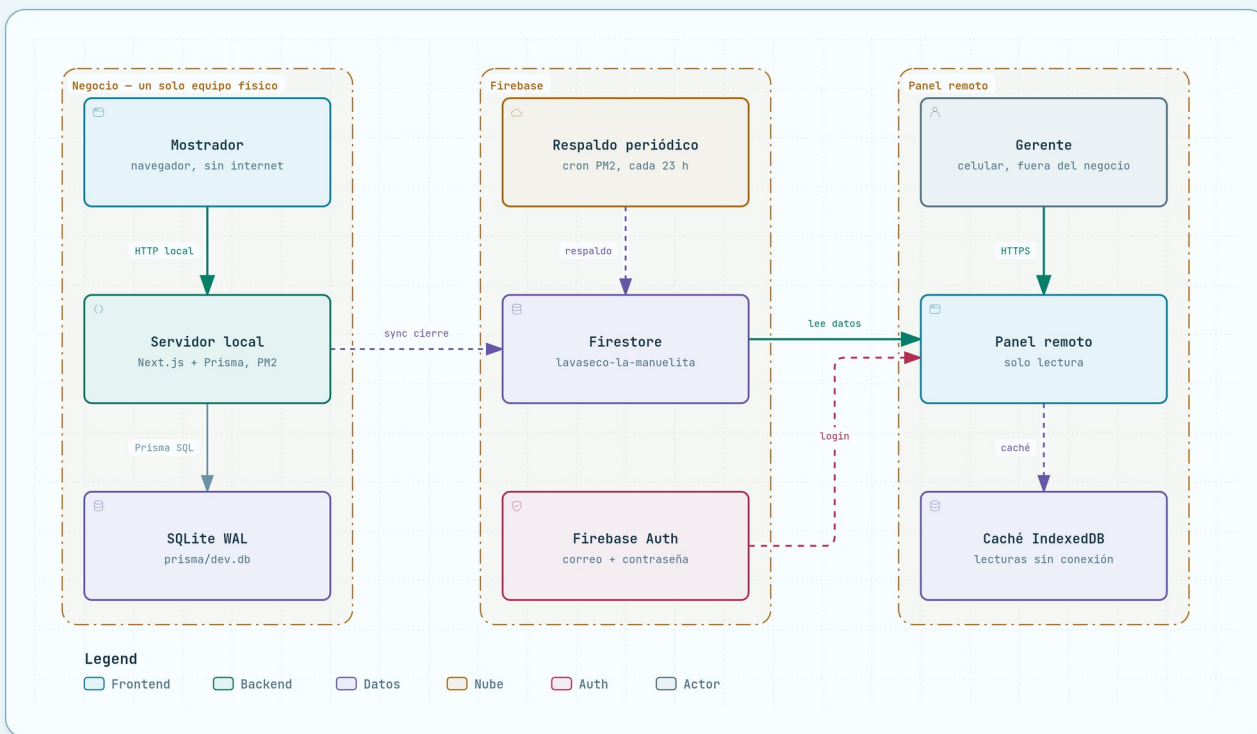
Figura 5. Arquitectura de despliegue local-first — Lavaseco La Manuelita. Elaboración propia.
