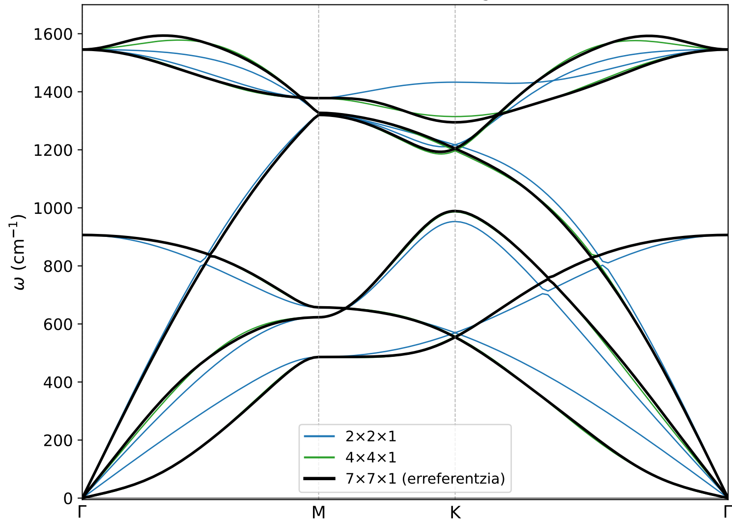
Grafenoa — DFPT konvergencia
