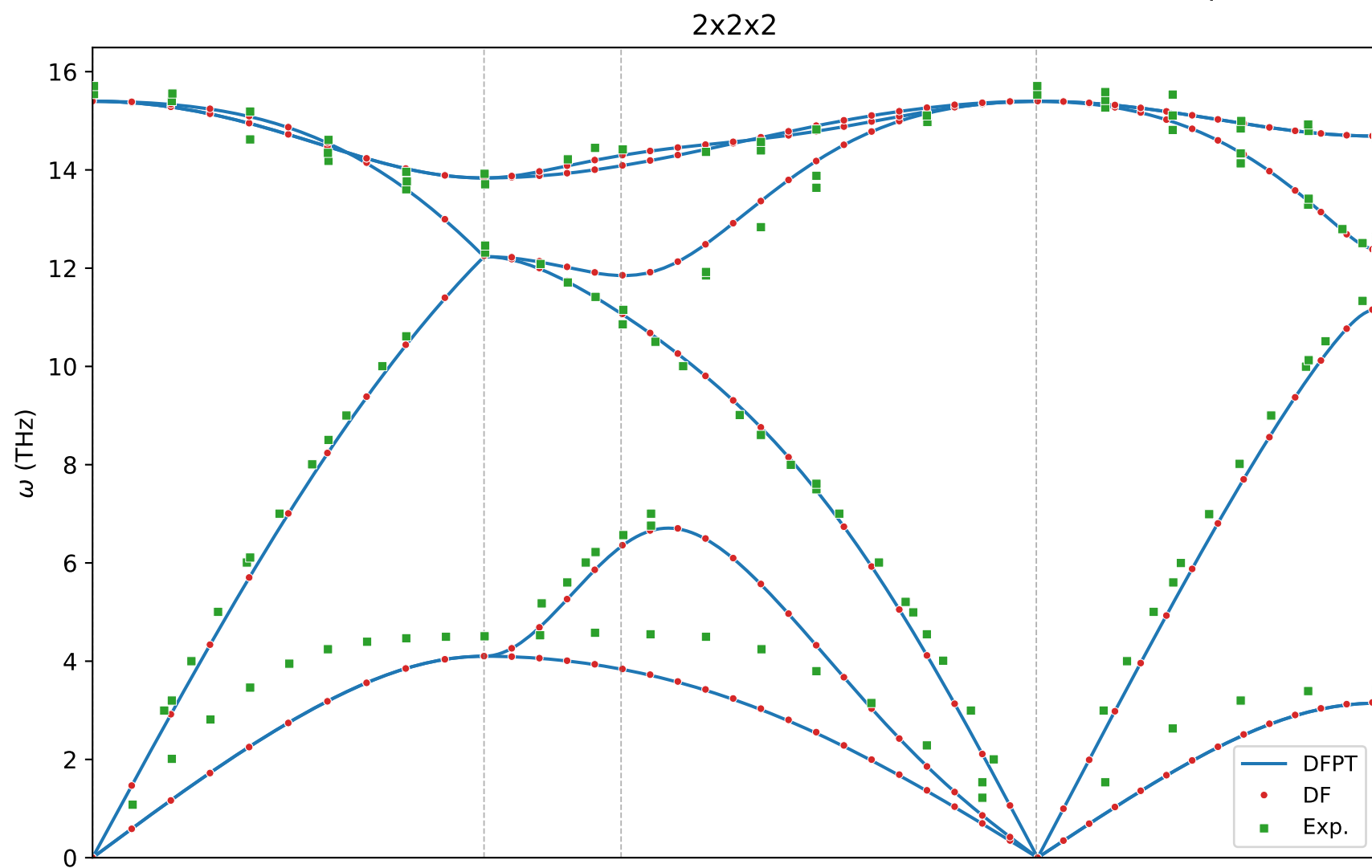
DF (puntos) vs DFPT (líneas) — Si
