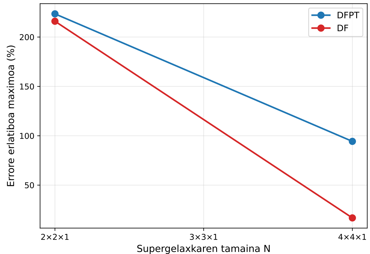
Konbergentzia: errore erlatiboa 6×6×1 erreferentziarekiko — Grafenoa
