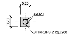
V1 SCALE 1:20
