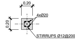
V1 SCALE 1:20
