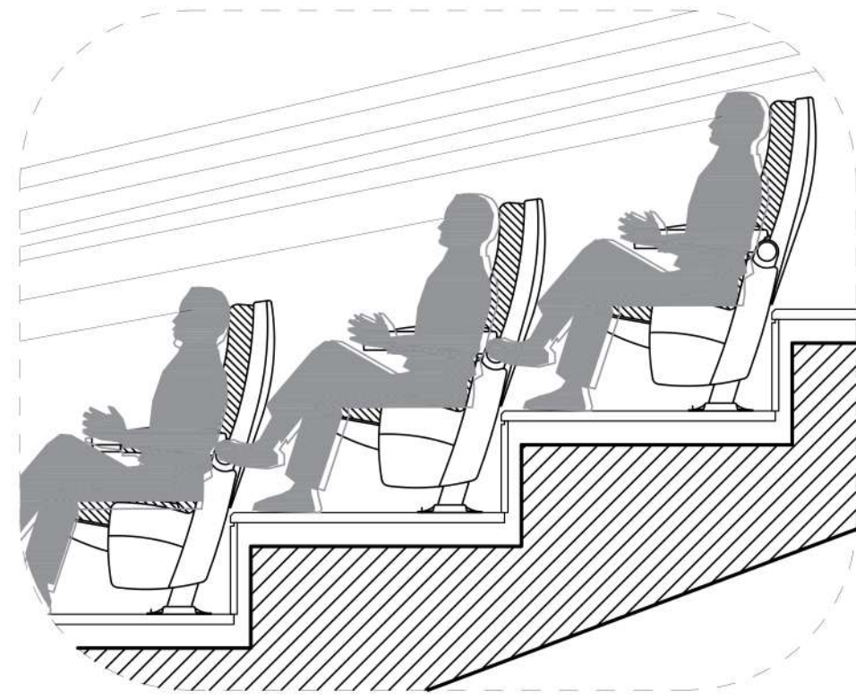
D01 COUPE-01 L'ÉCHAPPÉ VISUELLE DANS LE PETIT AUDITORIUM
