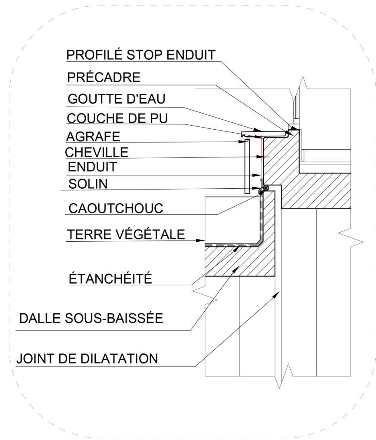
D02 COUPE LE JOINT DE DILATATION ET DALLE SOUS-BAISSÉE
