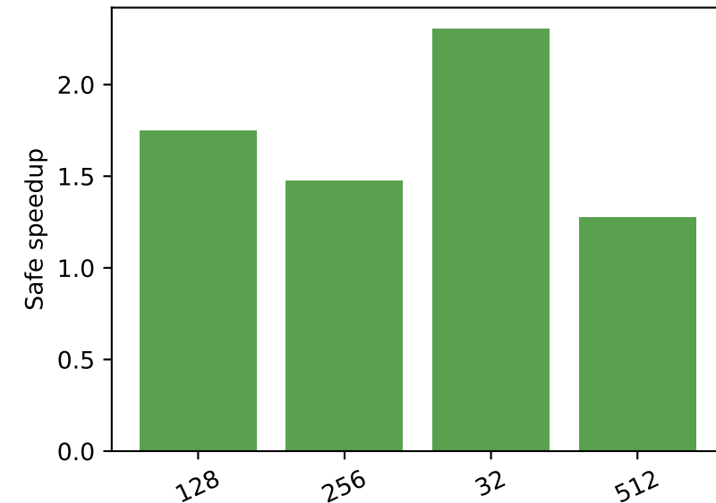
Tokens
