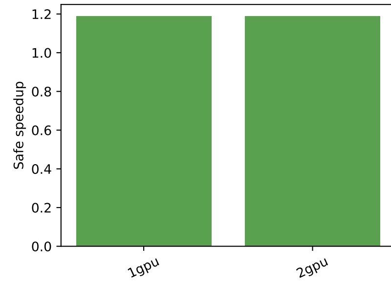
EP
