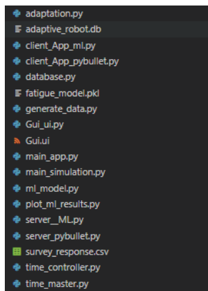
Рисунок 10 – Структура проекта
