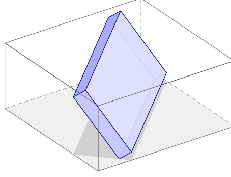
Рис. 1: Коробка 2,8 \times 1,3 \times 0,25 в ящике высоты 1,2 с полом 2,7 \times 2,64 в положении, которое описывает одна из проверок критерия: длинное ребро горизонтально, грань 1,3 \times 0,25 наклонена в вертикальной полосе, а ортогональная проекция коробки на пол (тень) — прямоугольник 2,8 \times h^* , повёрнутый на полу. Поворот вычислен как в доказательстве предложения 4.1.
