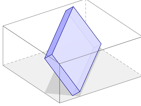
Рис. 1: Коробка 2,8 \times 1,3 \times 0,25 в ящике высоты 1,2 с полом 2,7 \times 2,64 в положении, которое описывает одна из проверок критерия: длинное ребро горизонтально, грань 1,3 \times 0,25 наклонена в вертикальной полосе, а ортогональная проекция коробки на пол (тень) — прямоугольник 2,8 \times h^* , повёрнутый на полу. Поворот вычислен как в доказательстве предложения 4.1.
