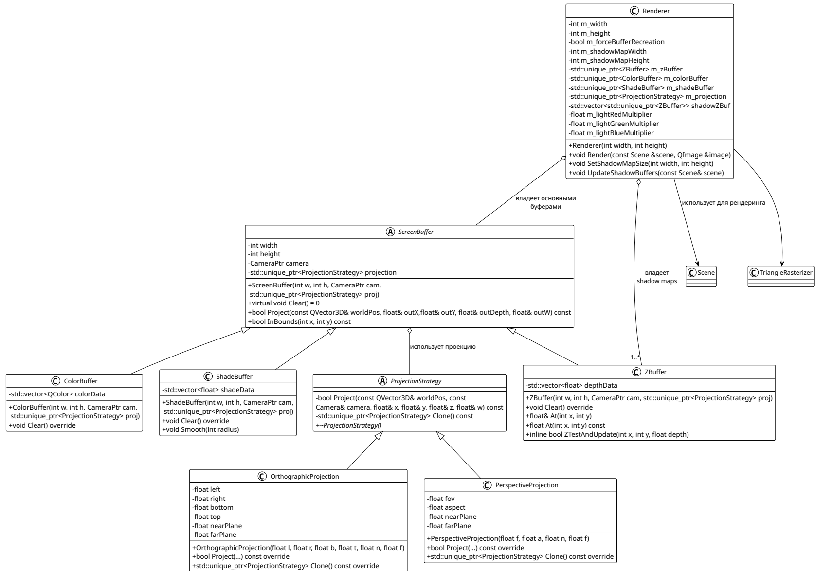
Рисунок 2 — Диаграмма классов домена отрисовки, ч. 1
