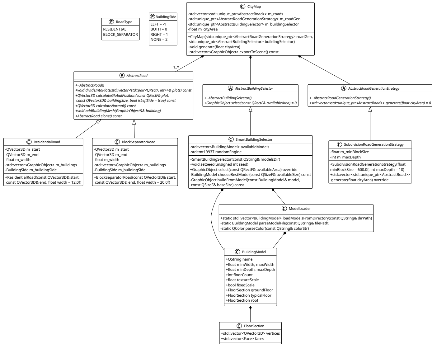
Рисунок 1 — Диаграмма классов домена генерации городской среды
