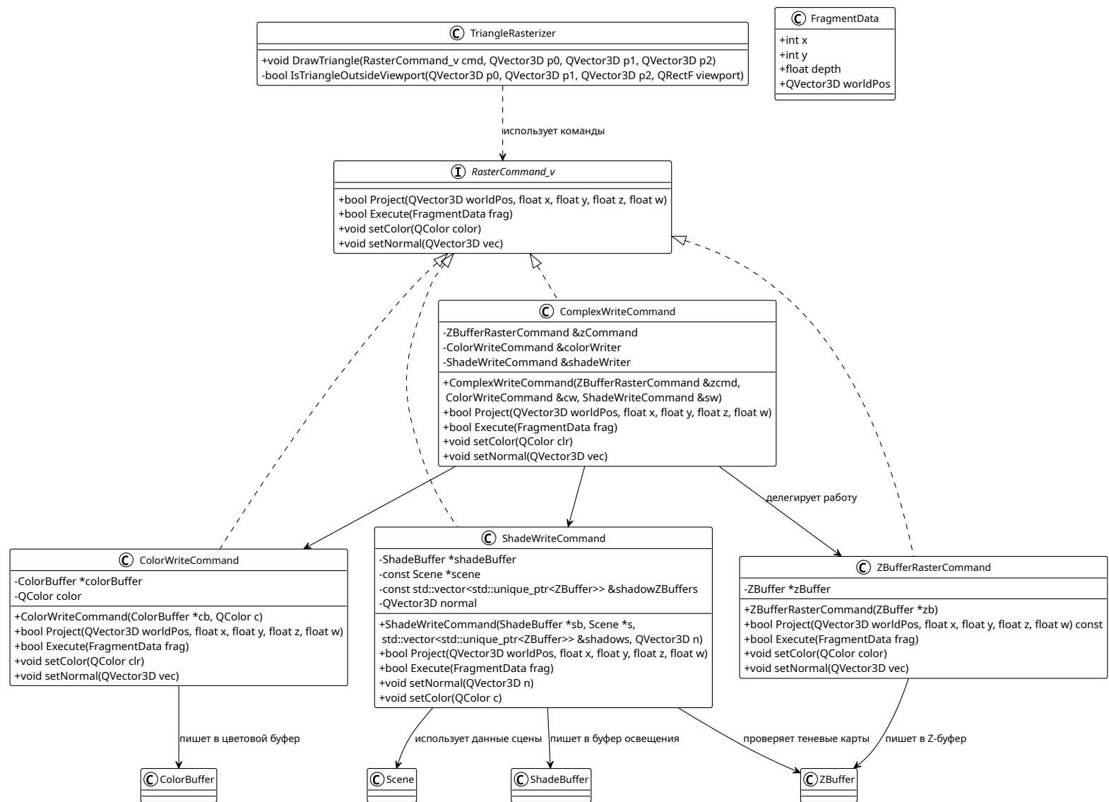
Рисунок 3 — Диаграмма классов домена отрисовки, ч. 2
