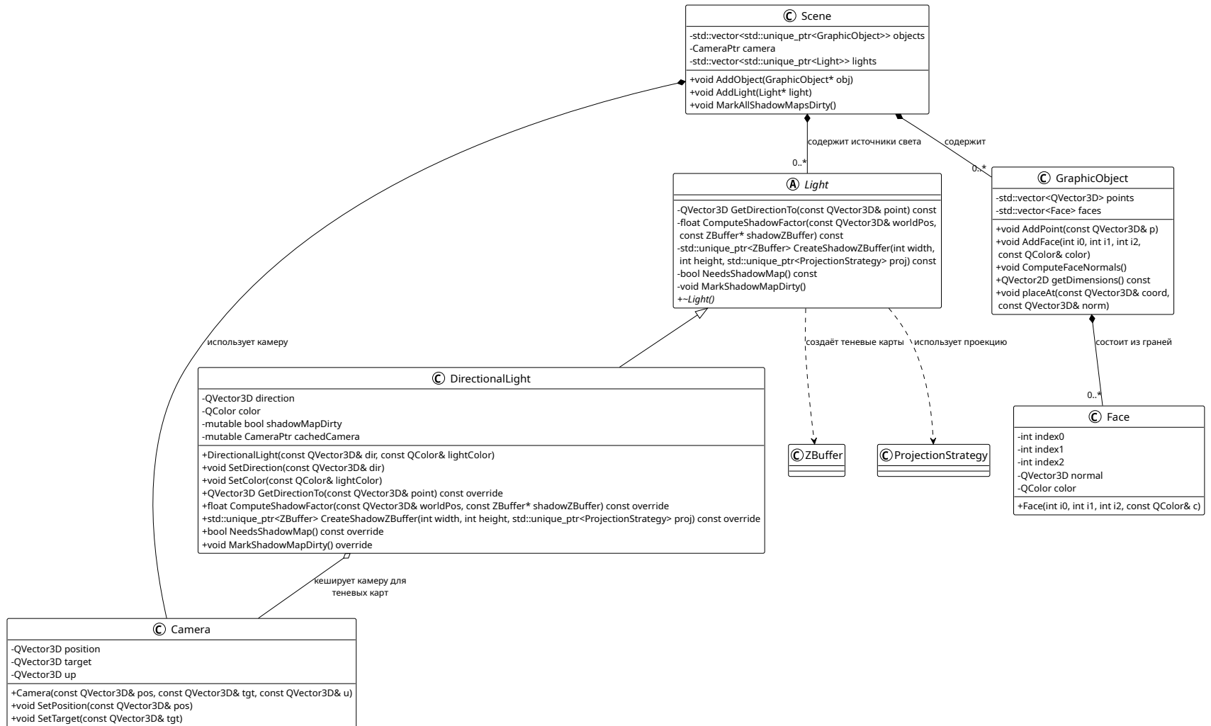
Рисунок 4 — Диаграмма классов домена отрисовки, ч. 3
