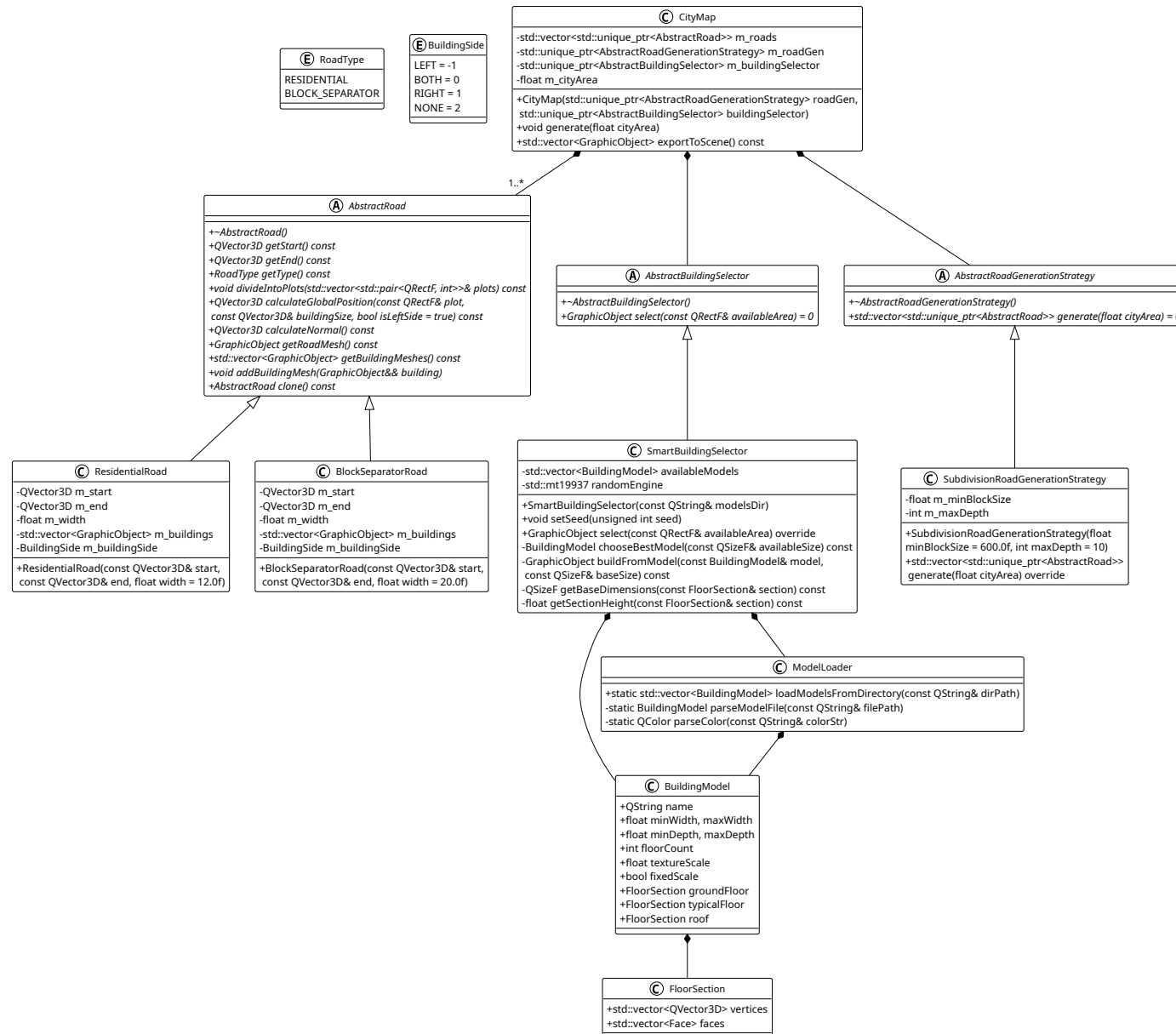
Рисунок 1 — Диаграмма классов домена генерации городской среды
