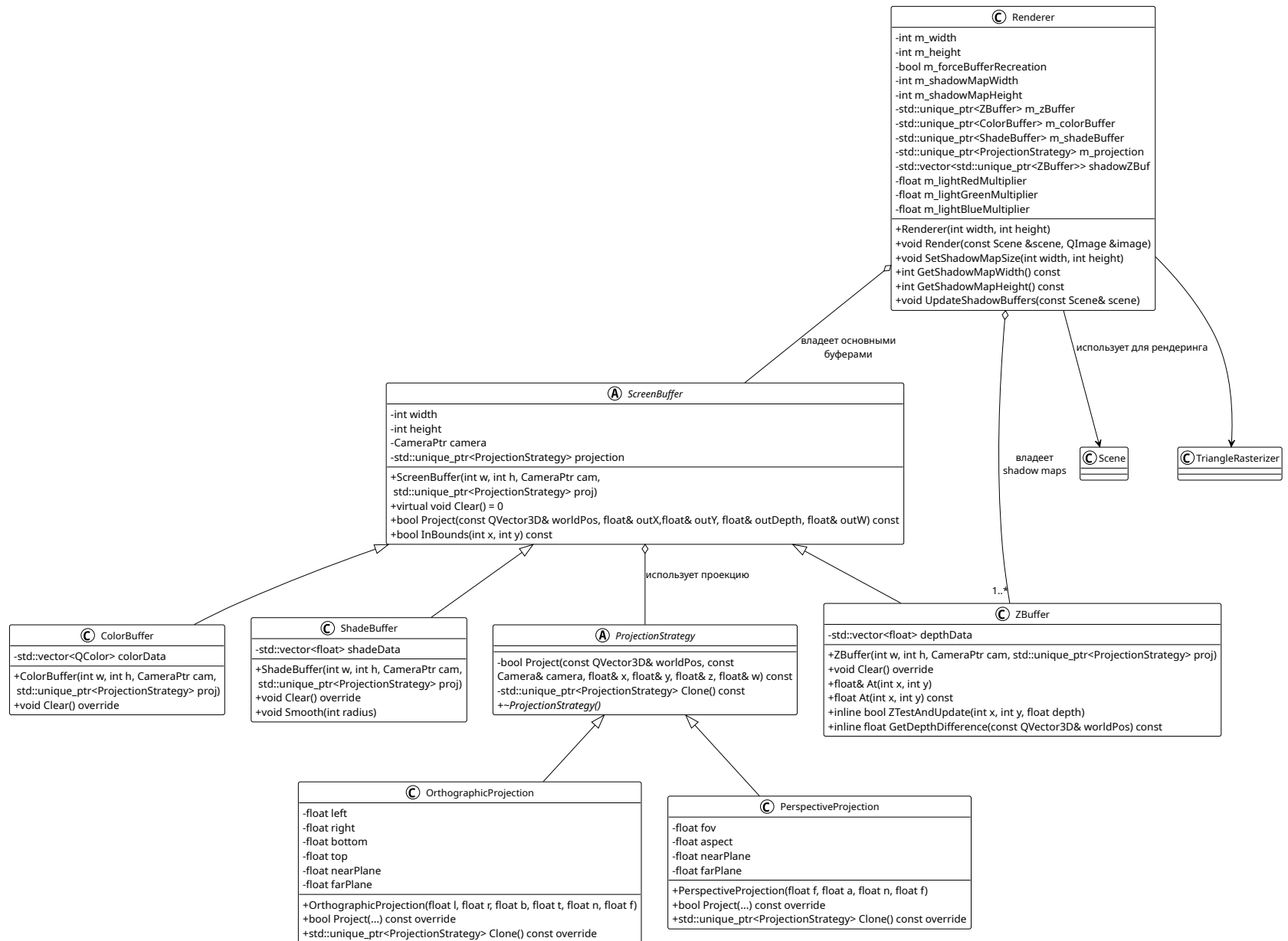
Рисунок 2 — Диаграмма классов домена отрисовки, ч. 1
