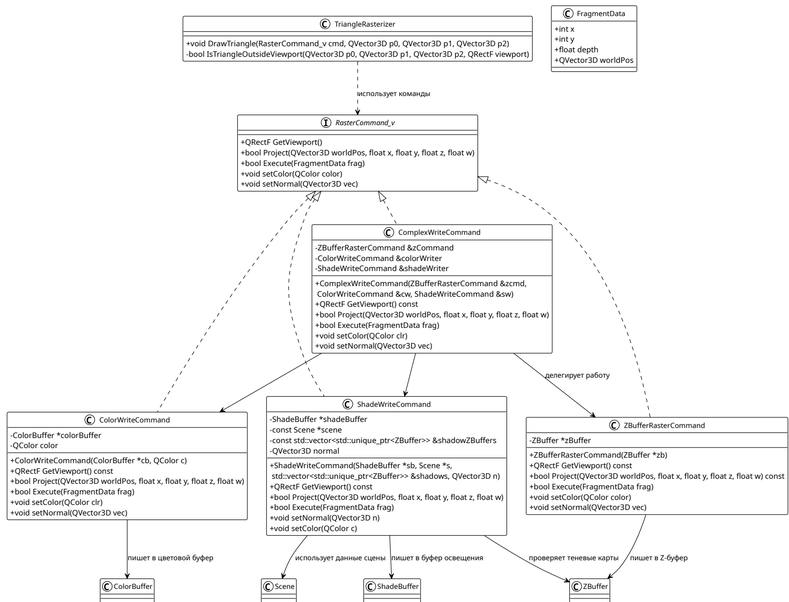
Рисунок 3 — Диаграмма классов домена отрисовки, ч. 2
