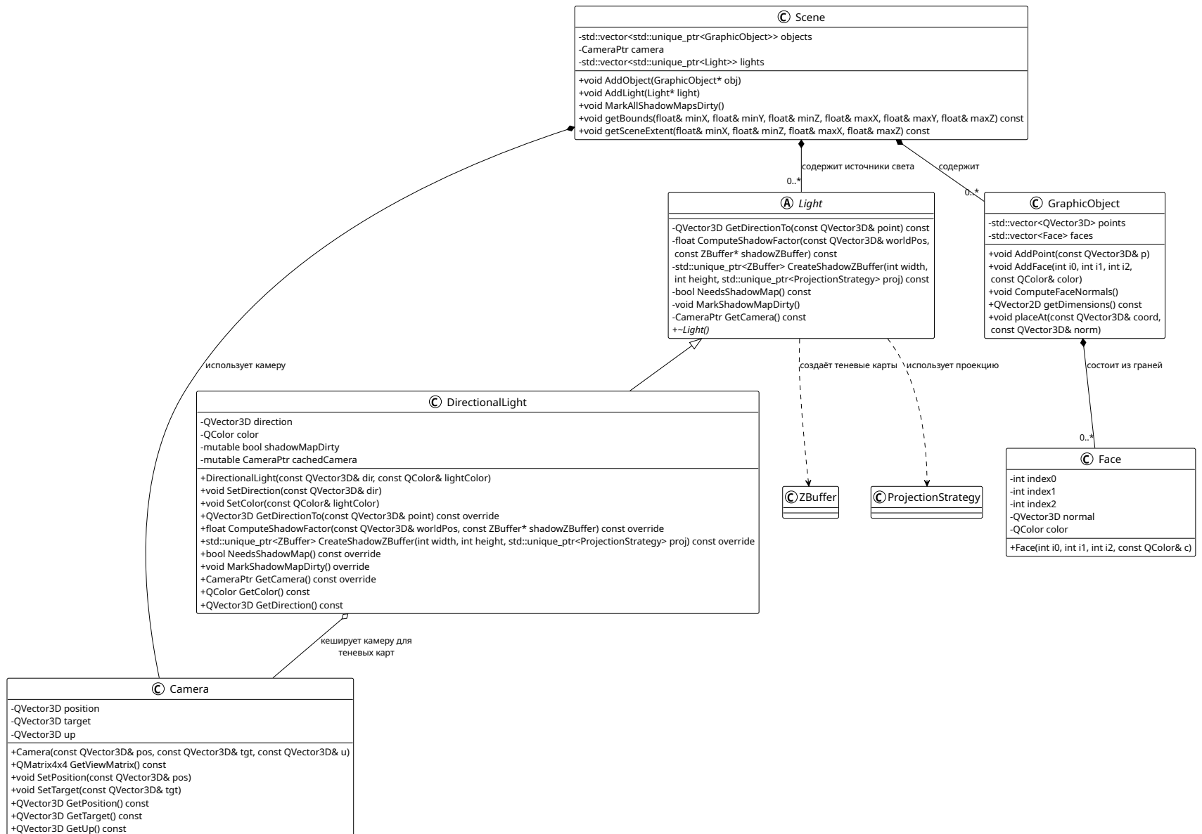
Рисунок 4 — Диаграмма классов домена отрисовки, ч. 3
