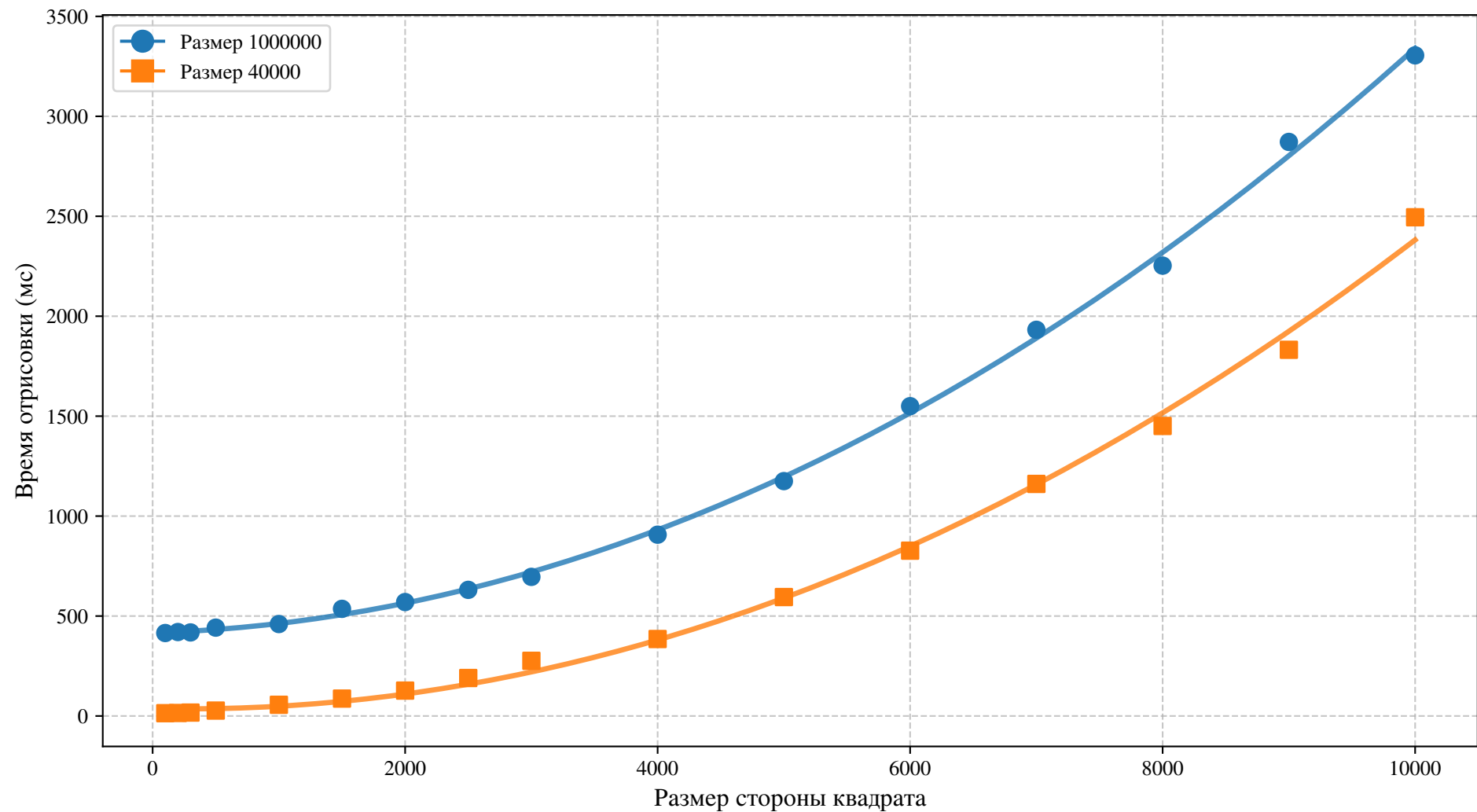
Время отрисовки квадратного кадра в зависимости от размера стороны
