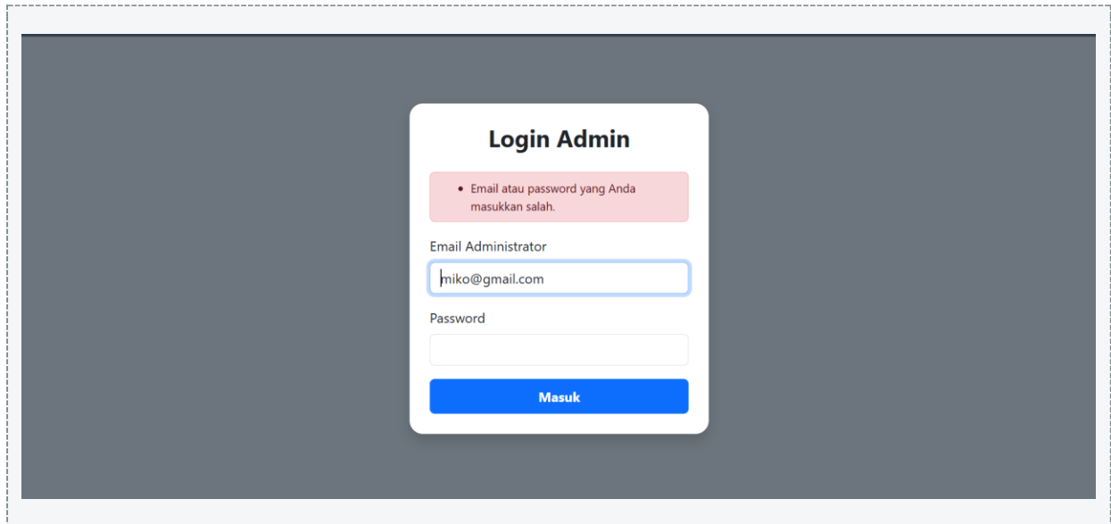
Gambar 2. Halaman Login
