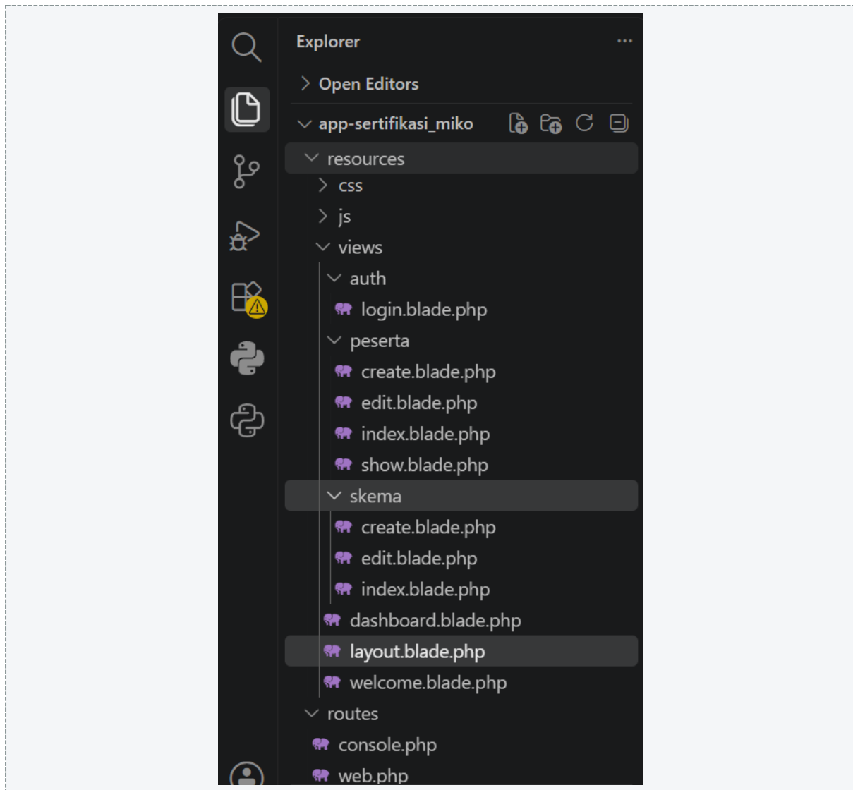
Gambar 13. Struktur Project
