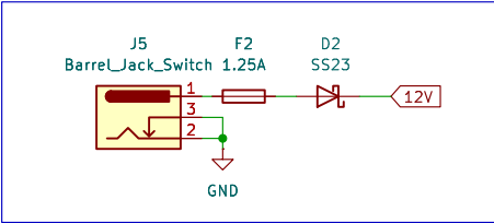
12V DC Input
