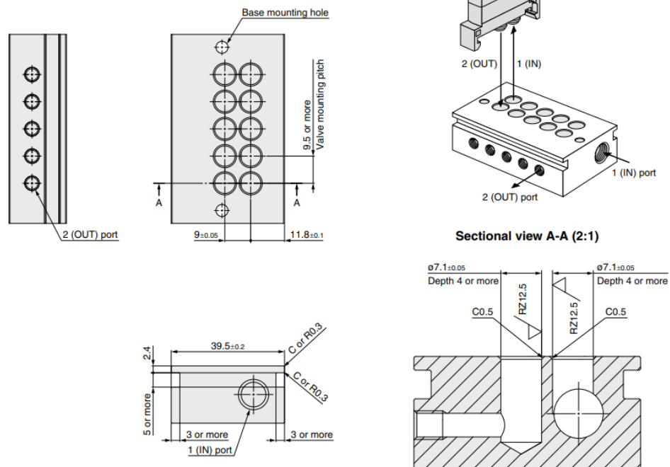
Rys. 21. Zalecenia dotyczące płyty montażowej dla zaworów z serii SX10 w konfiguracji szybkozłącznej firmy SMC [25].
