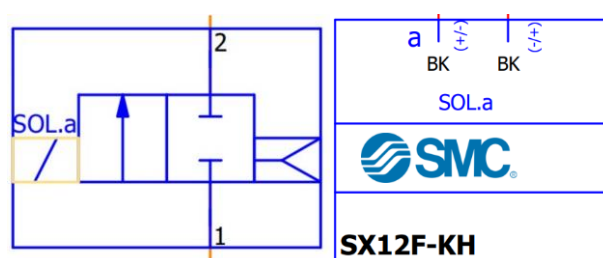
Rys. 19. Schemat zaworu z serii SX10.
