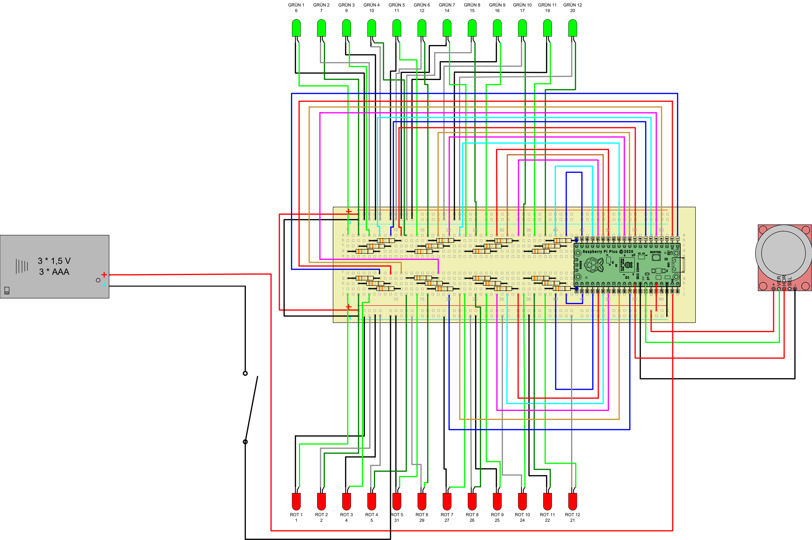
Schaltplan mit Widerständen auf der Platine
