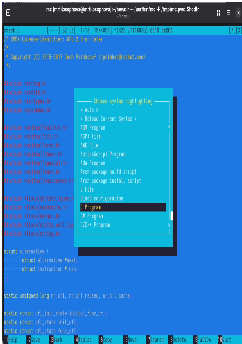
Рисунок 2.34: Цветовыделение синтаксиса
