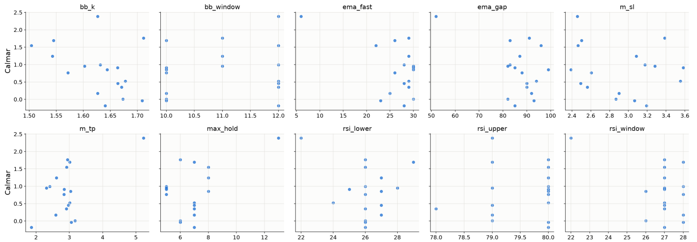
Slice plots: Calmar vs. cada parámetro (trials válidos)
