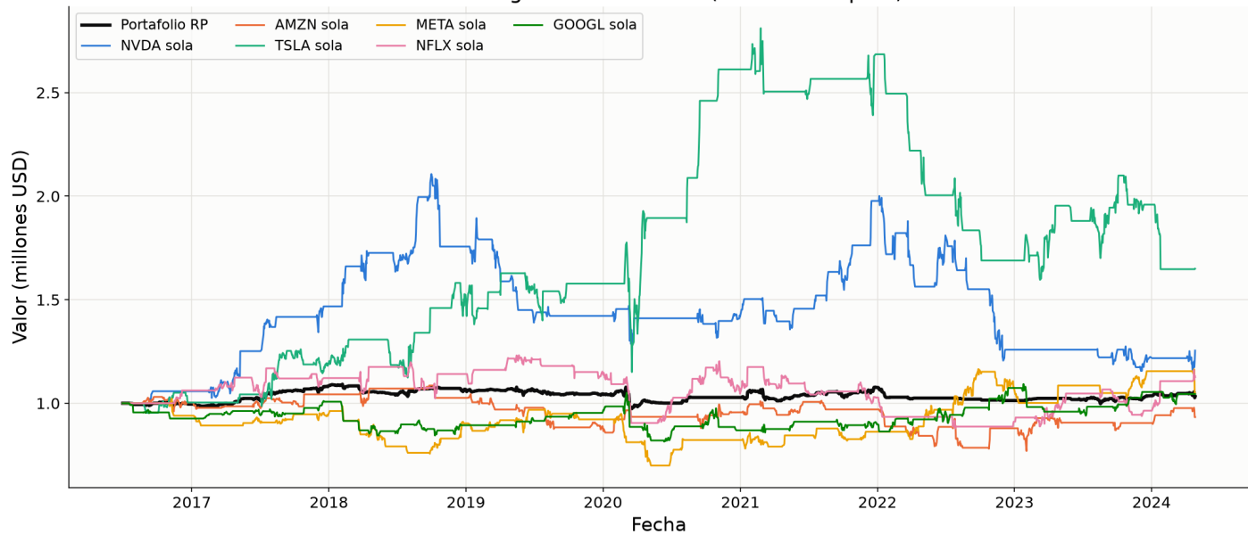
Portafolio vs. estrategia en cada activo (100% del capital) — WF-OOS
