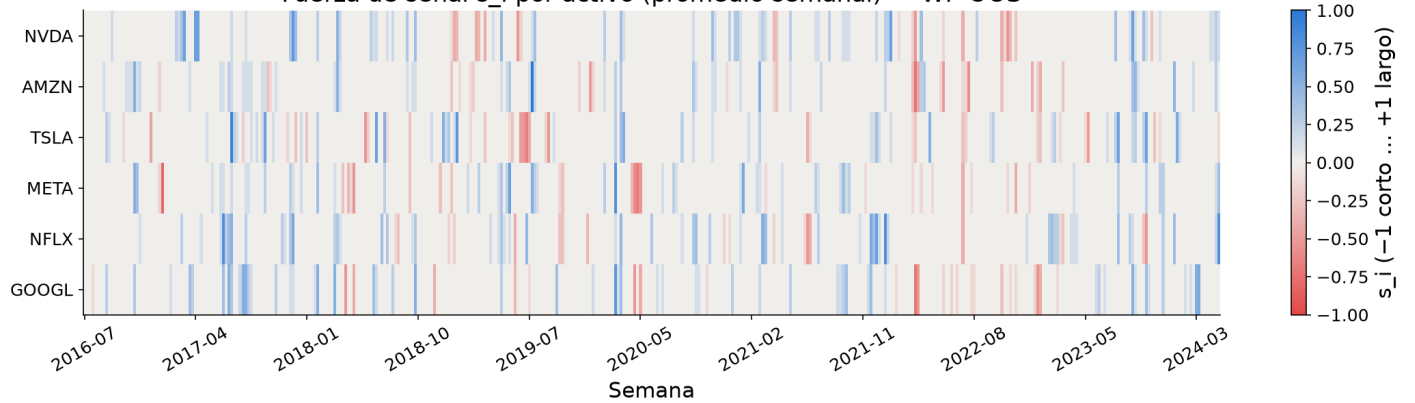
Fuerza de señal s_i por activo (promedio semanal) — WF-OOS
