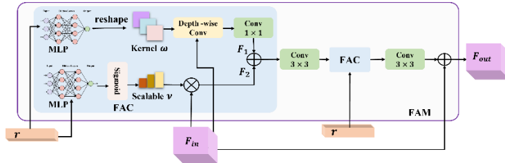
(b) 特征调整模块结构图
