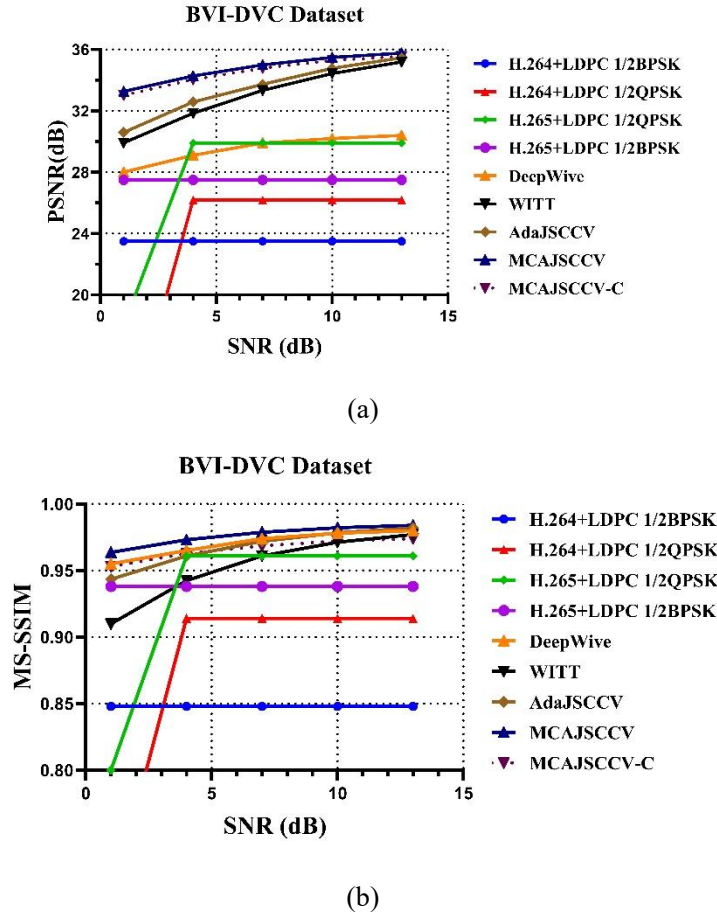
图 5-4 在 AWGN 信道下， \text{CBR} = 0.031 时，MCAJSCCV 在 BVI-DVC 数据集上测得的失真性能随信噪比变化曲线图
