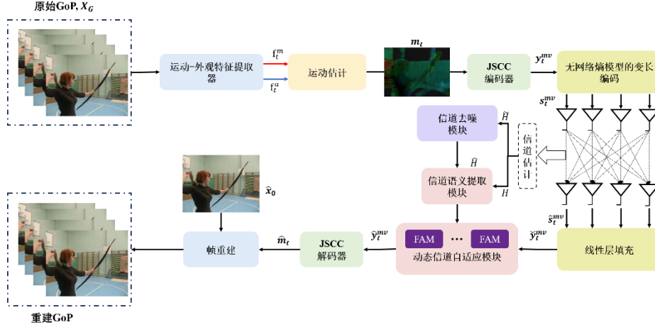
图 4-1 SAWV-MIMO 架构图
