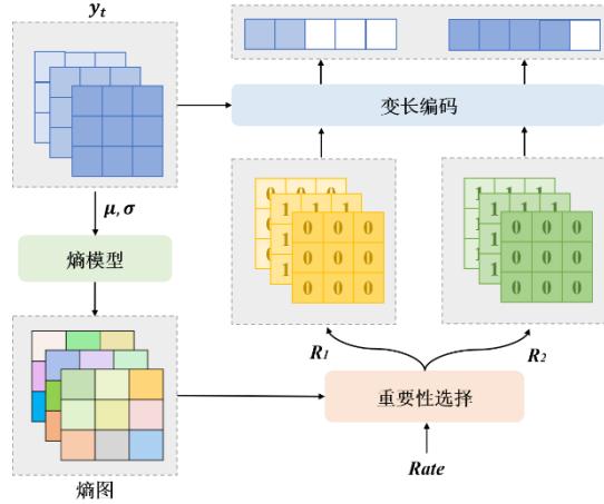
图 3-3 变长编码模块结构图
