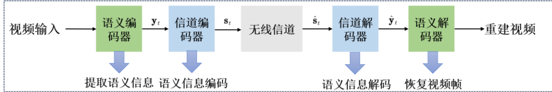
图 2-3 视频语义通信架构图
