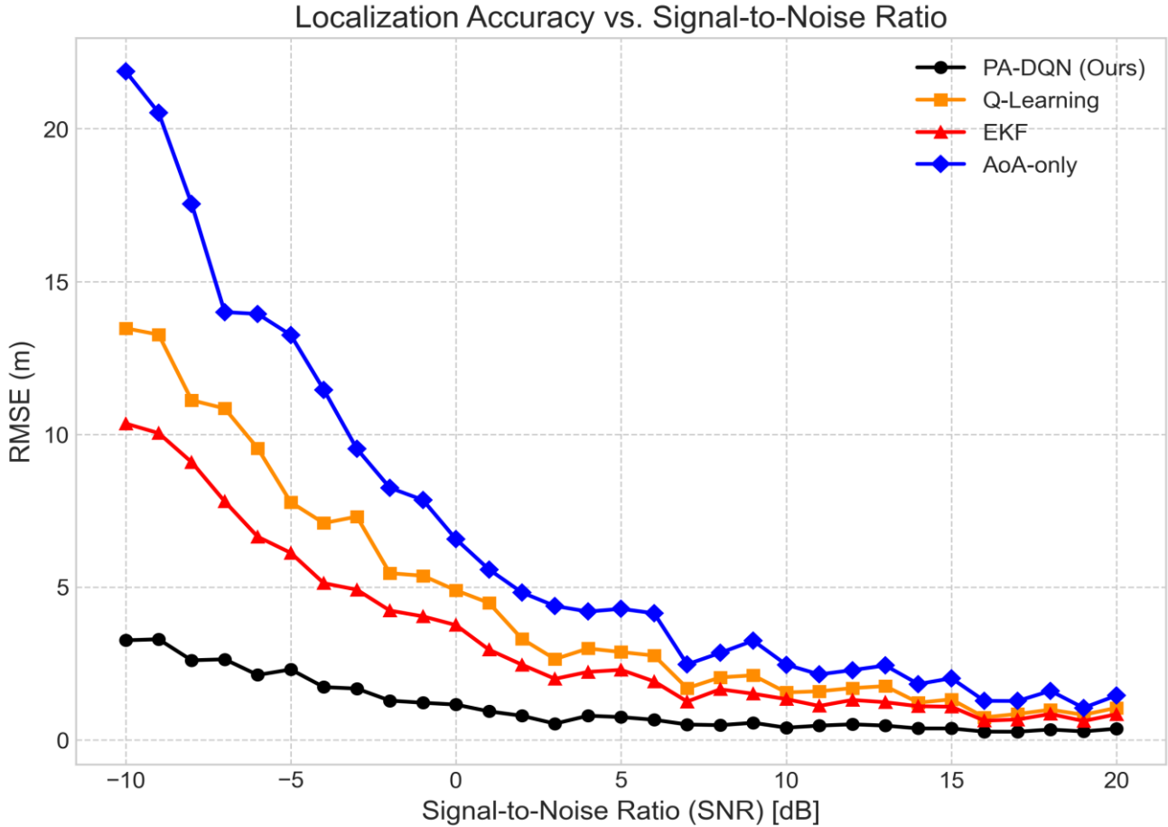
不同 SNR 条件下误差变化
