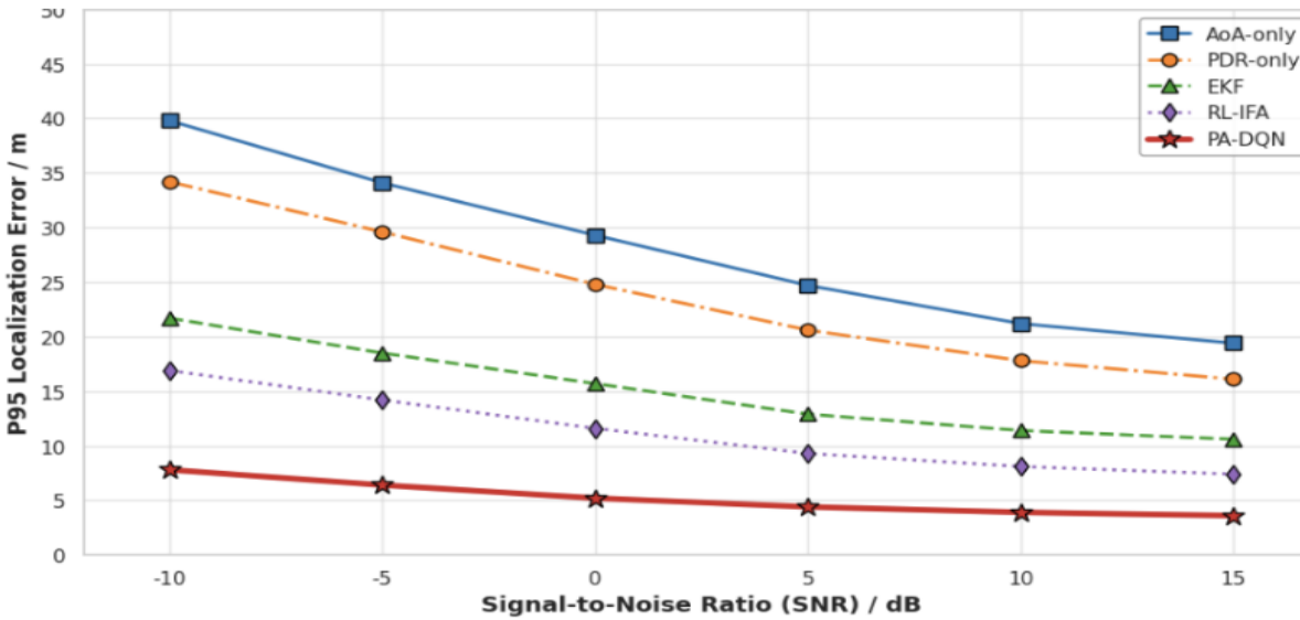
图 3-15 不同算法在多种信噪比条件下的 P95 对比曲线
