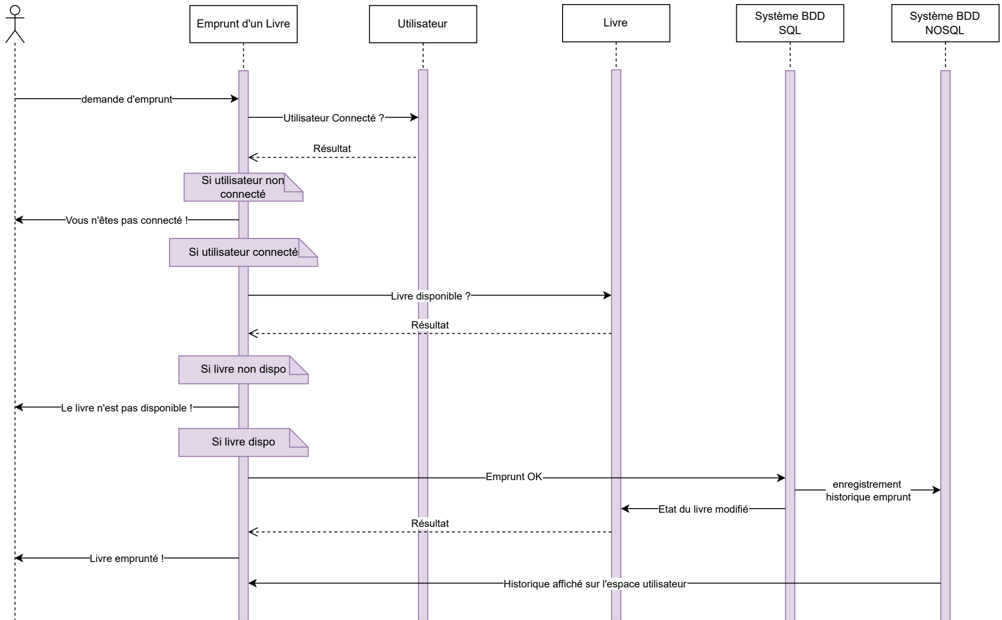
DIAGRAMME DE SEQUENCE - BIBLIOAPP EMPRUNT D'UN LIVRE
