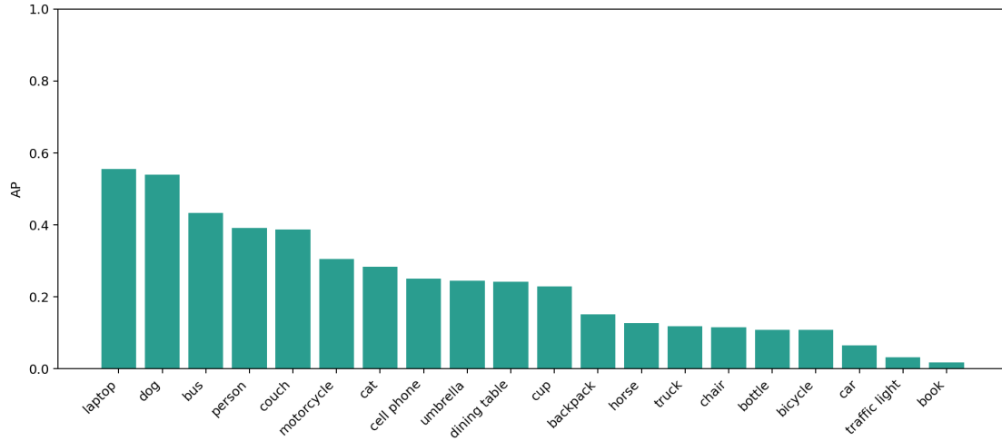
图 2: 改进方法每类 AP
