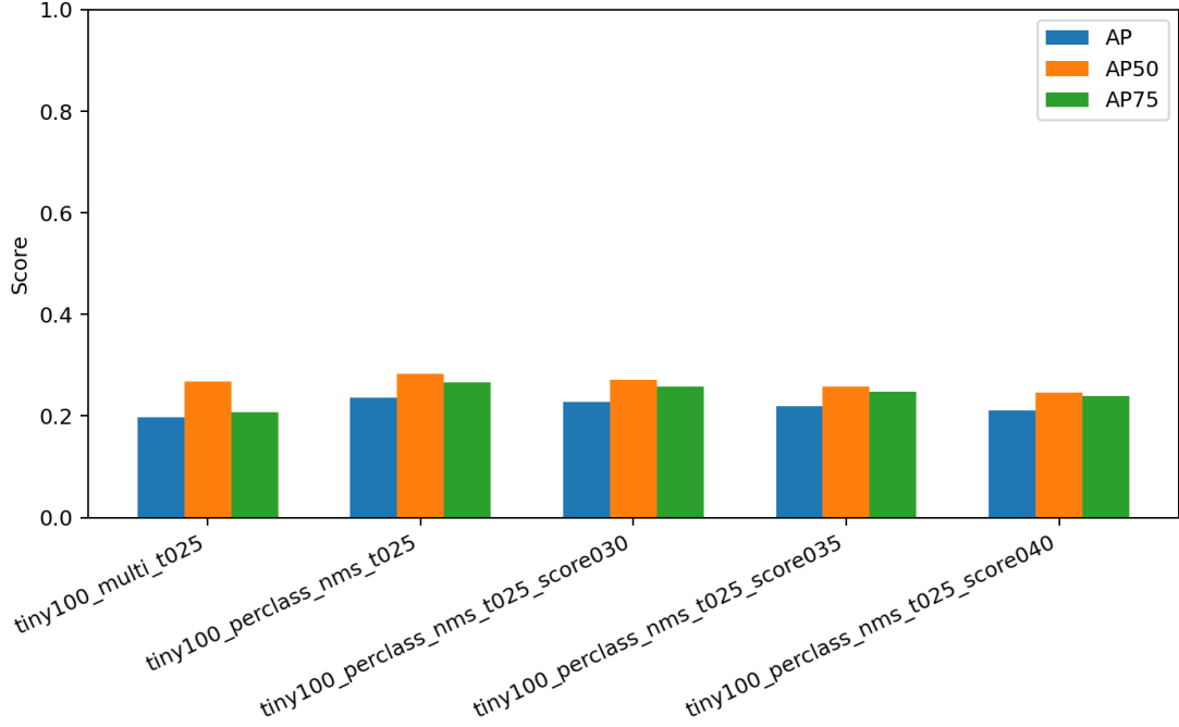
图 1: 100 张 COCO 子集实验对比
