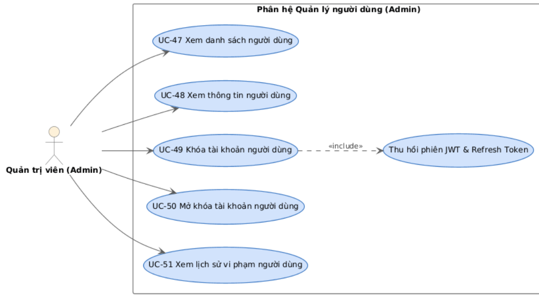
Hình 2.12: Sơ đồ Use Case Nhóm 10 - Quản lý người dùng Admin (UC-47 đến UC-51)
