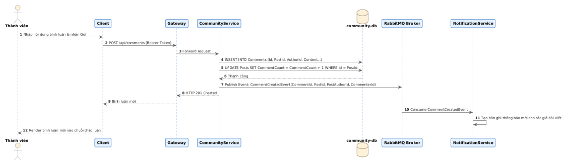
Hình 3.6.b: Biểu đồ Tuần tự (Sequence Diagram) Tiến trình Bình luận & Trả lời bình luận
