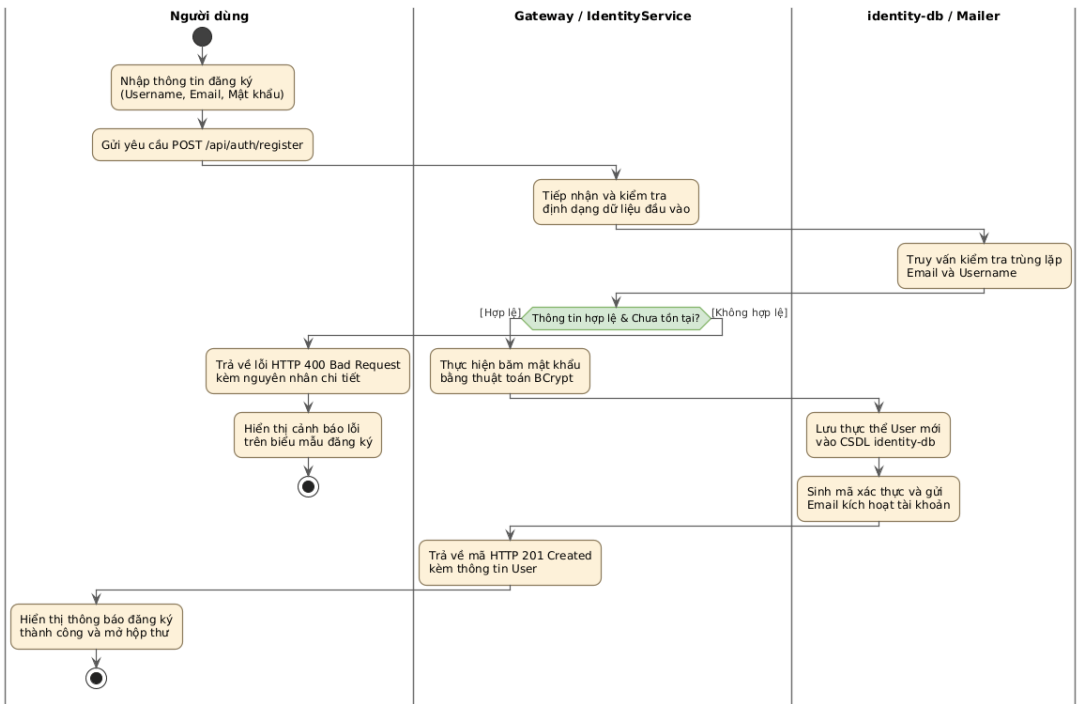
Hình 3.1.a: Biểu đồ Hoạt động (Activity Diagram) Tiến trình Đăng ký tài khoản
