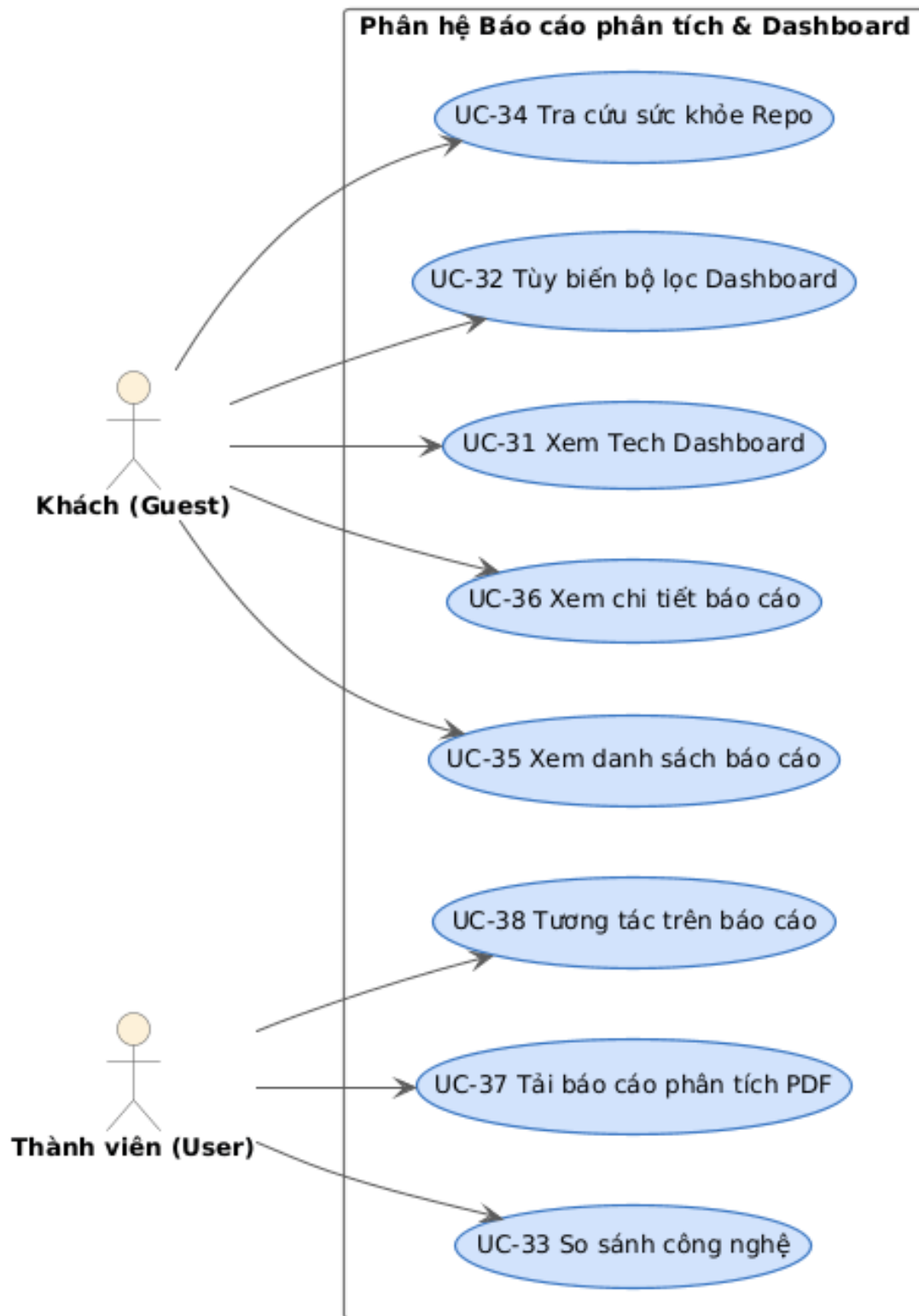
Hình 2.8: Sơ đồ Use Case Nhóm 6 - Báo cáo phân tích & Dashboard (UC-31 đến UC-38)
