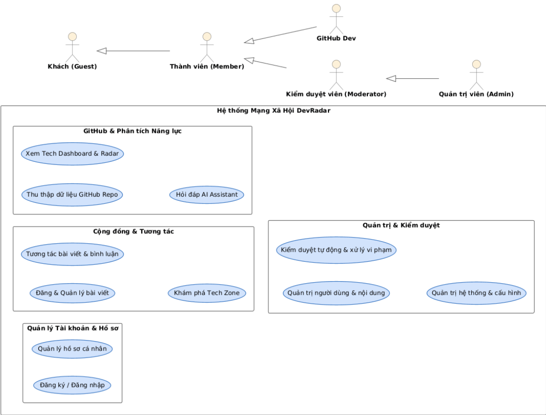
Hình 2.2: Sơ đồ Use Case Tổng quát Hệ thống DevRadar
