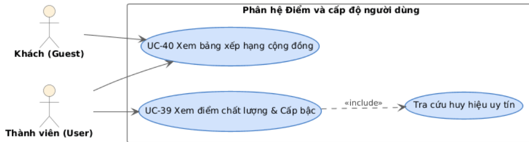
Hình 2.9: Sơ đồ Use Case Nhóm 7 - Điểm và cấp độ người dùng (UC-39, UC-40)
