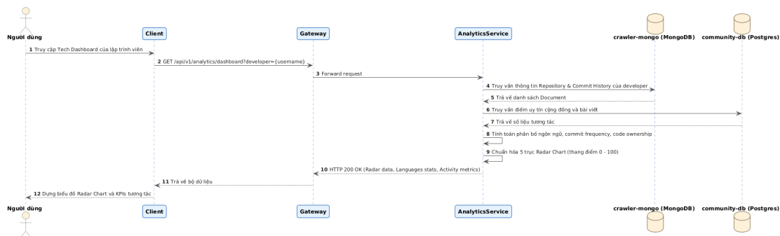
Hình 3.10.b: Biểu đồ Tuần tự (Sequence Diagram) Tiến trình Tra cứu Tech Dashboard & Radar Chart
