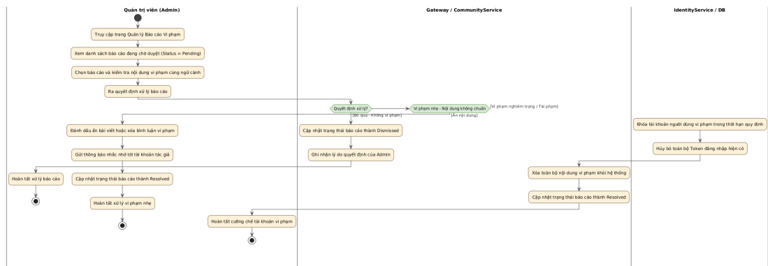
Hình 3.14.a: Biểu đồ Hoạt động (Activity Diagram) Tiến trình Admin Xử lý báo cáo vi phạm
