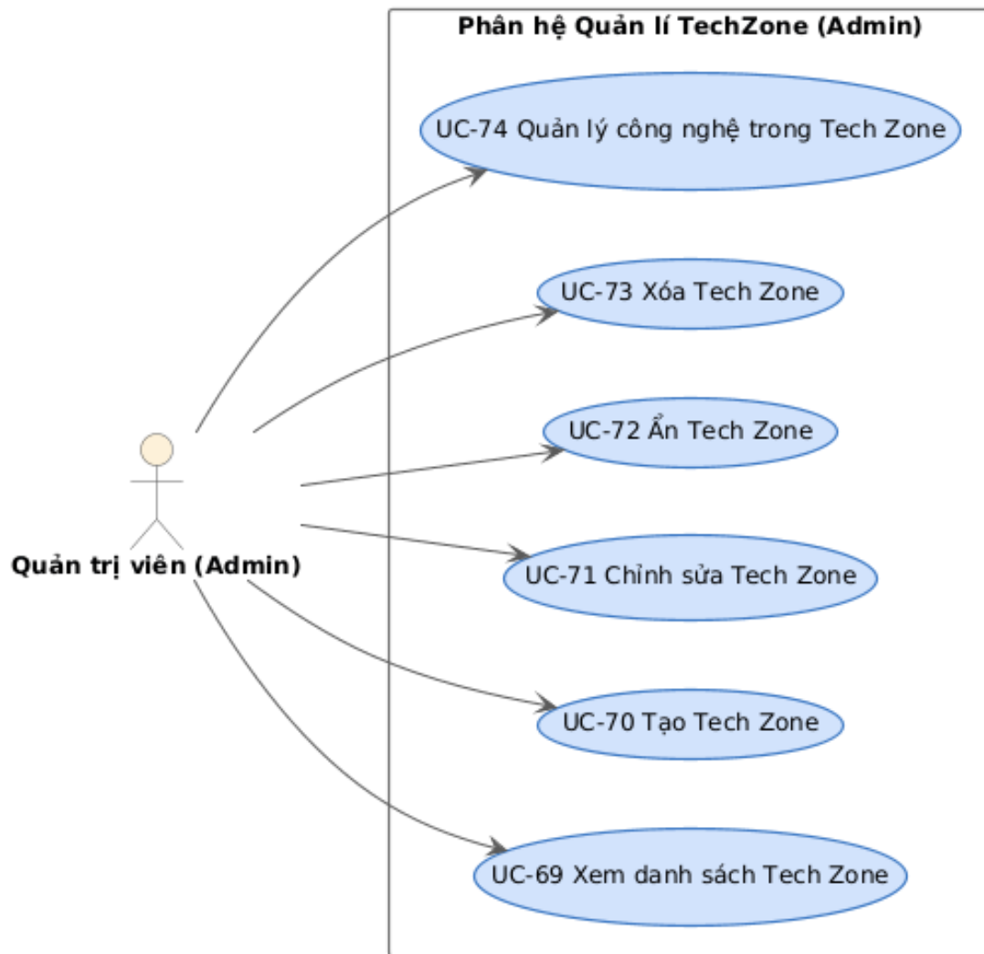
Hình 2.15: Sơ đồ Use Case Nhóm 13 - Quản lý TechZone Admin (UC-69 đến UC-74)
