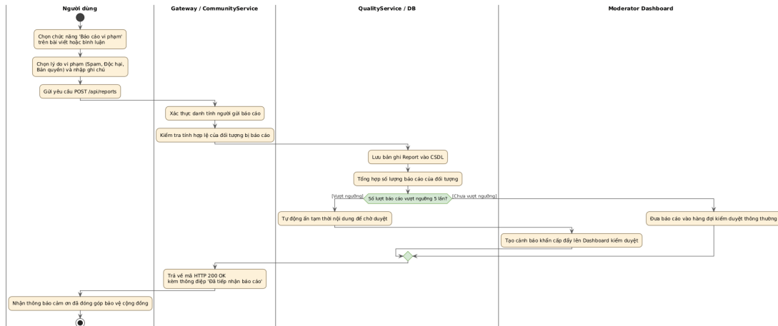
Hình 3.8.a: Biểu đồ Hoạt động (Activity Diagram) Tiến trình Báo cáo vi phạm nội dung
