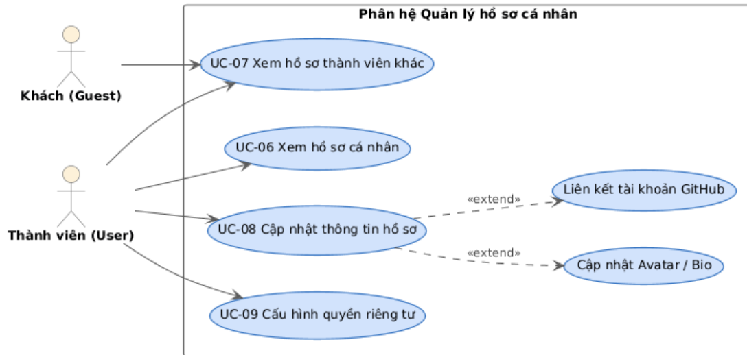
Hình 2.4: Sơ đồ Use Case Nhóm 2 - Quản lý hồ sơ cá nhân (UC-06 đến UC-09)
