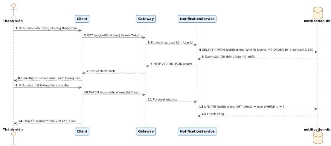
Hình 3.9.b: Biểu đồ Tuần tự (Sequence Diagram) Tiến trình Xem và Quản lý thông báo
