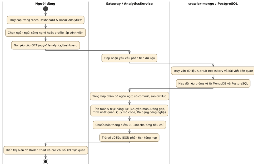
Hình 3.10.a: Biểu đồ Hoạt động (Activity Diagram) Tiến trình Tra cứu Tech Dashboard & Radar Chart
