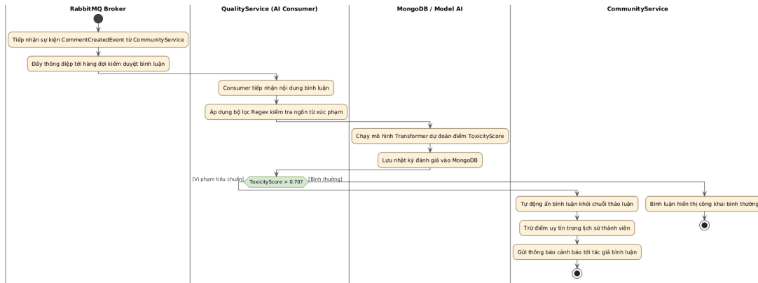
Hình 3.13.a: Biểu đồ Hoạt động (Activity Diagram) Tiến trình AI Kiểm duyệt bình luận vi phạm
