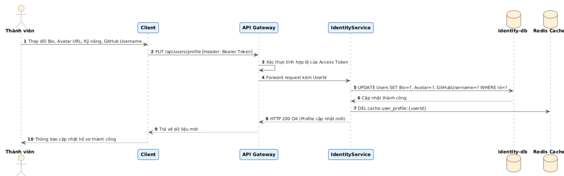
Hình 3.3.b: Biểu đồ Tuần tự (Sequence Diagram) Tiến trình Cập nhật hồ sơ cá nhân
