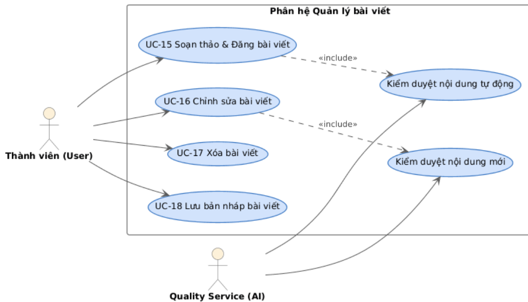
Hình 2.5: Sơ đồ Use Case Nhóm 3 - Quản lý bài viết (UC-15 đến UC-18)
