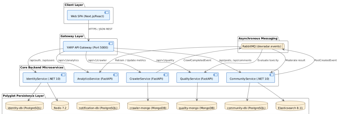
Hình 2.1: Sơ đồ kiến trúc tổng quan hệ thống Microservices DevRadar
