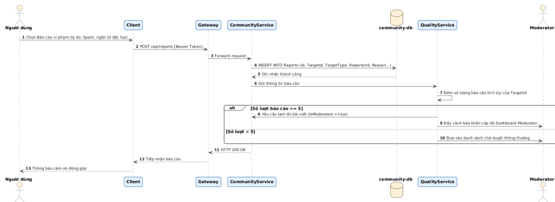
Hình 3.8.b: Biểu đồ Tuần tự (Sequence Diagram) Tiến trình Báo cáo vi phạm nội dung
