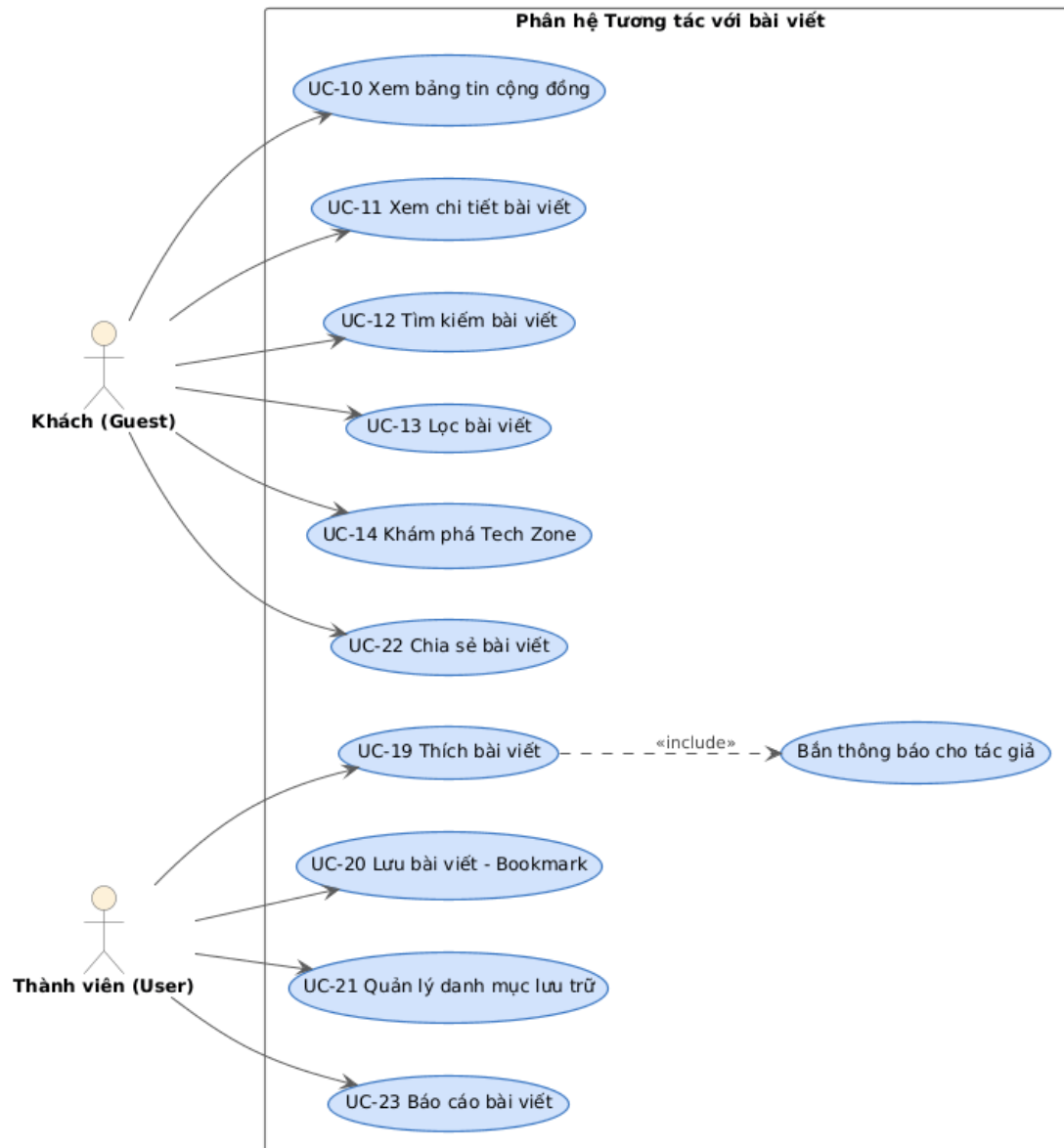
Hình 2.6: Sơ đồ Use Case Nhóm 4 - Tương tác với bài viết (UC-10 đến UC-14, UC-19 đến UC-23)
