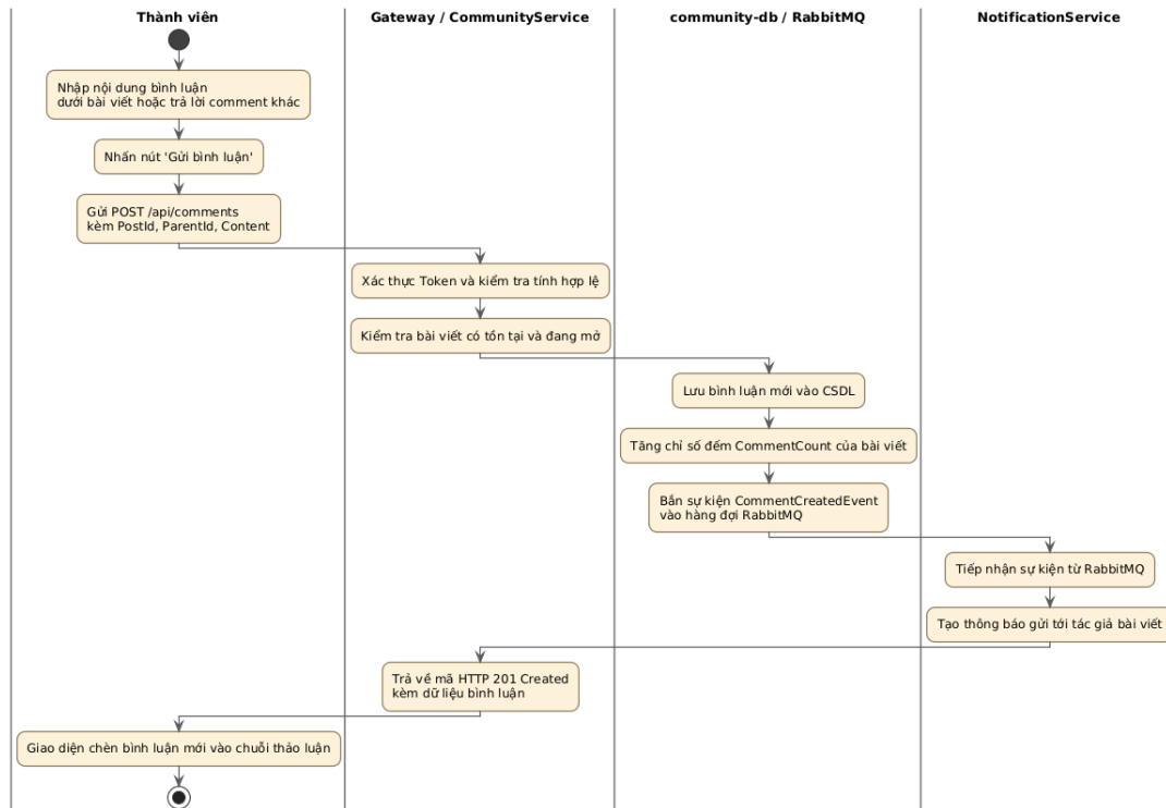
Hình 3.6.a: Biểu đồ Hoạt động (Activity Diagram) Tiến trình Bình luận & Trả lời bình luận
