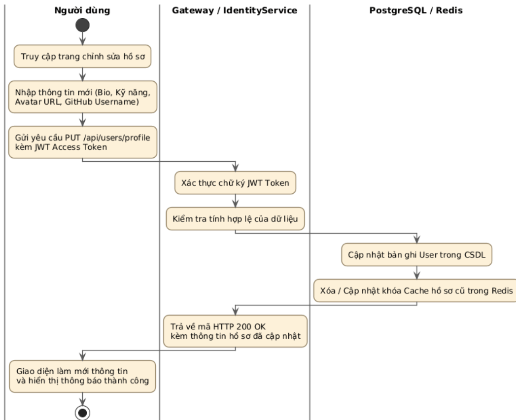
Hình 3.3.a: Biểu đồ Hoạt động (Activity Diagram) Tiến trình Cập nhật hồ sơ cá nhân
