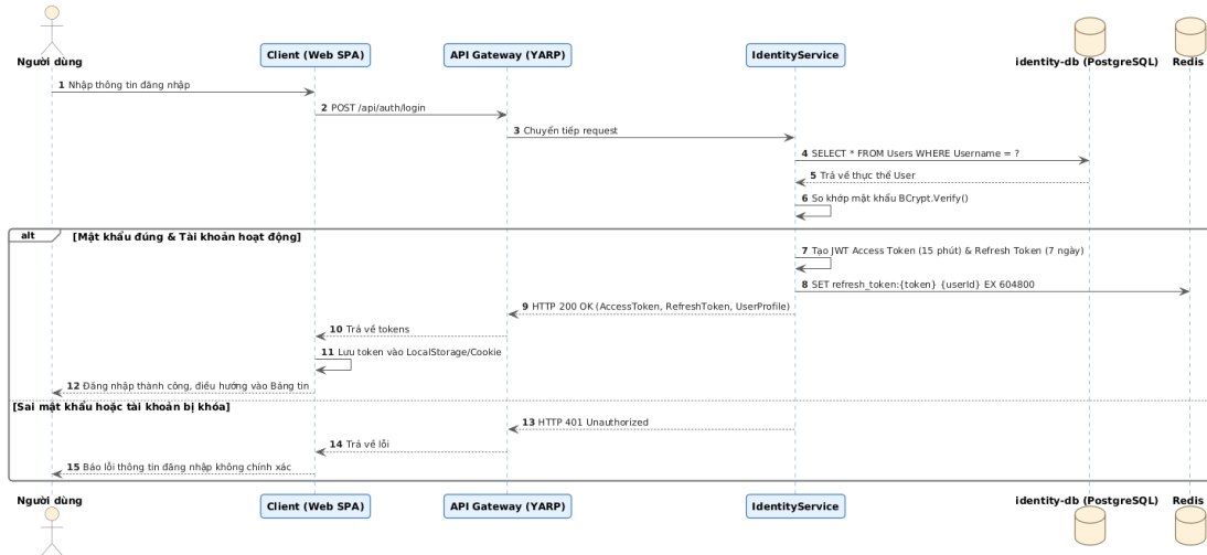
Hình 3.2.b: Biểu đồ Tuần tự (Sequence Diagram) Tiến trình Đăng nhập hệ thống
