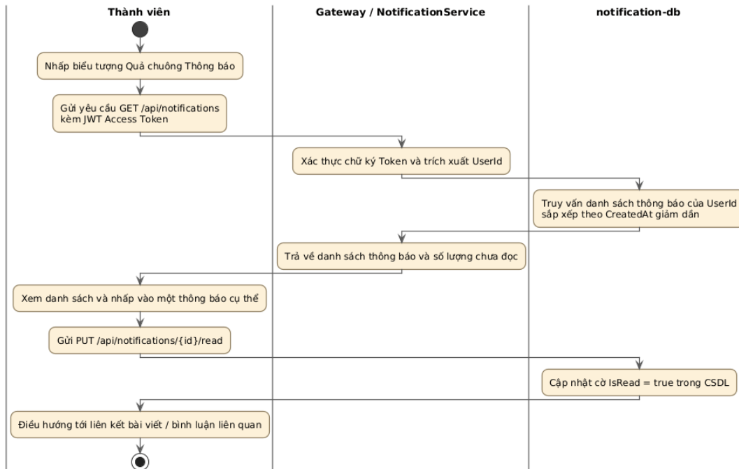
Hình 3.9.a: Biểu đồ Hoạt động (Activity Diagram) Tiến trình Xem và Quản lý thông báo
