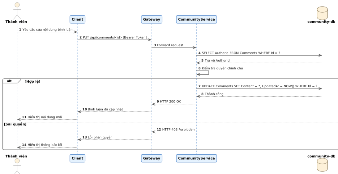
Hình 3.7.b: Biểu đồ Tuần tự (Sequence Diagram) Tiến trình Sửa và Xóa bình luận
