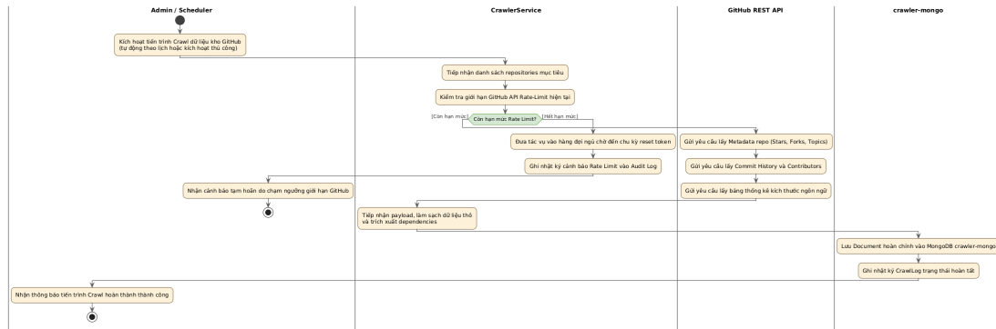
Hình 3.11.a: Biểu đồ Hoạt động (Activity Diagram) Tiến trình Thu thập dữ liệu kho lưu trữ GitHub
