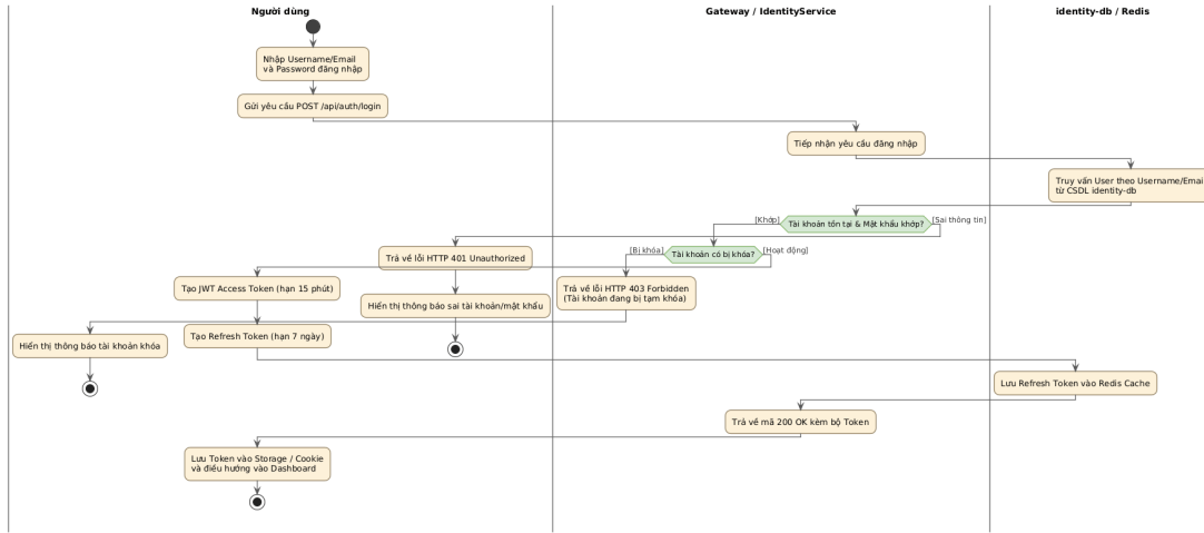
Hình 3.2.a: Biểu đồ Hoạt động (Activity Diagram) Tiến trình Đăng nhập hệ thống
