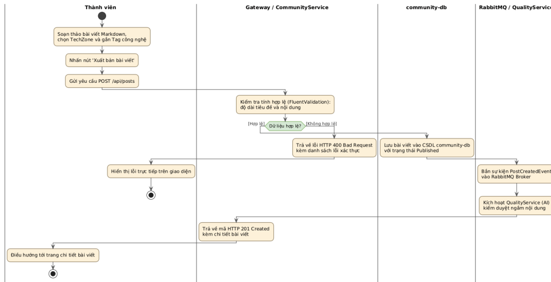
Hình 3.4.a: Biểu đồ Hoạt động (Activity Diagram) Tiến trình Đăng bài viết chia sẻ kỹ thuật
