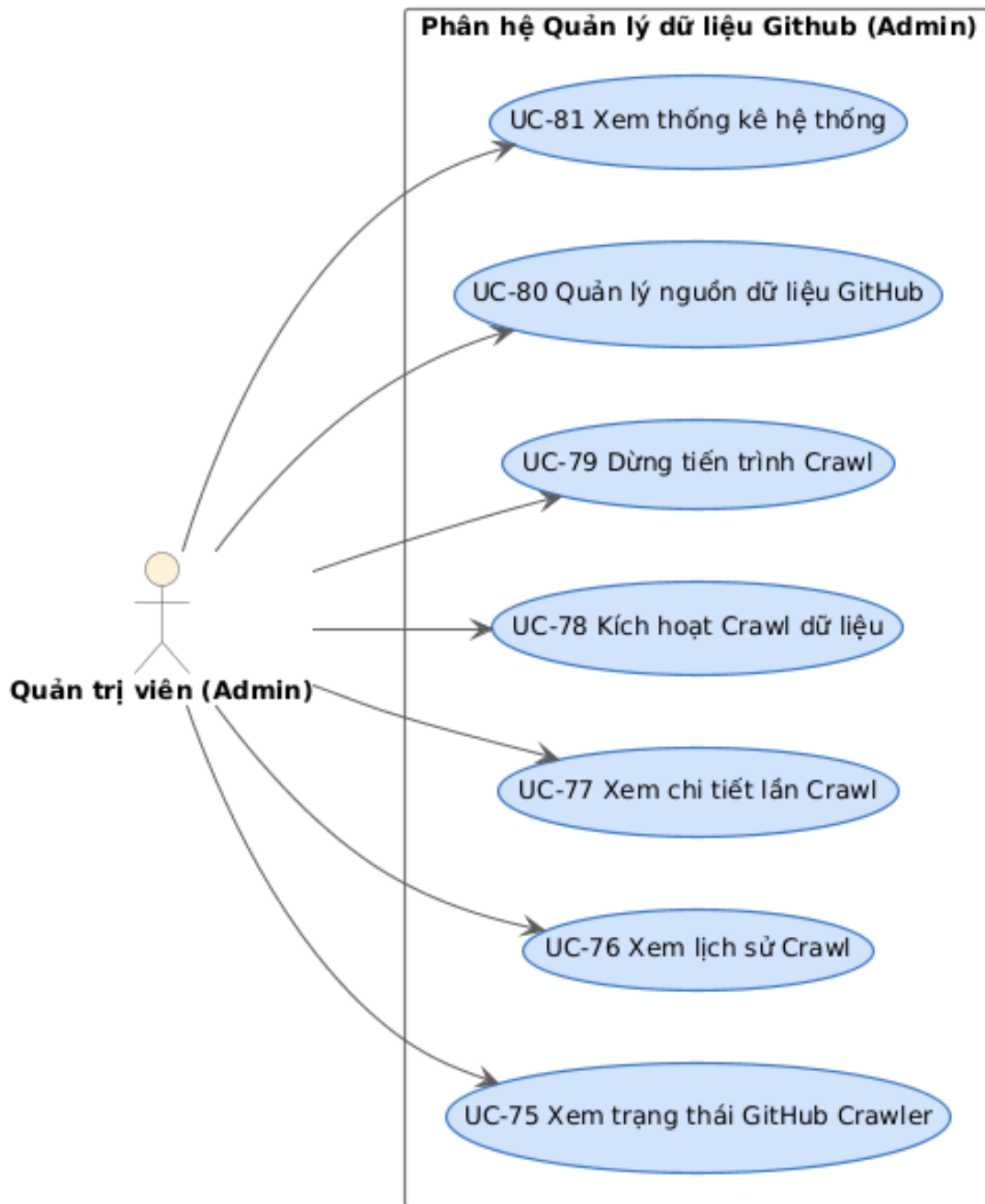
Hình 2.16: Sơ đồ Use Case Nhóm 14 - Quản lý dữ liệu GitHub Admin (UC-75 đến UC-81)
