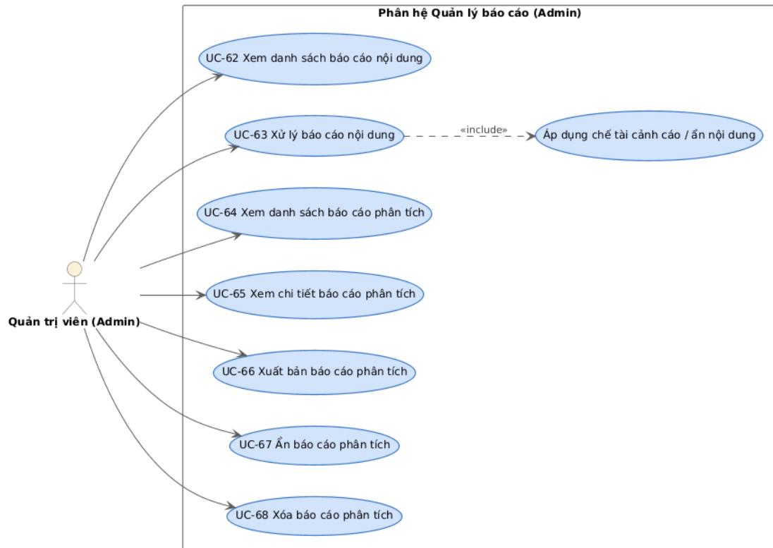
Hình 2.14: Sơ đồ Use Case Nhóm 12 - Quản lý báo cáo Admin (UC-62 đến UC-68)
