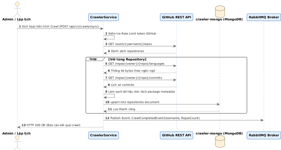
Hình 3.11.b: Biểu đồ Tuần tự (Sequence Diagram) Tiến trình Thu thập dữ liệu kho lưu trữ GitHub
