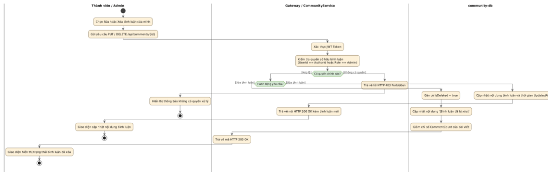
Hình 3.7.a: Biểu đồ Hoạt động (Activity Diagram) Tiến trình Sửa và Xóa bình luận
