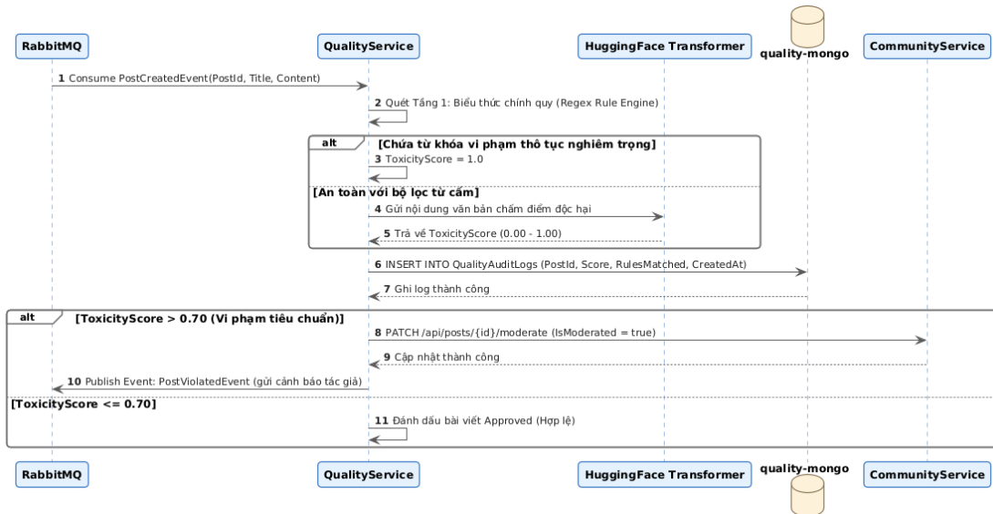
Hình 3.12.b: Biểu đồ Tuần tự (Sequence Diagram) Tiến trình AI Kiểm duyệt bài viết vi phạm
