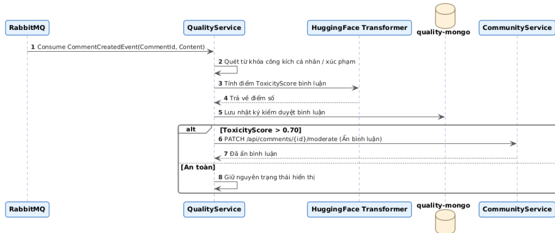
Hình 3.13.b: Biểu đồ Tuần tự (Sequence Diagram) Tiến trình AI Kiểm duyệt bình luận vi phạm
