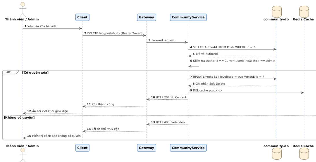
Hình 3.5.b: Biểu đồ Tuần tự (Sequence Diagram) Tiến trình Sửa và Xóa bài viết
