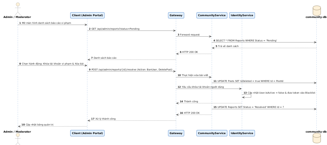
Hình 3.14.b: Biểu đồ Tuần tự (Sequence Diagram) Tiến trình Admin Xử lý báo cáo vi phạm
