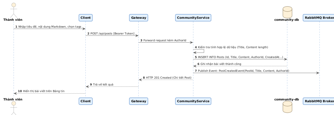
Hình 3.4.b: Biểu đồ Tuần tự (Sequence Diagram) Tiến trình Đăng bài viết chia sẻ kỹ thuật
