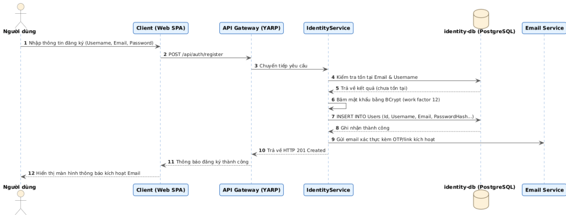
Hình 3.1.b: Biểu đồ Tuần tự (Sequence Diagram) Tiến trình Đăng ký tài khoản
