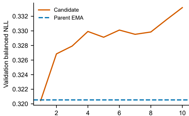
mixup
