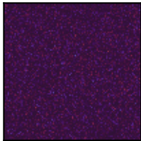
Vision · global
