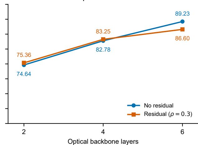
100 epochs · LR 0.003
