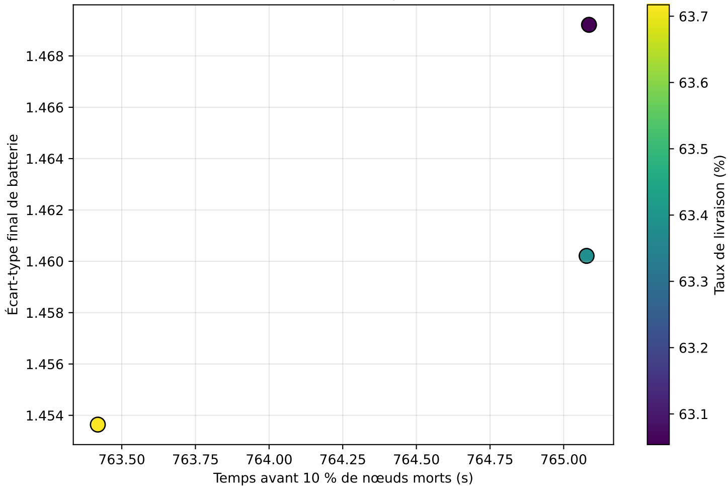
Front de Pareto obtenu par NSGA-II
