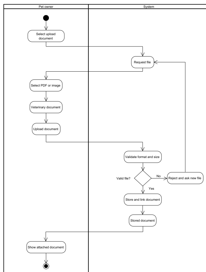
Figura 26: Diagrama de actividades – Cargar documento veterinario y carnet de vacunación (CU-03).
