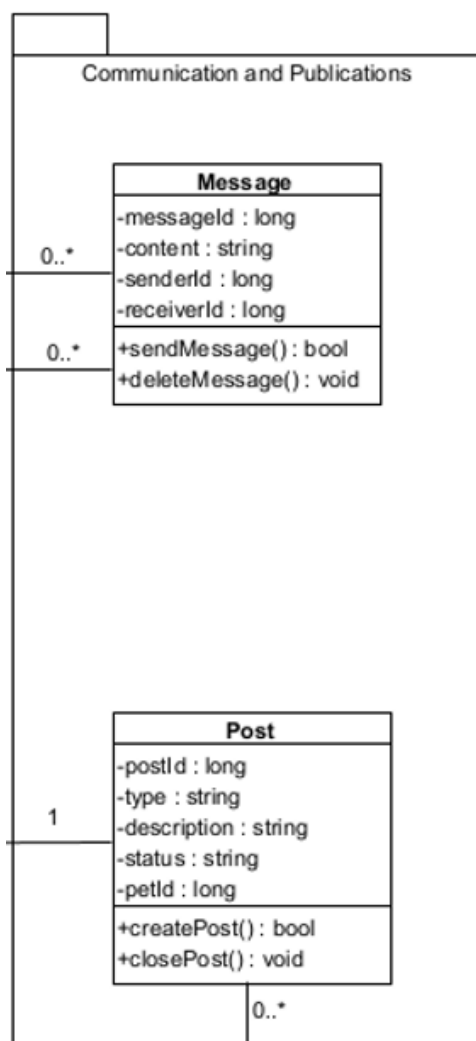
Figura 39: Diagrama de clases – Comunicación y Publicaciones.
