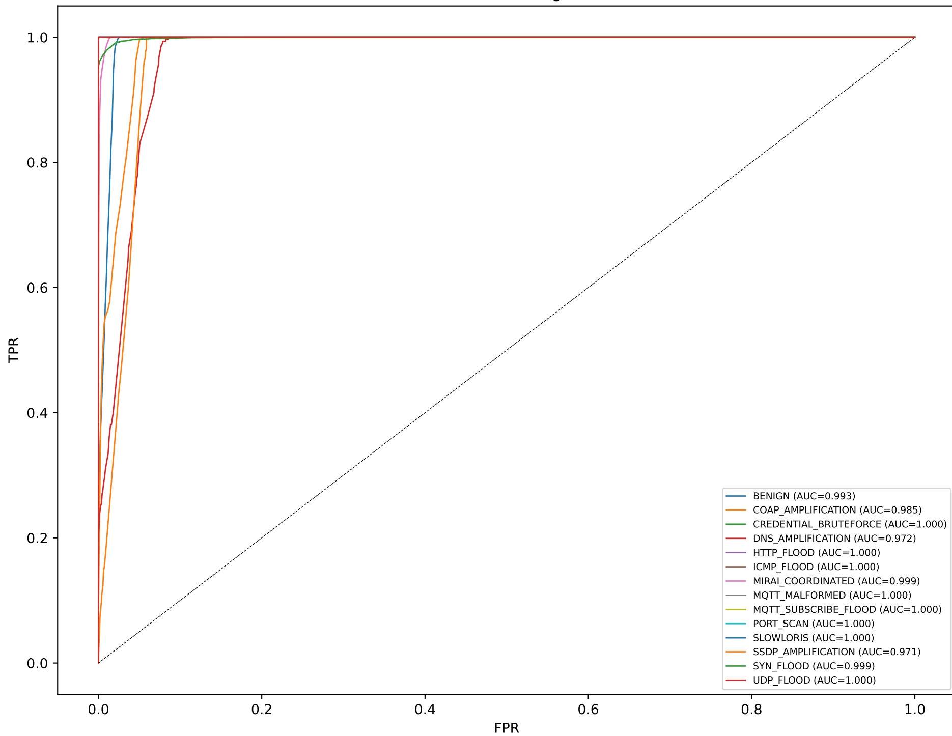
ROC OvR — xgb
