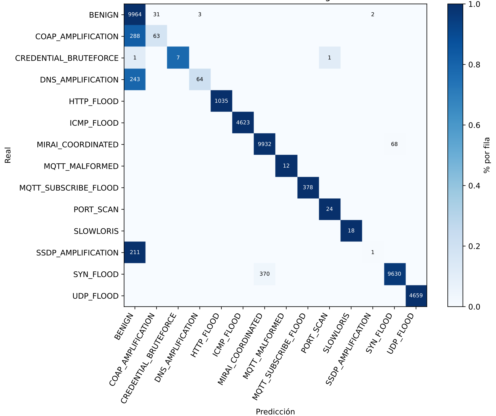
Matriz de confusión — xgb
