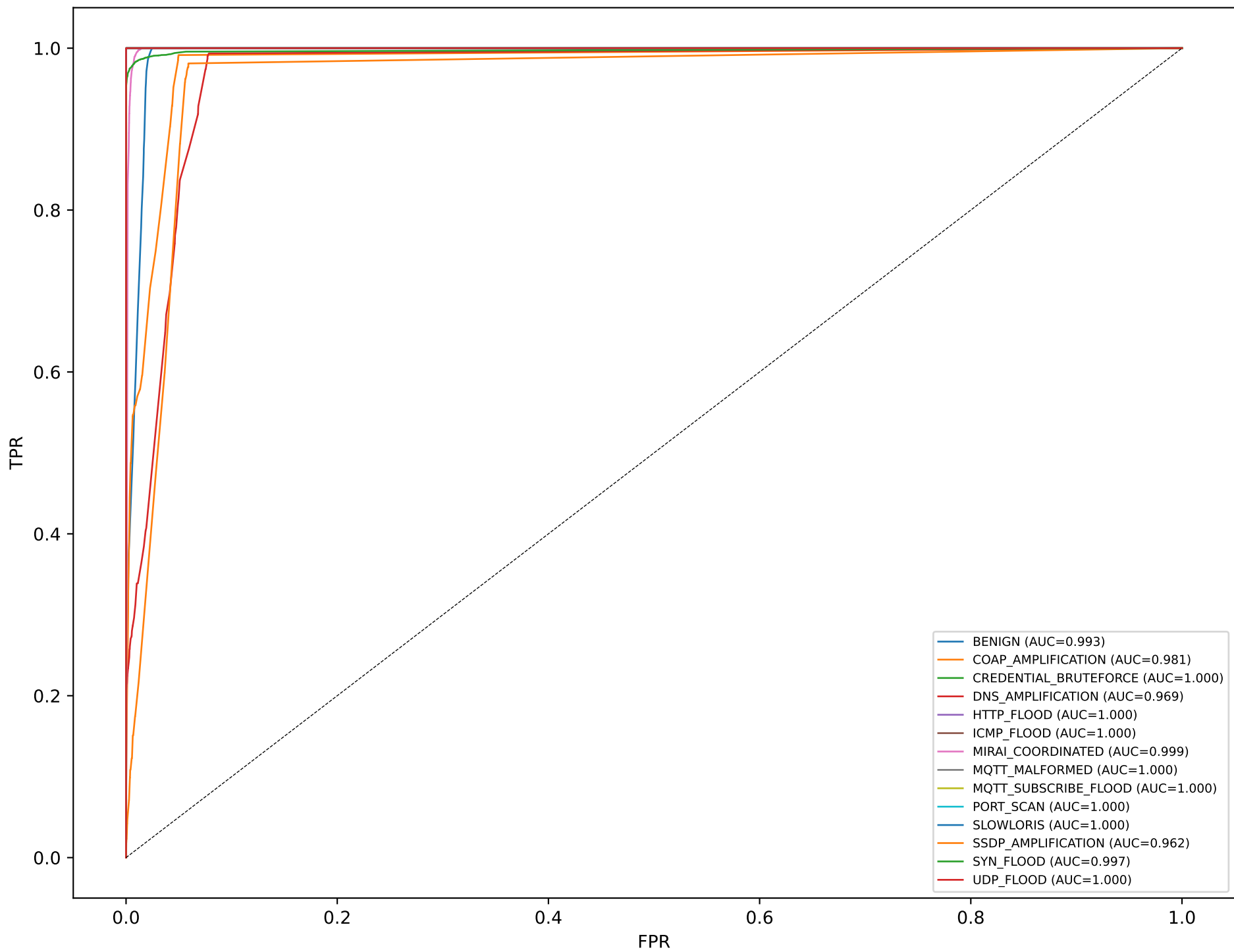
ROC OvR — rf
